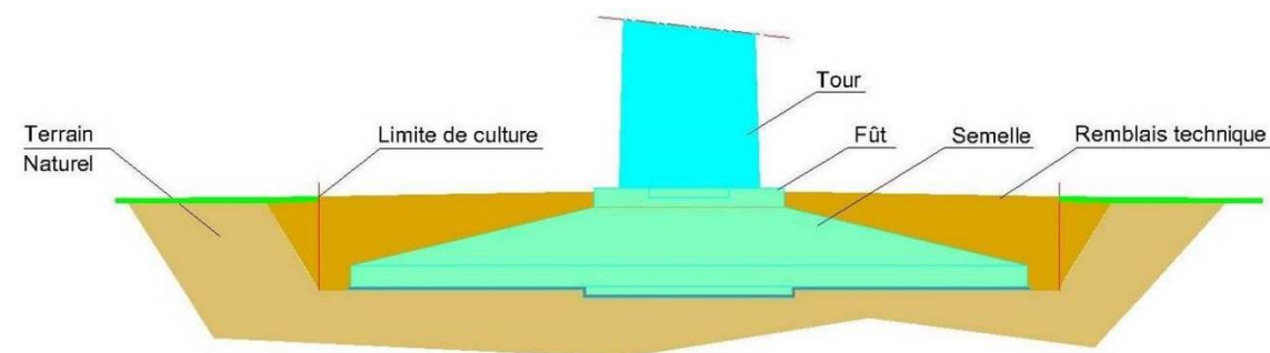
Figure 1 : Schéma type d'une fondation
