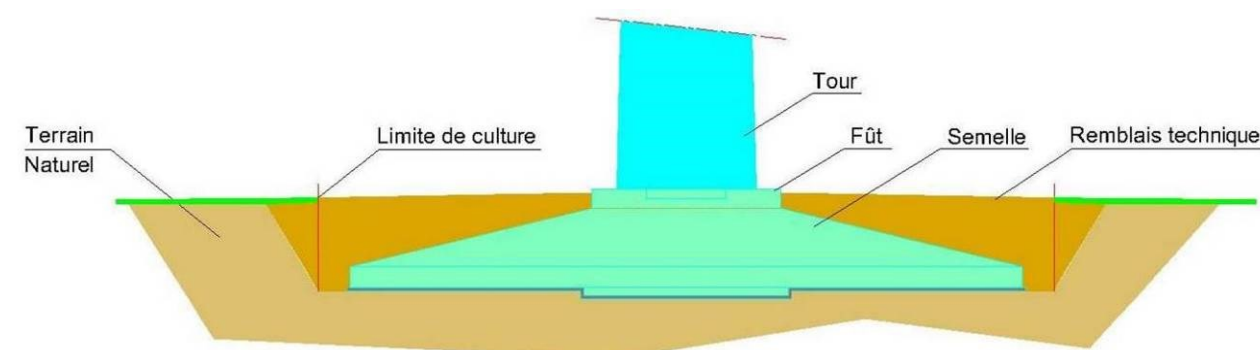
Figure 3 : Schéma type d'une fondation
