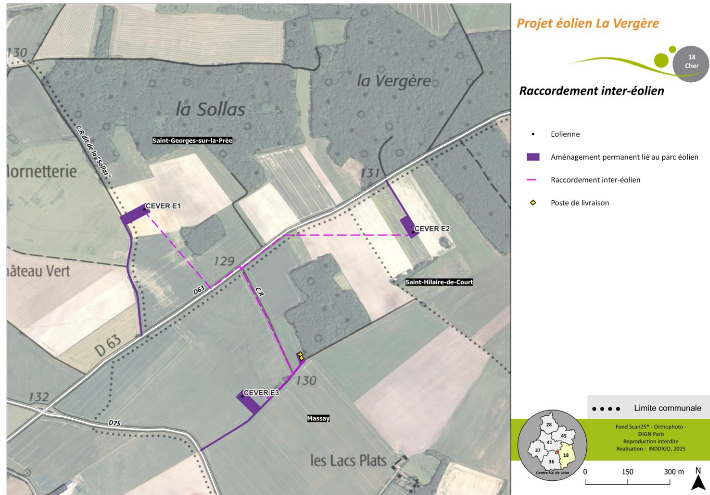
Carte 13 : Plan du raccordement inter-éolien et des postes de livraison
