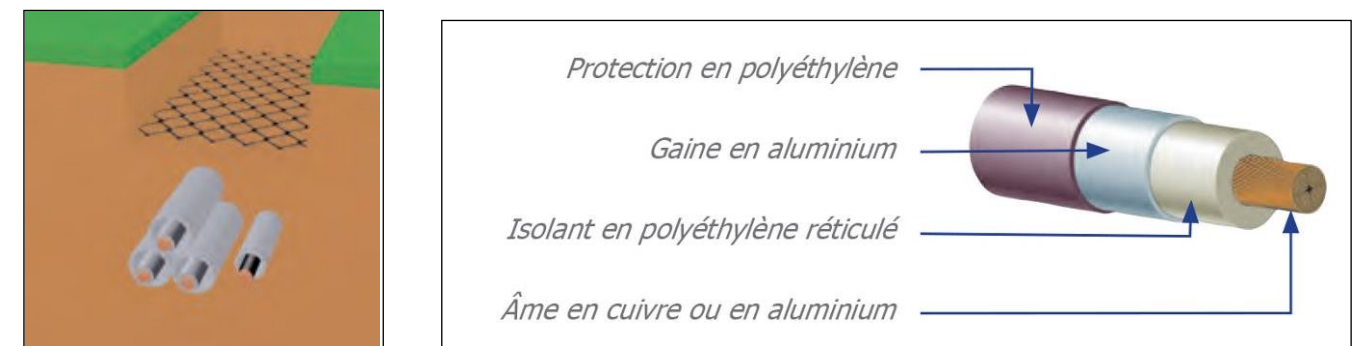
Figure 5 : Principe d'enfouissement et coupe d'un câble de raccordement souterrain (source : RTE)
