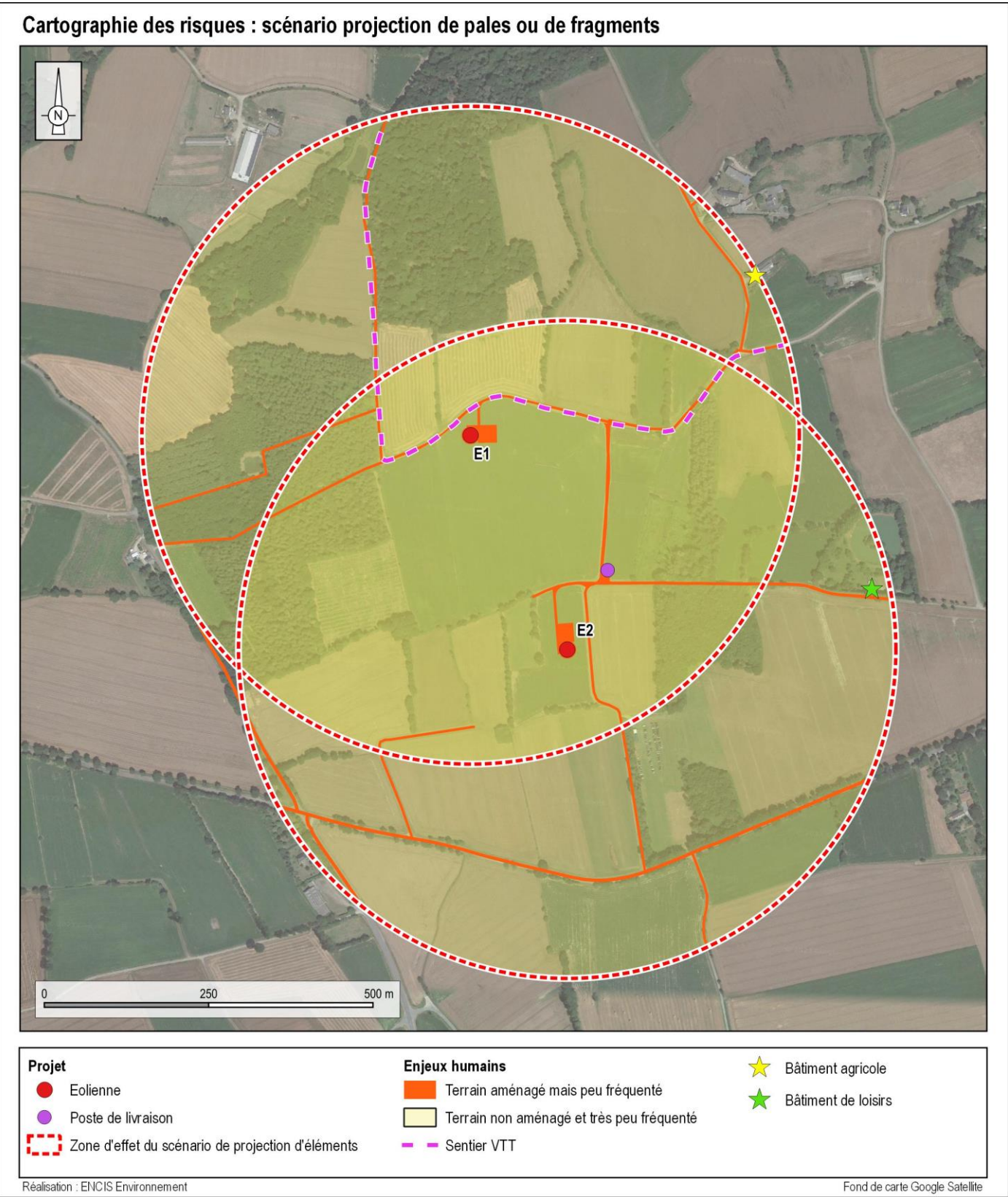
Carte 14 : Cartographie des enjeux identifiés dans les zones d'effet du scénario de projection de pales ou de fragments de pales
