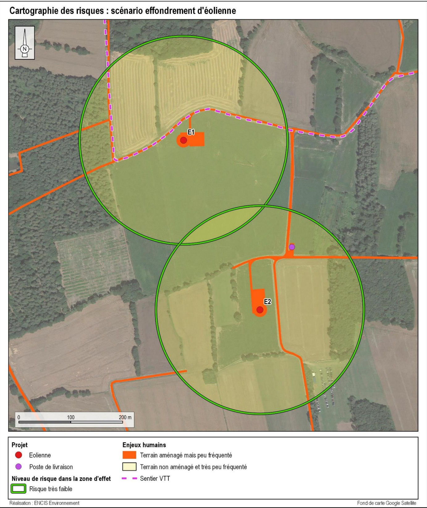
Carte 16 : Cartographie des risques – Scénario d'effondrement de l'éolienne
