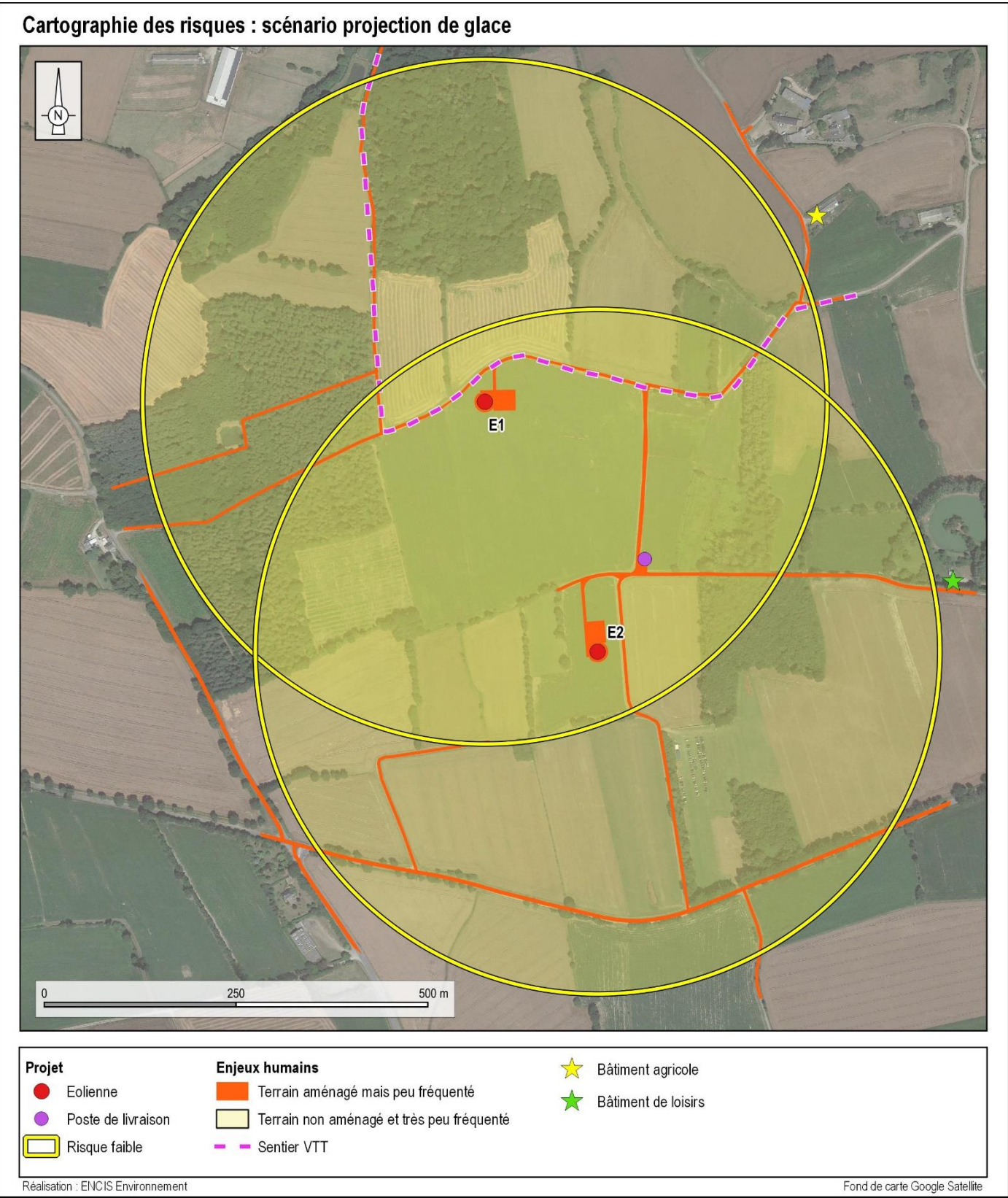
Carte 20 : Cartographie des risques – Scénario de projection de morceaux de glace
