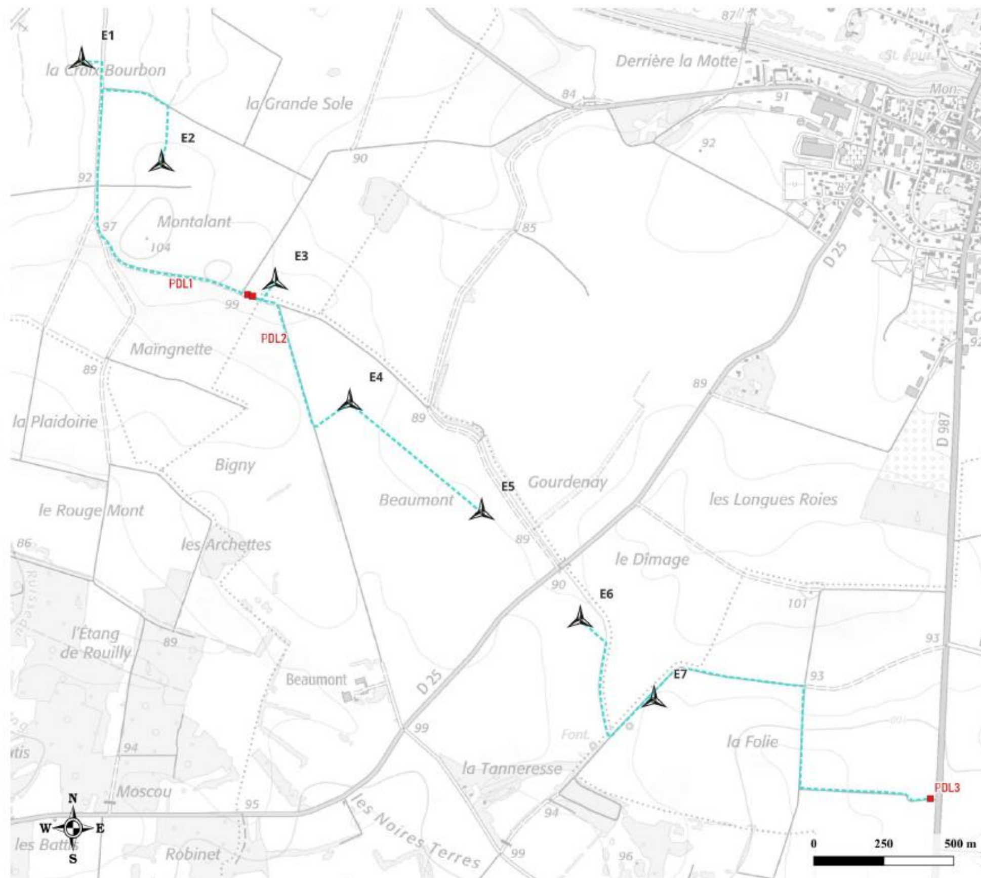
Carte 2 : Plan du raccordement inter-éolien et des postes de livraison
