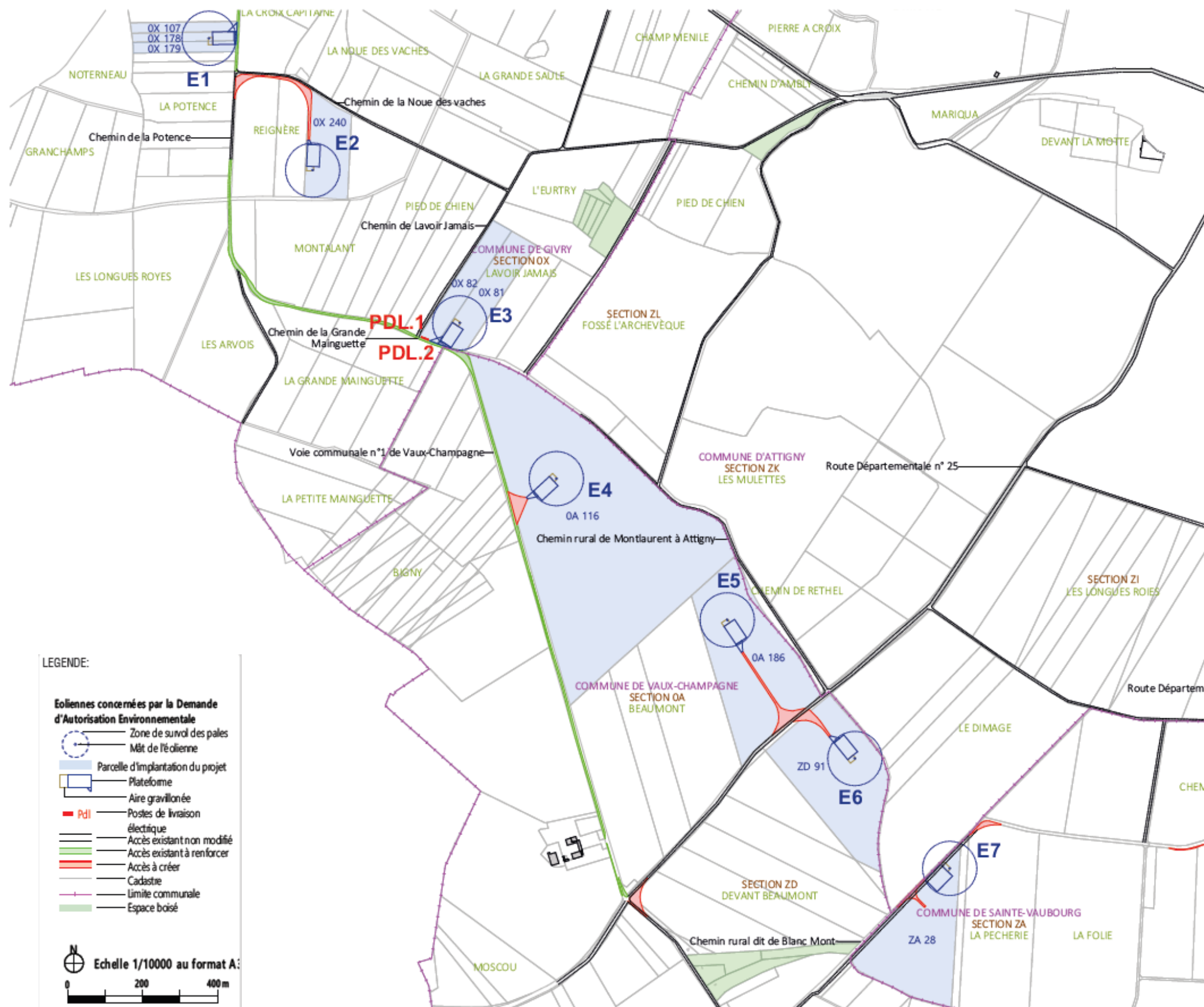
Carte 3 : Vue générale du projet éolien du Pied des Monts à l'échelle 1/10000
