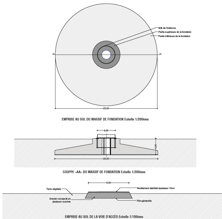
Figure 3 : Principe de dimensionnement d'une fondation d'une éolienne
