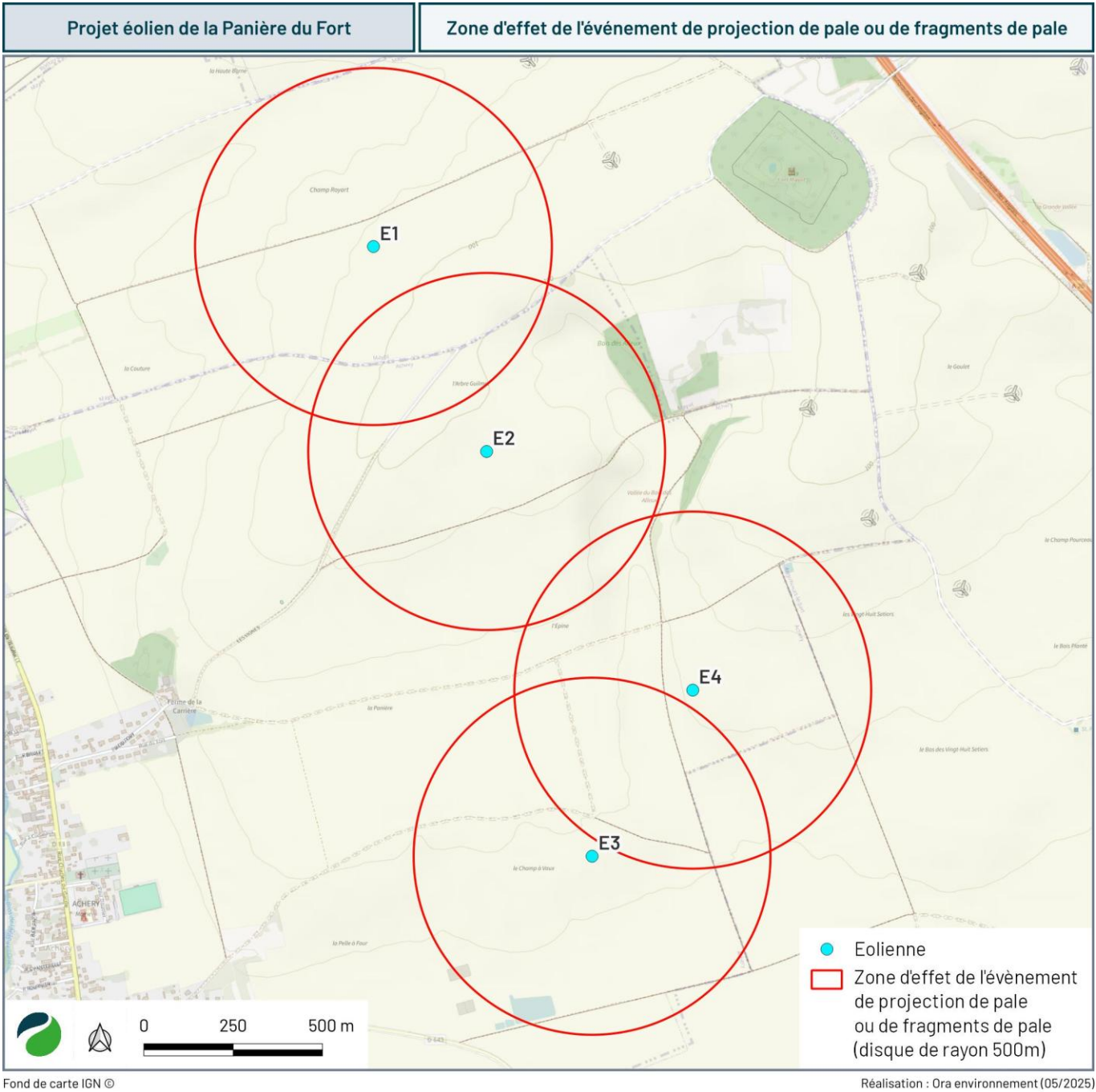
Carte 18 : Zone d'effet de l'événement de projection de pale ou de fragments de pale
