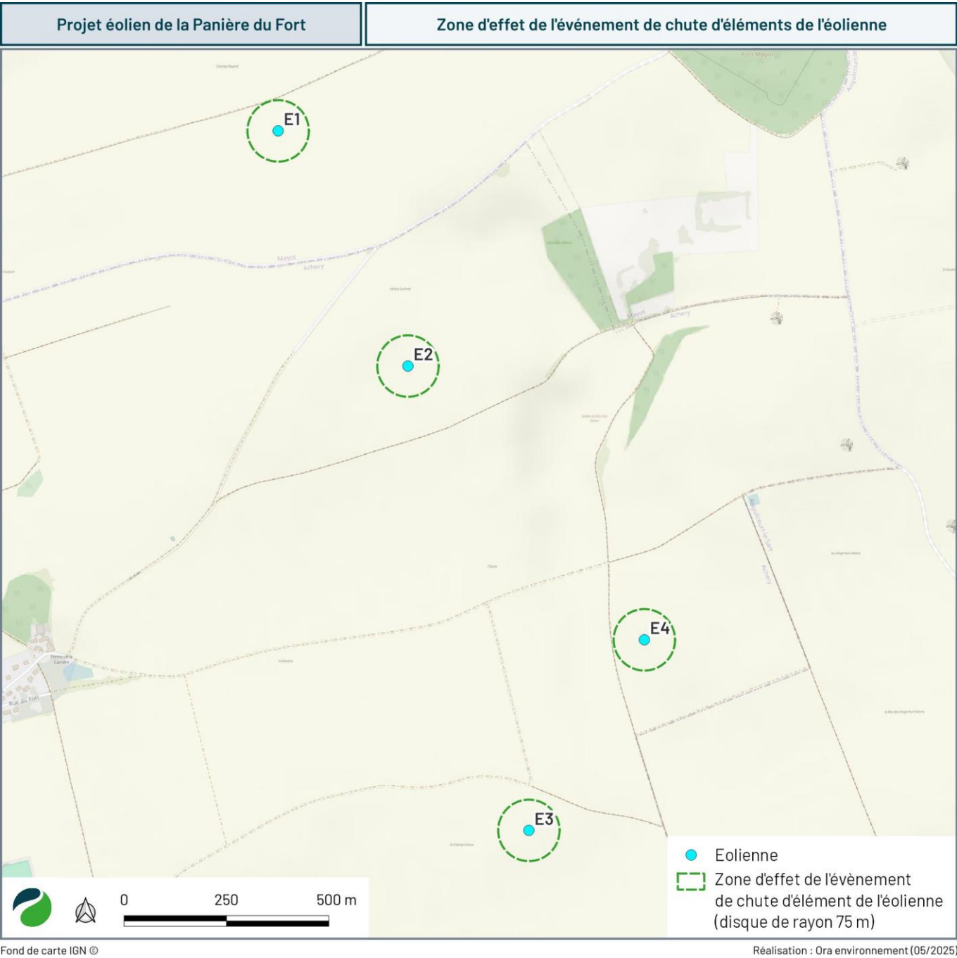
Carte 17 : Zone d'effet de l'événement de chute d'éléments de l'éolienne
