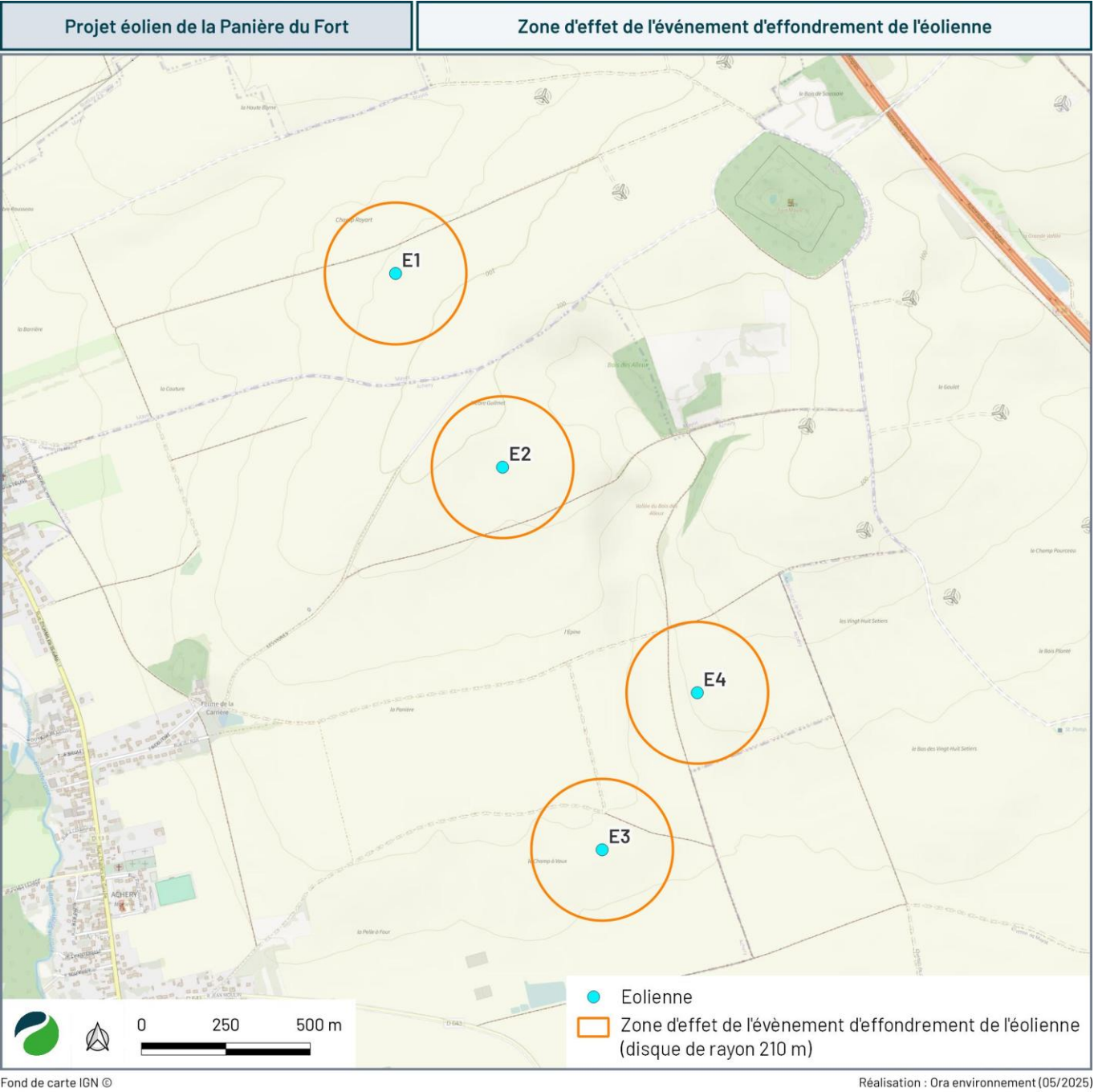
Carte 15 : Zone d'effet de l'évènement d'effondrement de l'éolienne
