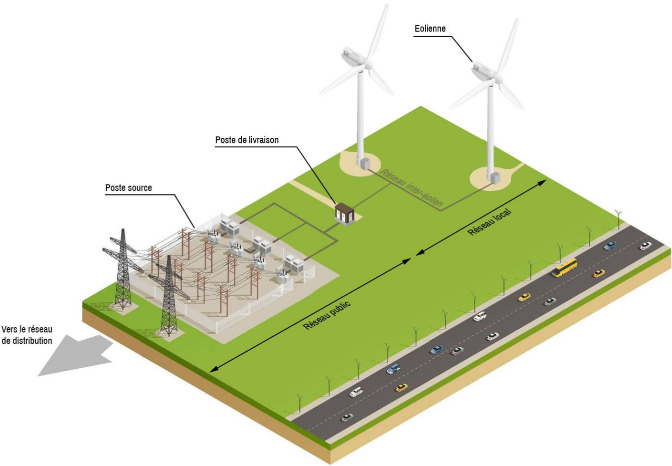
Figure 6 : Raccordement électrique des installations avec l'option HTA (Source : Ora environnement)
