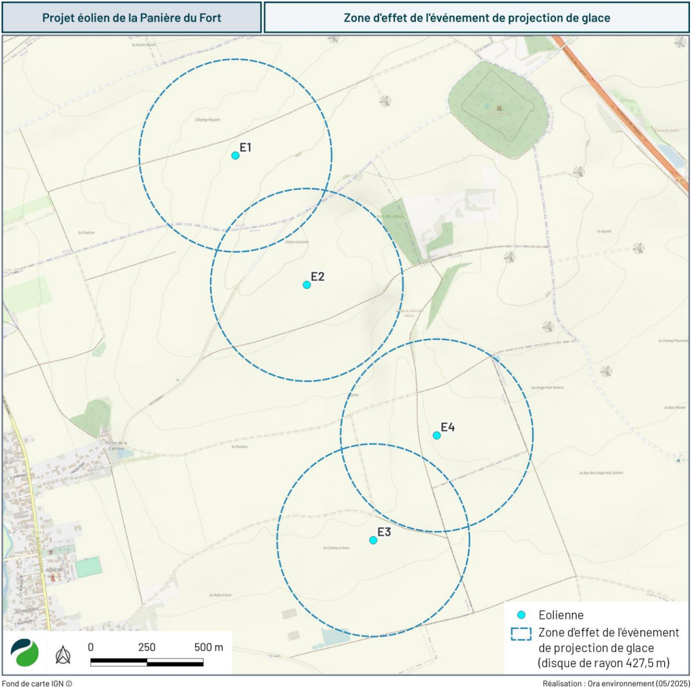
Carte 19 : Zone d'effet de l'événement de projection de glace
