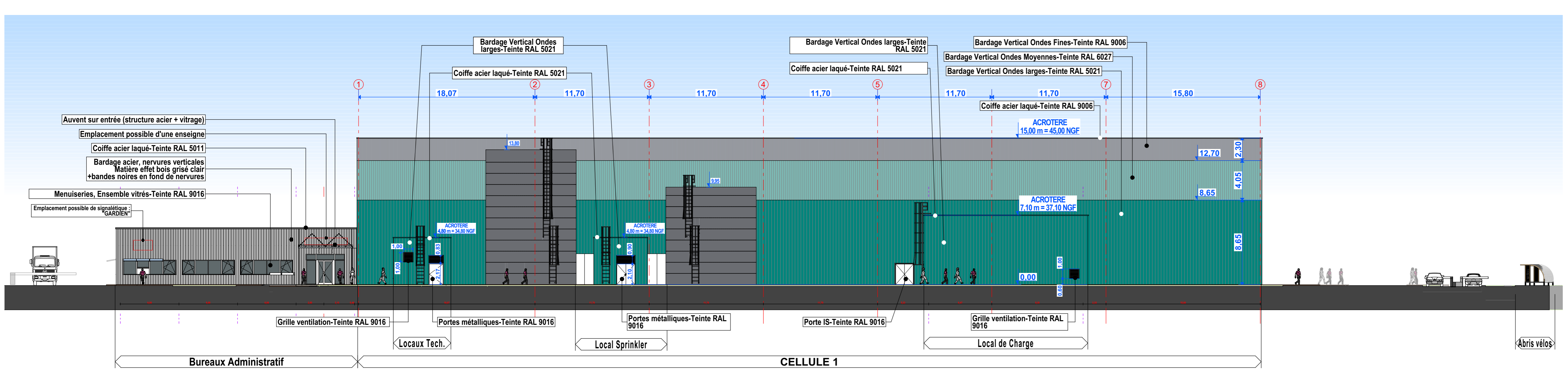
ELEVATION NORD - Ech 1/200
