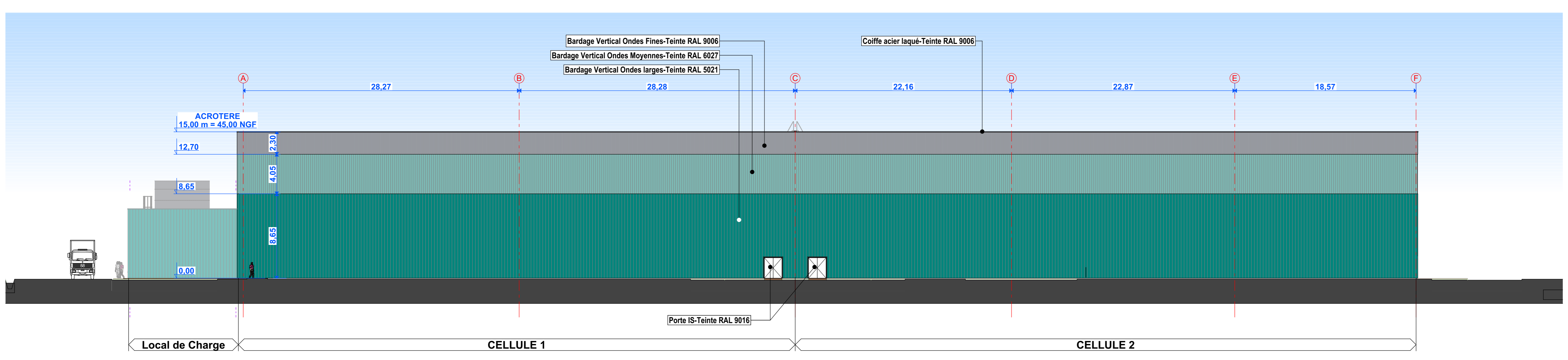
ELEVATION OUEST - Ech 1/200
