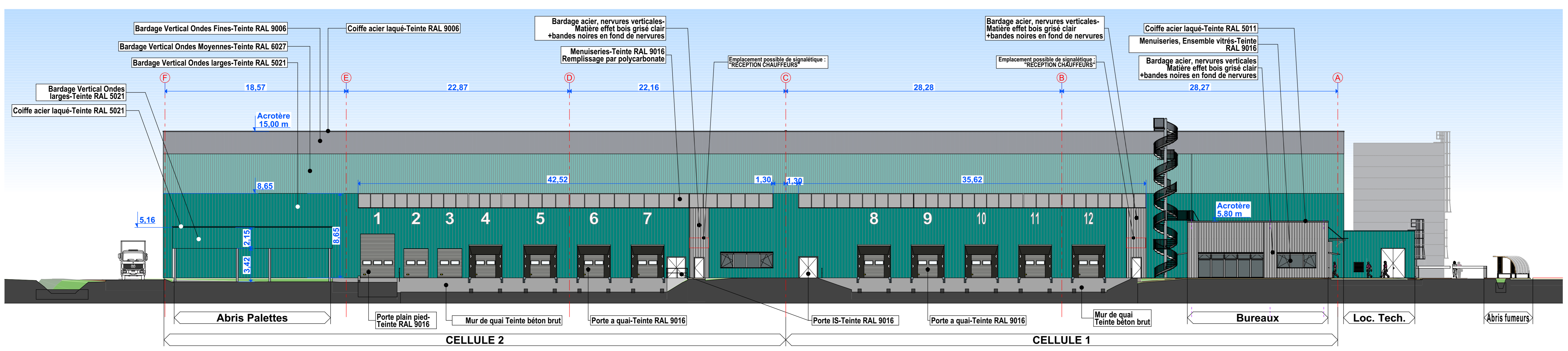
ELEVATION EST - Ech 1/200
