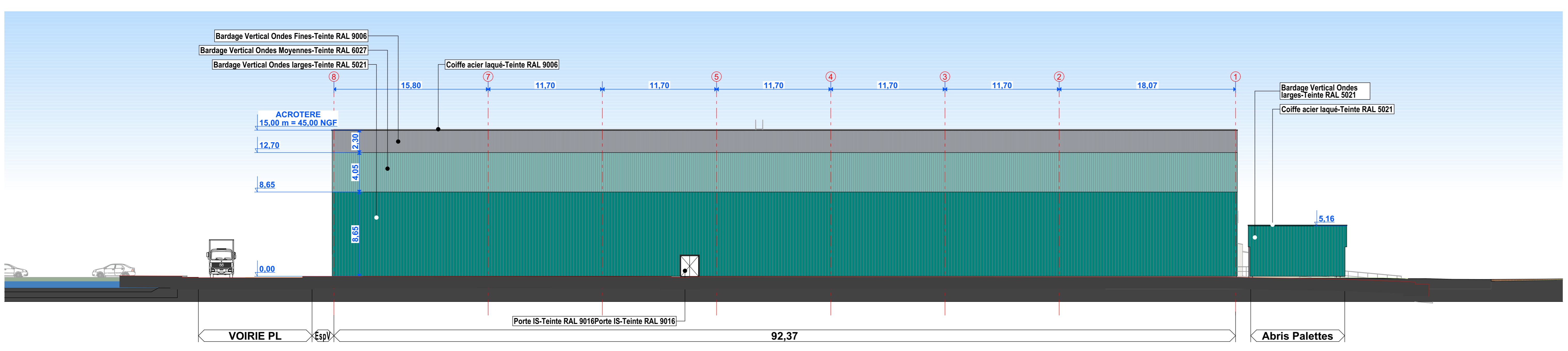
ELEVATION SUD - Ech 1/200
