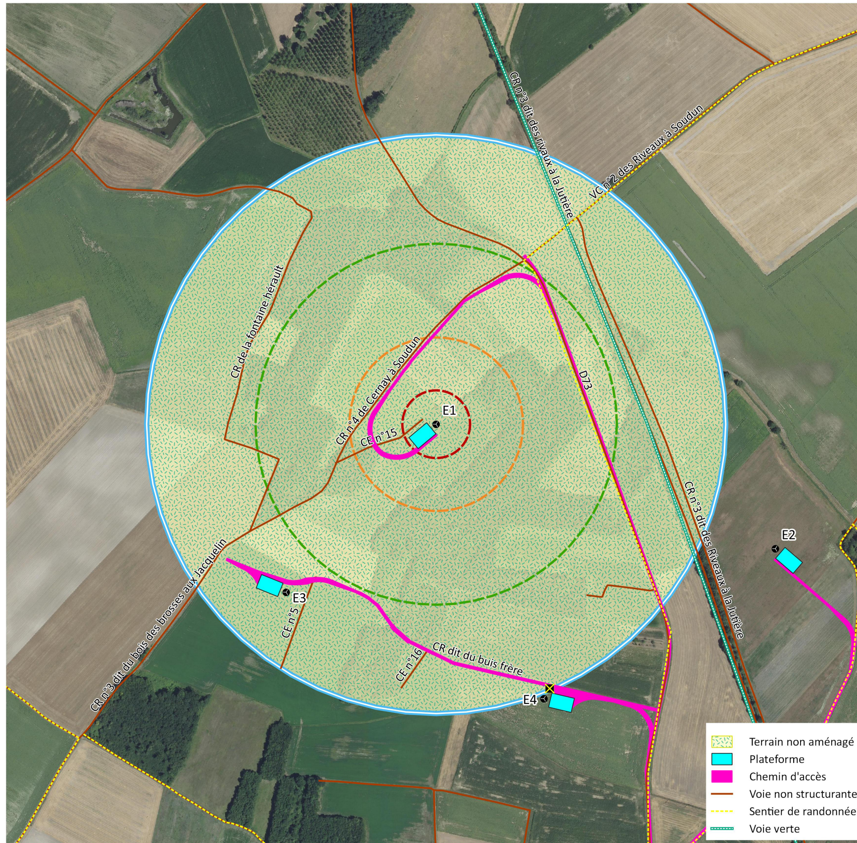
Carte 15 : Synthèse des risques pour l'éolienne E1
