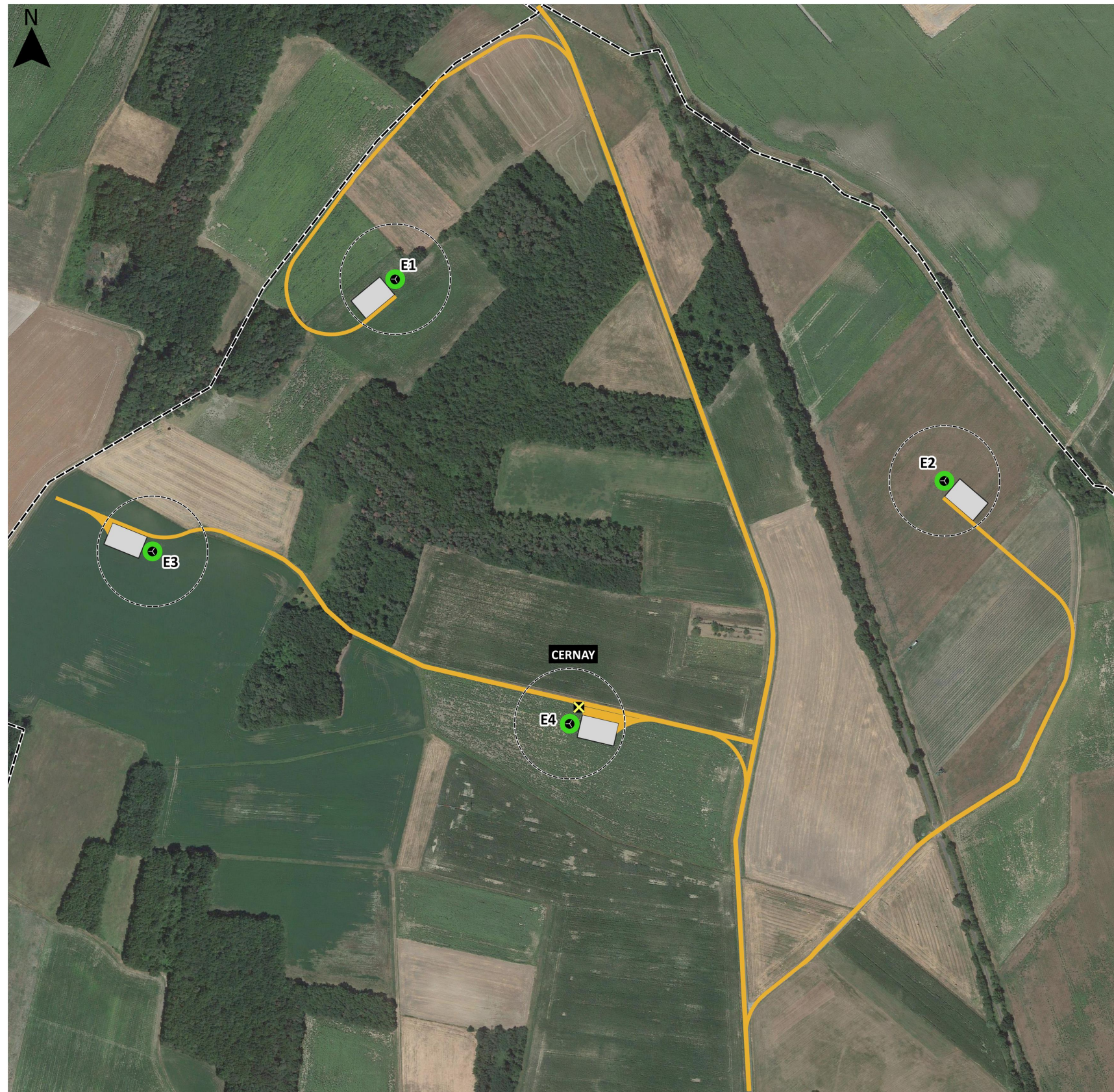
Carte 11 : Le projet en phase d'exploitation
