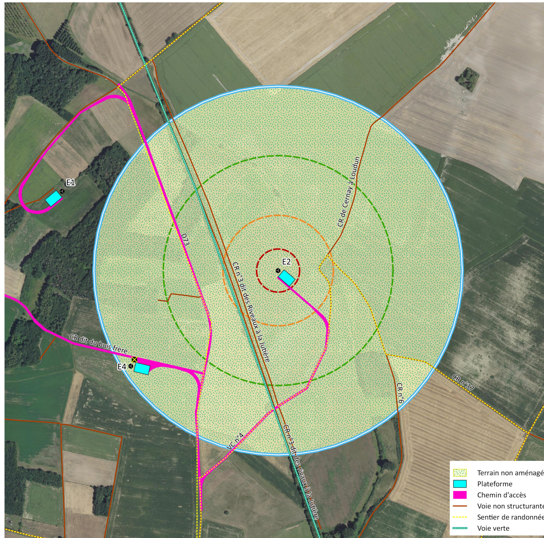
Carte 16 : Synthèse des risques pour l'éolienne E2
