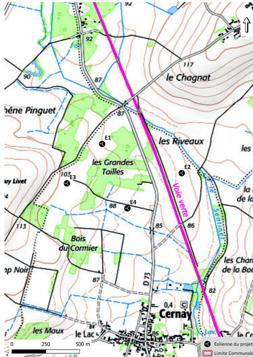
Carte 1 : Plan de situation du projet de parc éolien de Cernay
