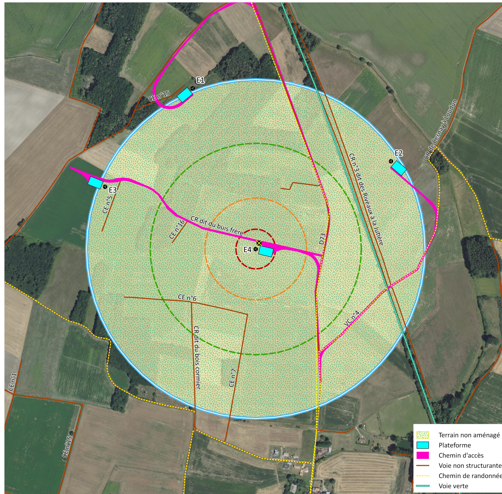
Carte 18 : Synthèse des risques pour l'éolienne E4
