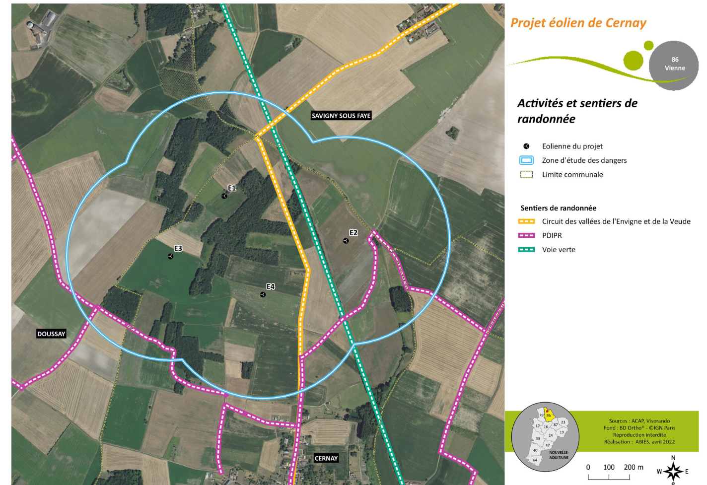
Carte 4 : Activités sur l'aire d'étude de dangers
