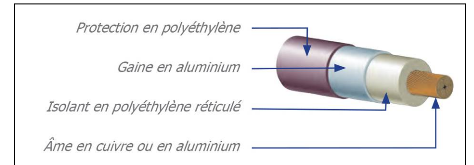
Figure 6 : Principe d'enfouissement et coupe d'un câble de raccordement souterrain (source : RTE)
