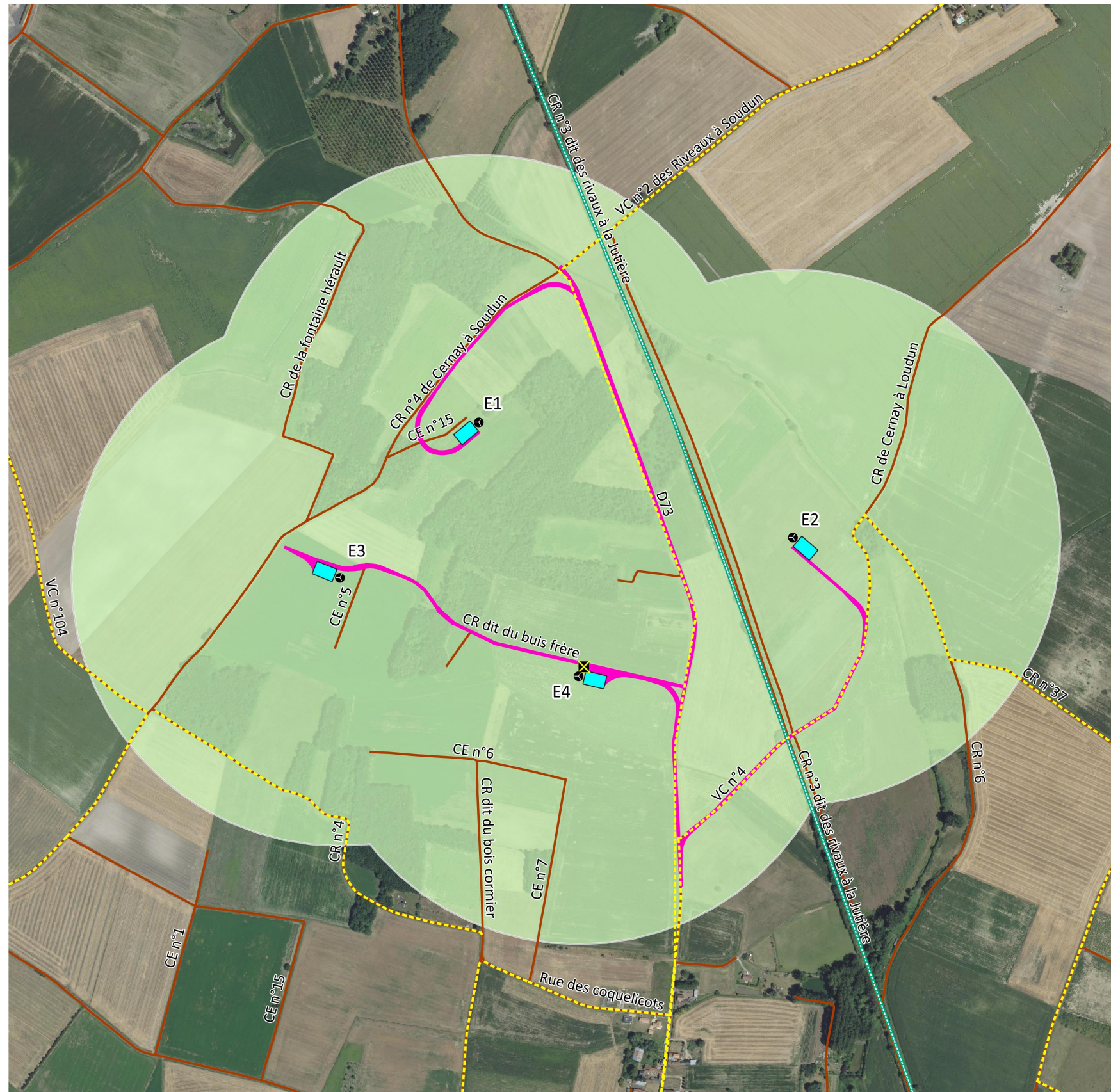
Carte 6 : Cartographie de synthèse des enjeux pour le projet éolien de Cernay
