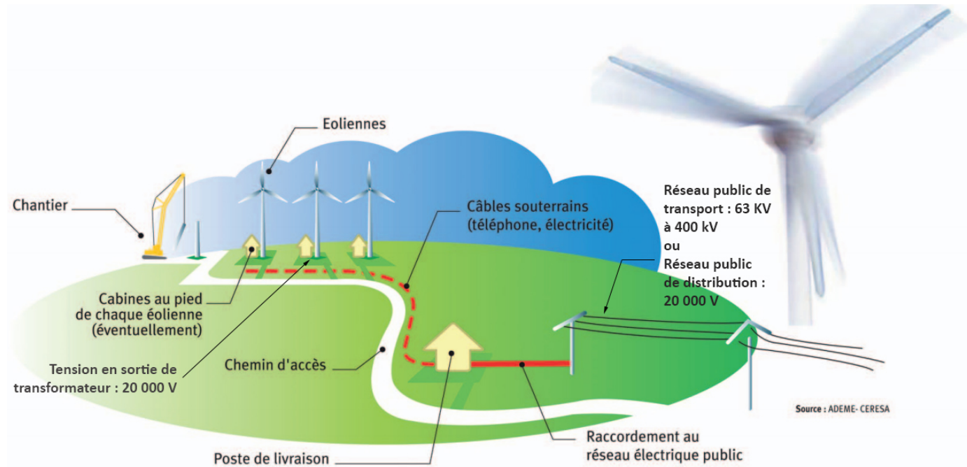
Figure 5 : Schéma de principe du raccordement électrique des installations. (Source: ADEME et CERESA)
