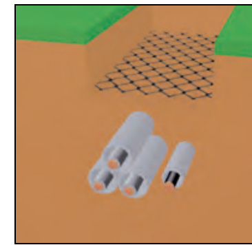
Figure 6 : Principe d'enfouissement et coupe d'un câble de raccordement souterrain (source : RTE)
