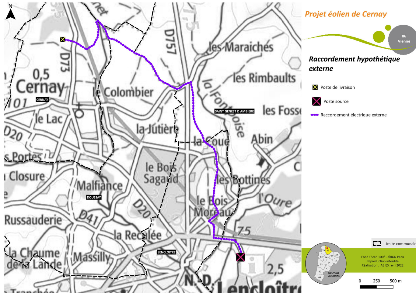
Carte 13 : Hypothèse de raccordement électrique externe envisagée en avril 2022
