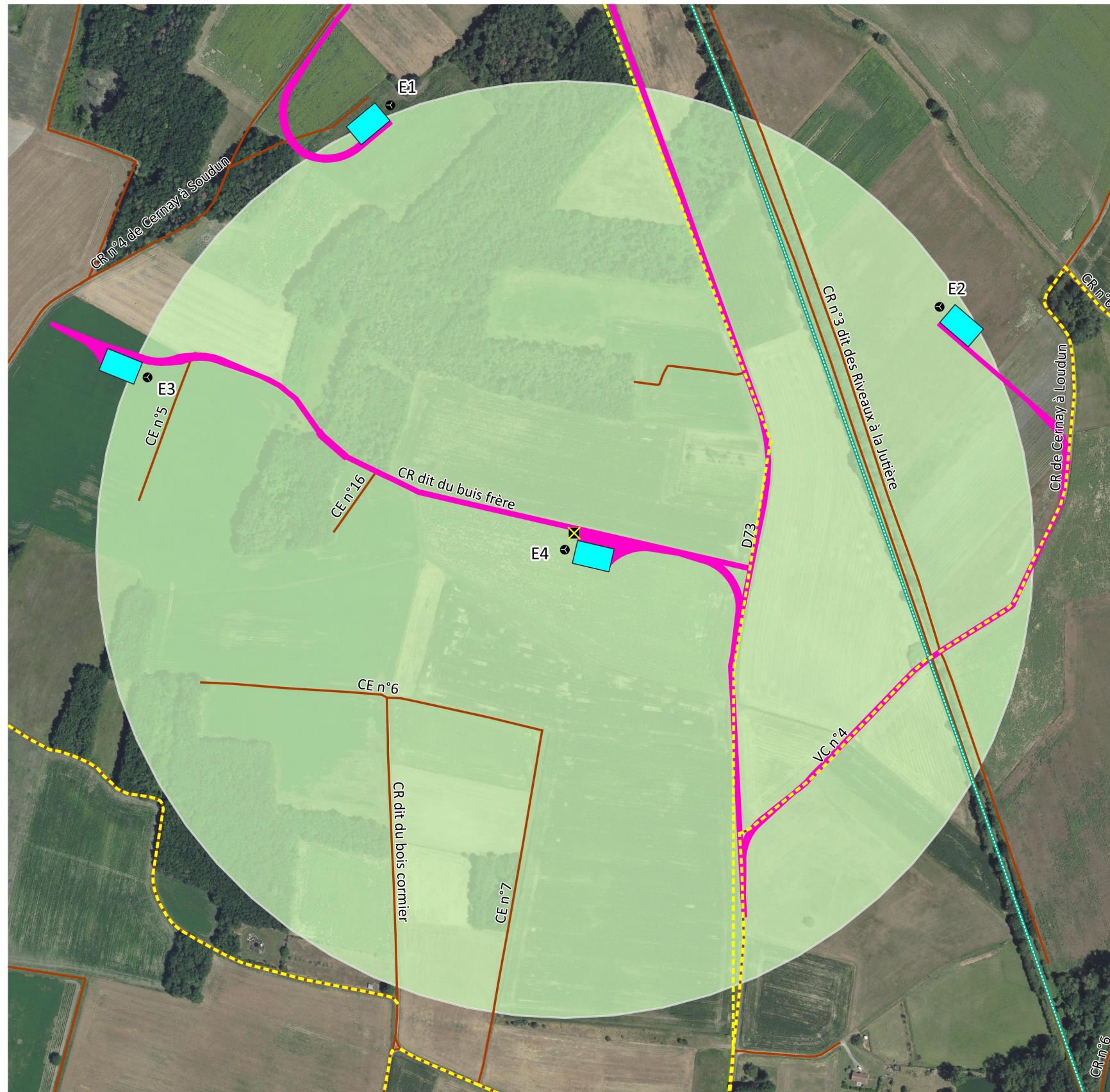
Carte 10 : Cartographie de synthèse des enjeux au droit de l'aire d'étude des dangers d'E4
