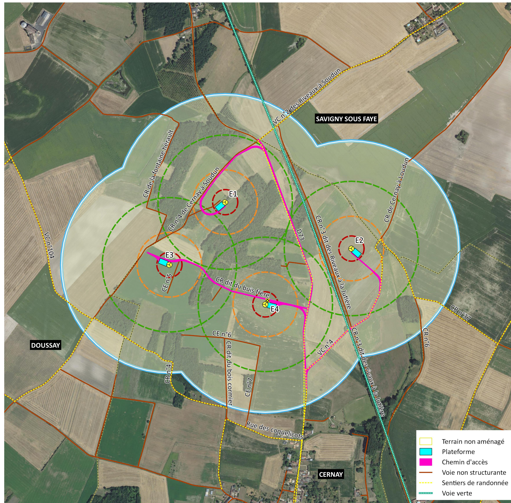
Carte 14 : Synthèse des risques pour les éoliennes de Cernay
