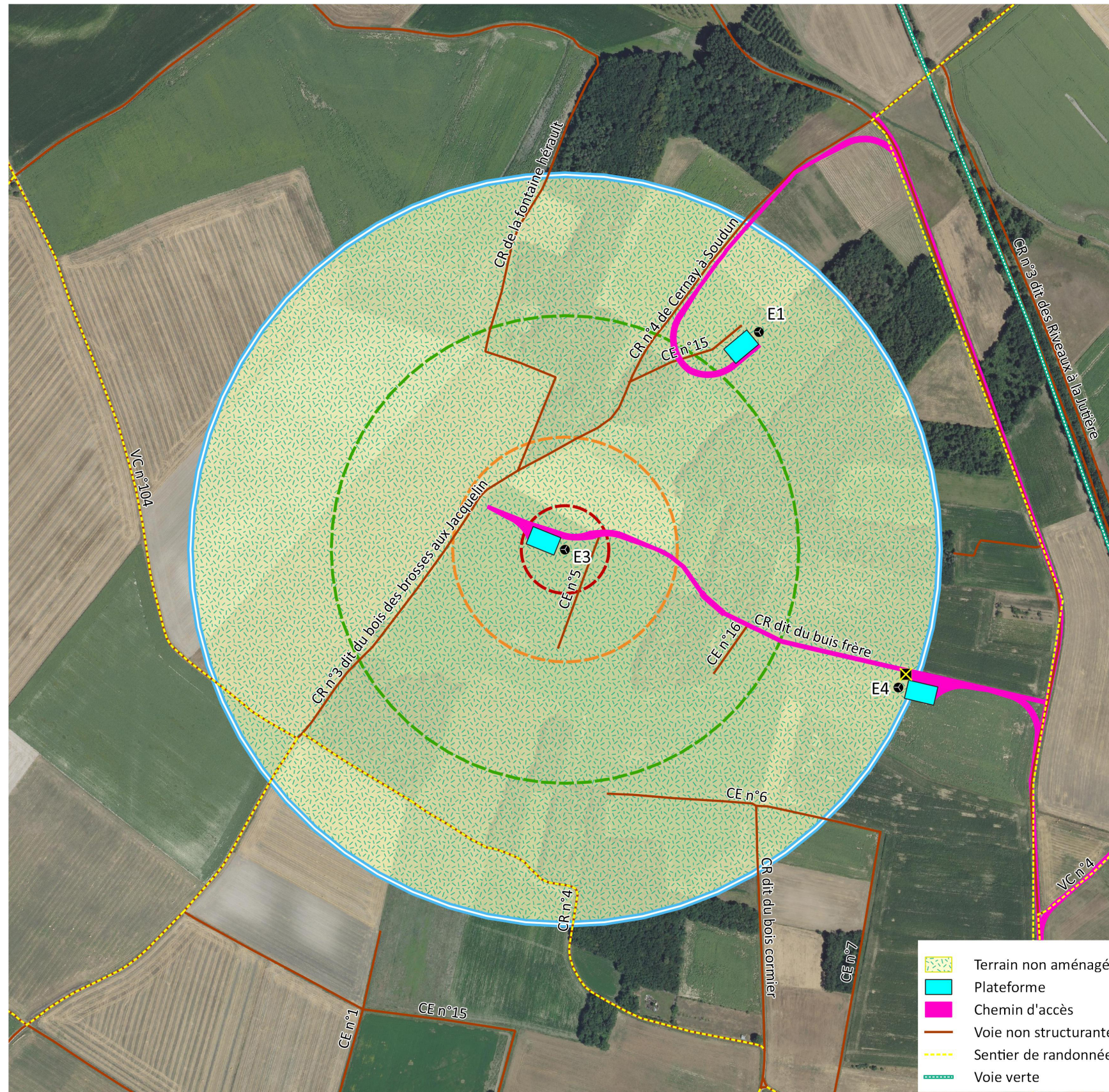
Carte 17 : Synthèse des risques pour l'éolienne E3
