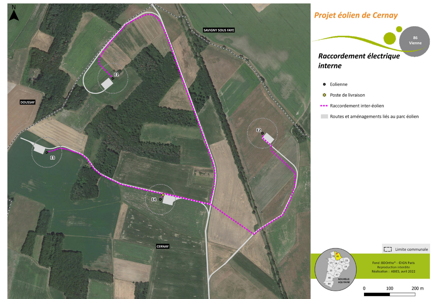
Carte 12 : Plan du raccordement inter-éolien et du poste de livraison
