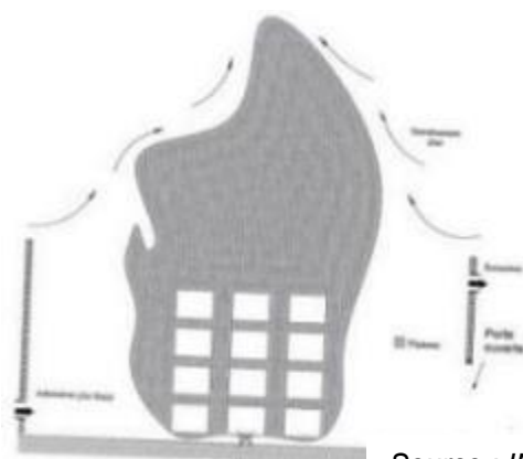
Figure 114 : Schéma de propagation du feu après effondrement de la toiture (feu bien ventilé)
