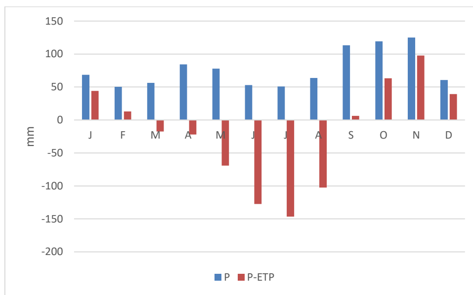
Figure 26 : Précipitations et bilan climatologique (station d'observation de Puy-Saint-Martin pour la pluie, Montélimar pour l'ETP)
