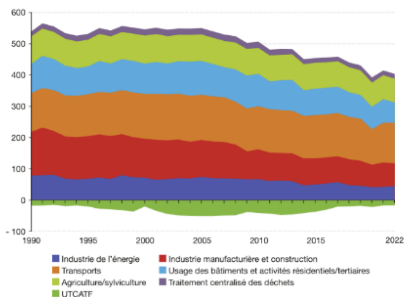
Figure 77 : Evolution des émissions sectorielles de GES en France entre 1990 et 2022 en Mt eq-CO 2
