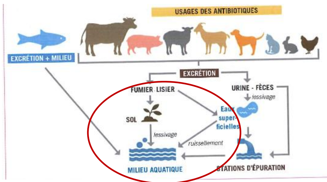
Figure 95 : Devenir des antibiotiques vétérinaires et contamination de l'environnement – Poulets : voies en rouge
