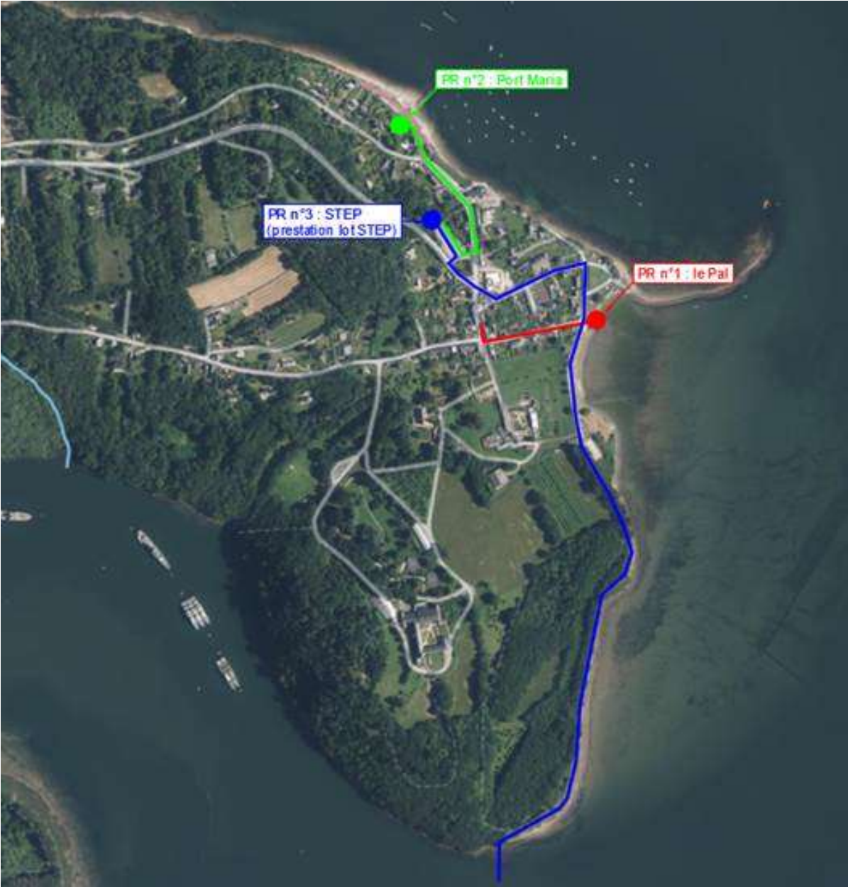
Vue du projet de travaux de réseau de refoulement des eaux usées et traitées de Landévennec.
