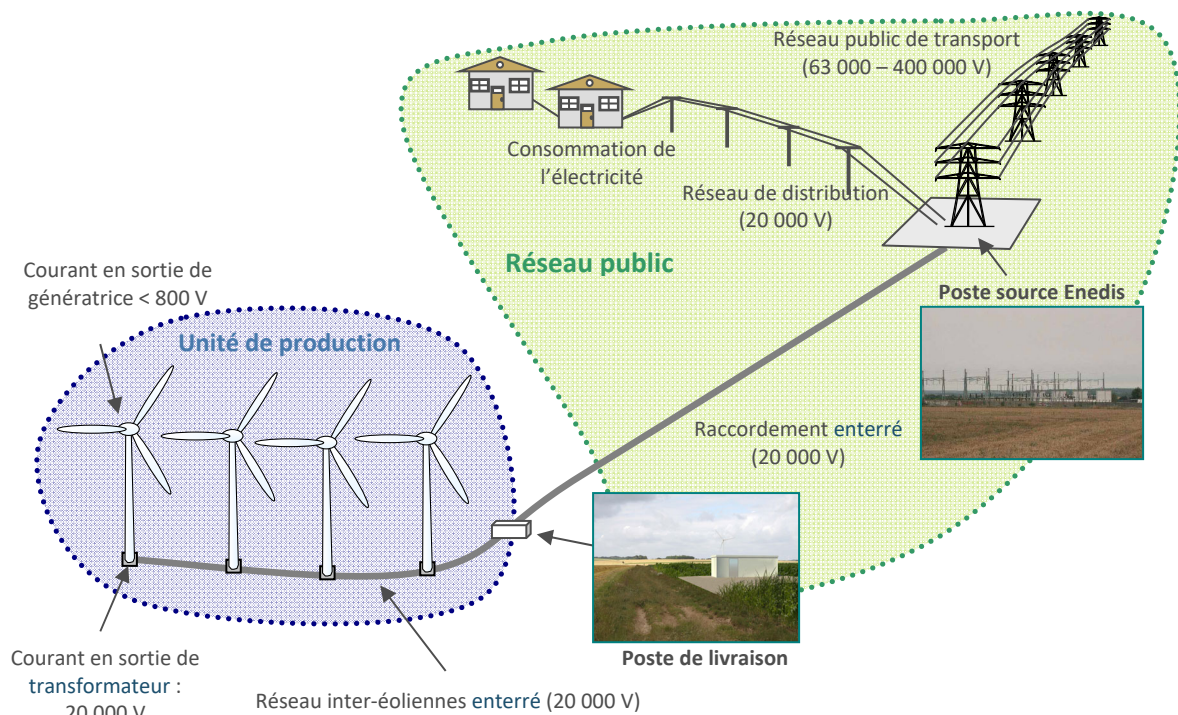
Figure 6 - Fonctionnement d'un parc éolien
