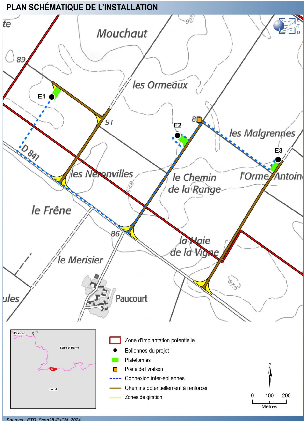
Carte 10 - Plan schématique de l'installation
