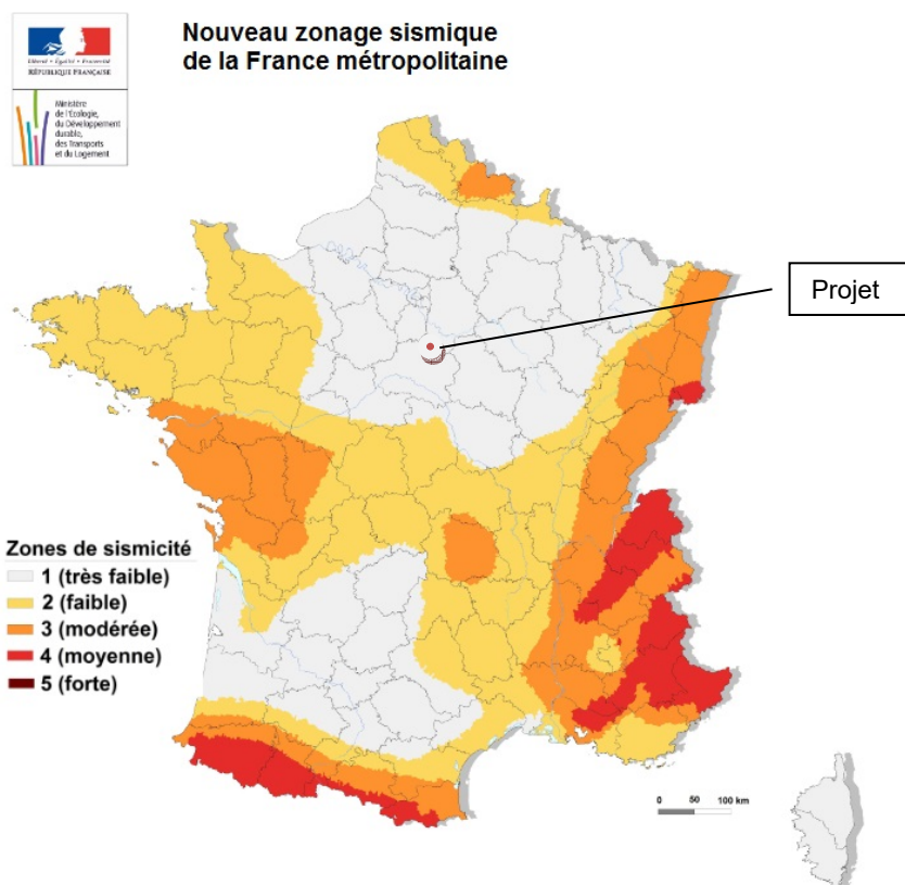
Figure 4 - Zonage sismique de la France métropolitaine et de la zone d'étude
