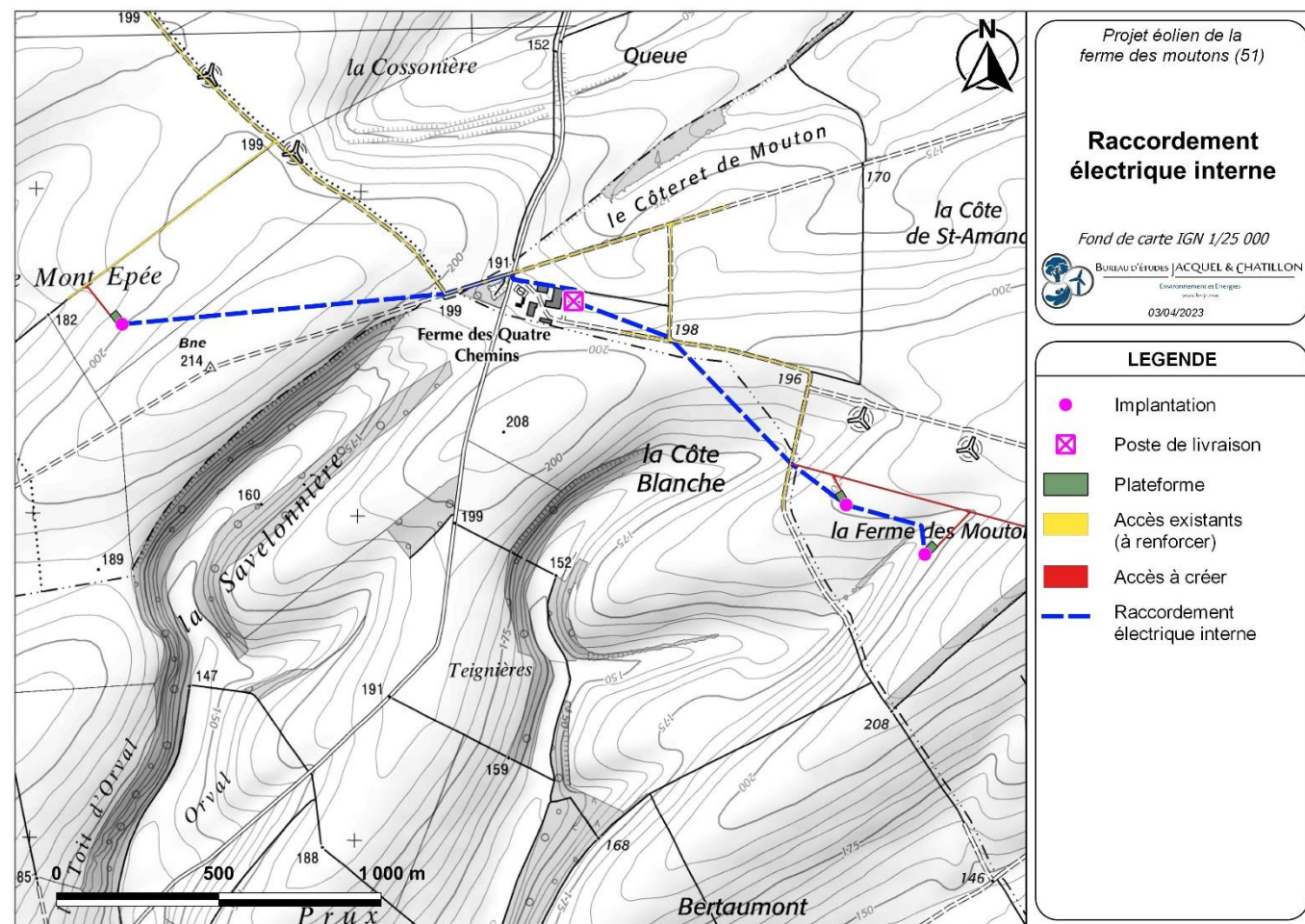
Carte 19 : Réseau inter-éolien du projet (Source : BE Jacquel et Chatillon)
