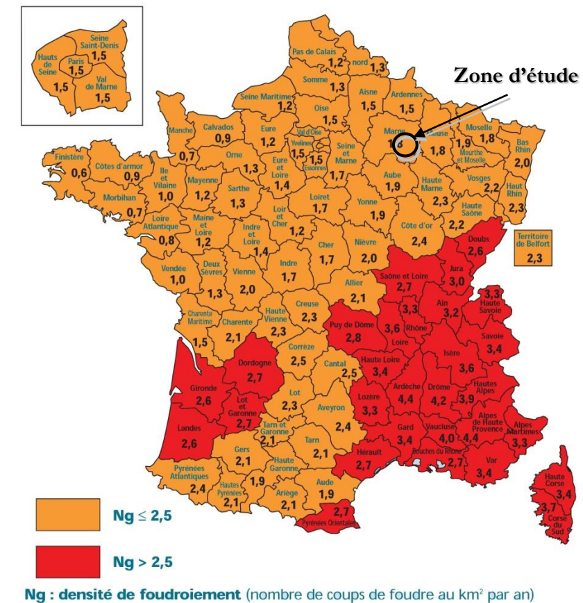
Carte 9 : Densité de foudroiement en France par département (Source : SOULE, 2003)
