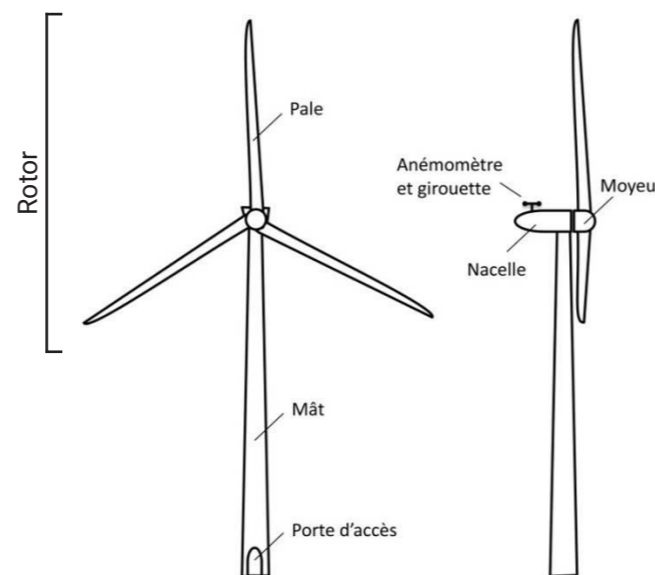
Figure 1. Schéma type d'un aérogénérateur
