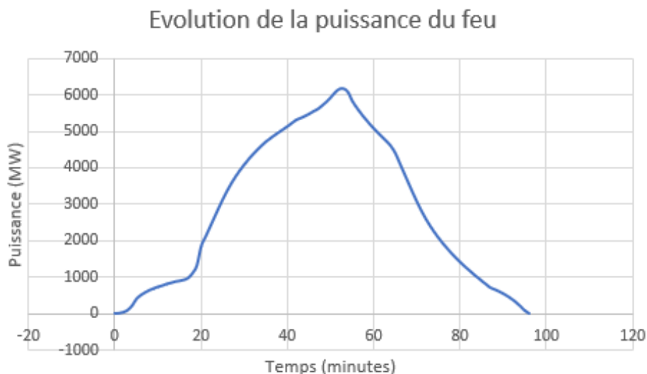
Figure 2 - Puissance du feu pour la cellule 1
