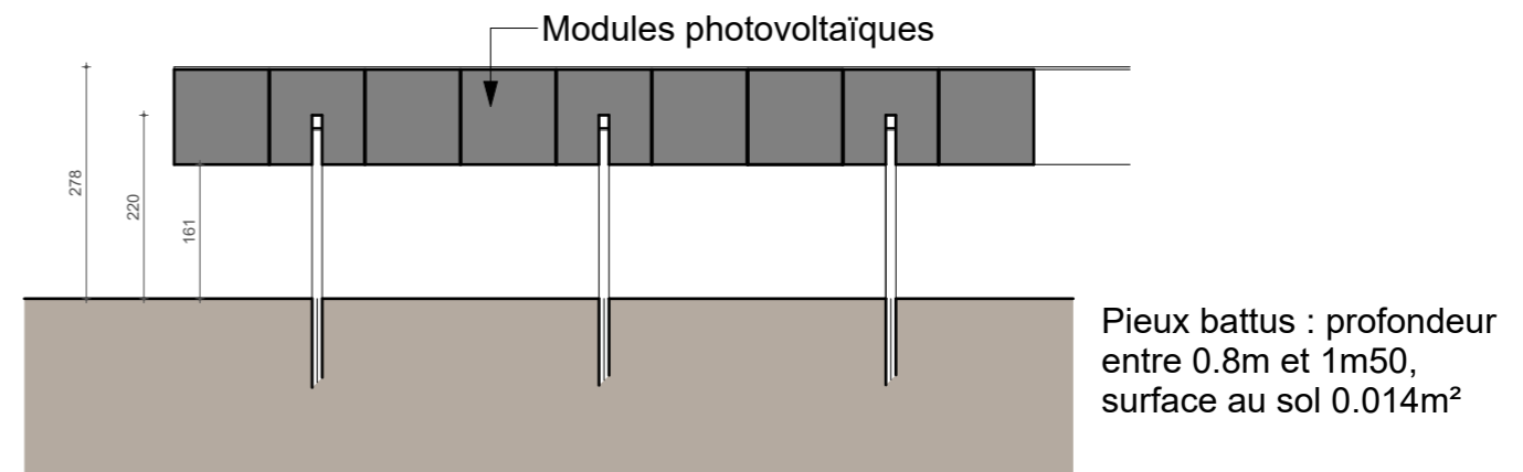
ELEVATION ARRIERE D'UNE CHAINE DE MODULES EN SERIE inclinaison 27°
