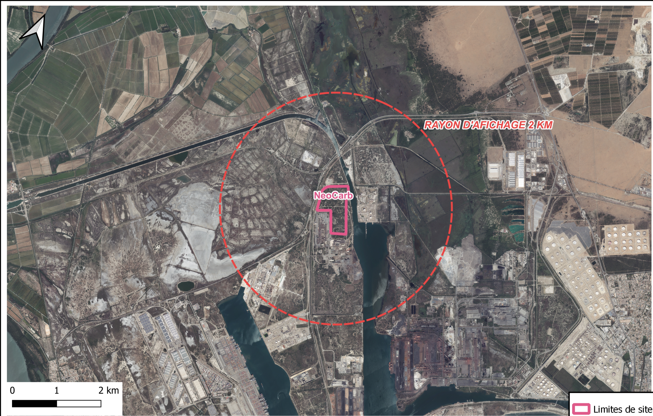
Plan de situation du projet NeoCarb (1/50 000)
