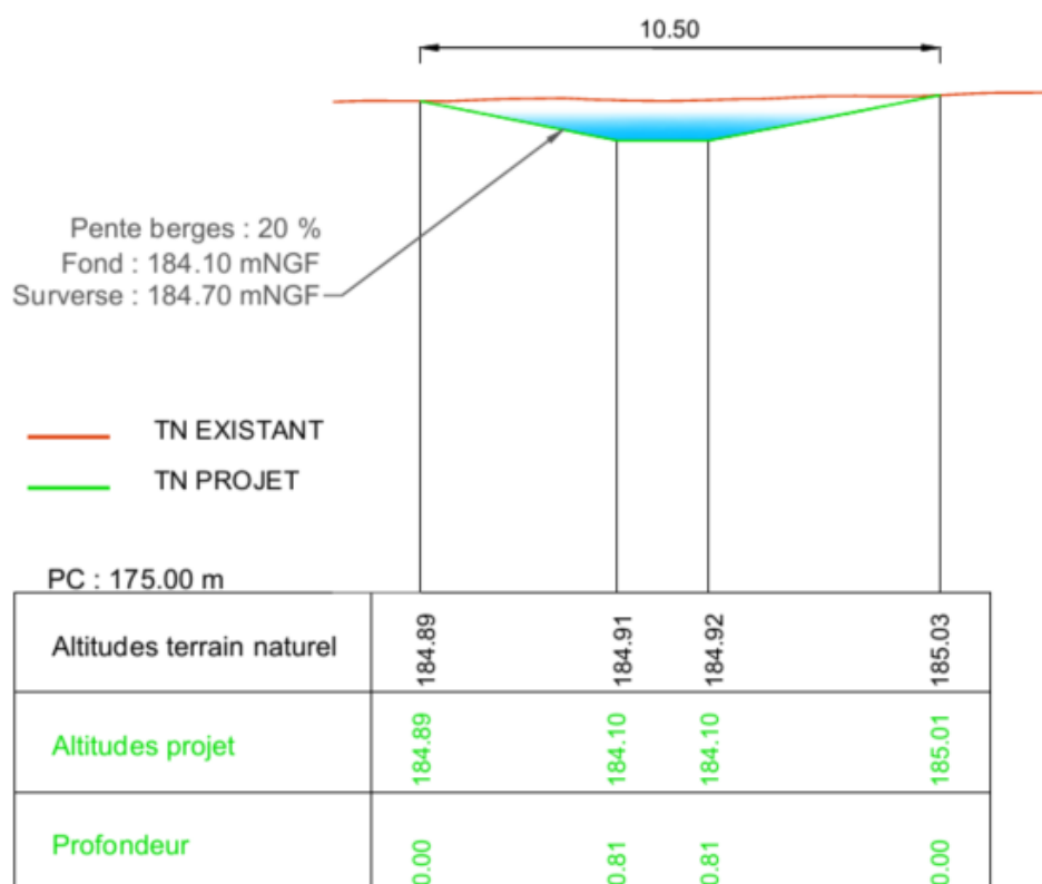
Illustration 38 : Vue en coupe d'une mare
