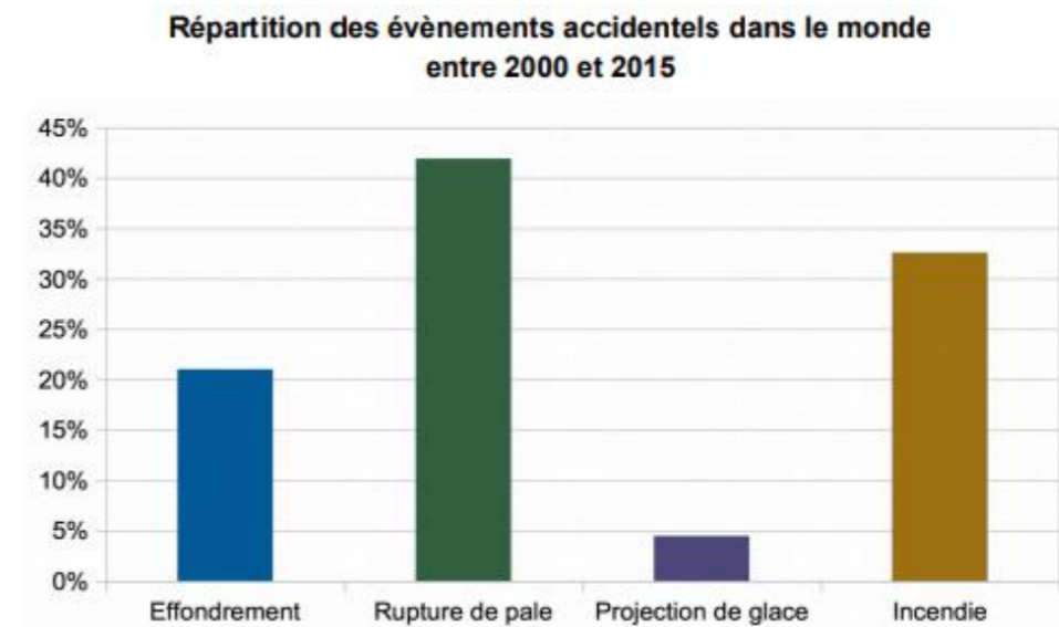
Figure 26 : Répartition des accidents liés à des parcs éoliens dans le monde entre 2000 et 2015
