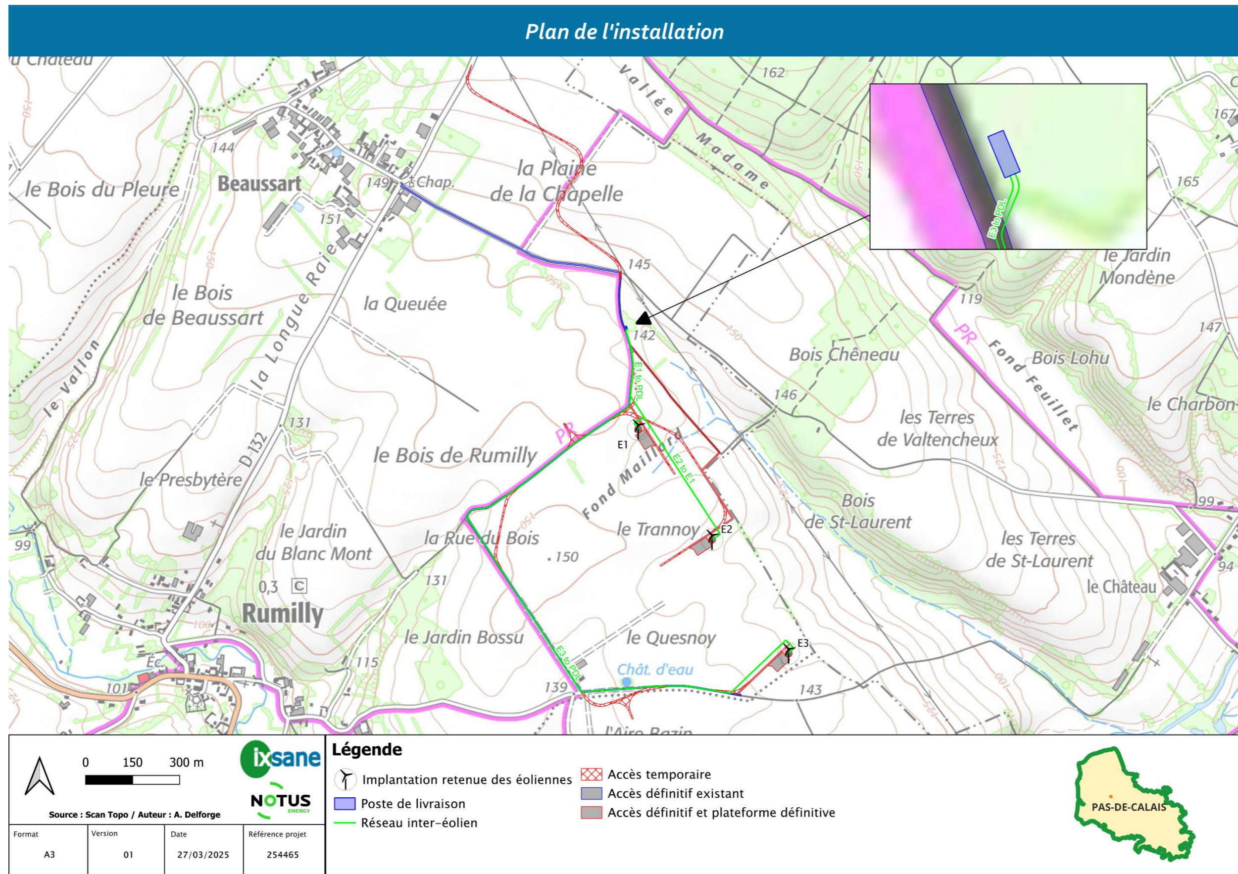
Figure 22 : Plan de l'installation
