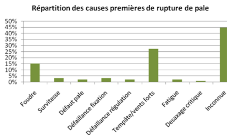
Figure 28 : Répartition des causes premières de rupture de pale
