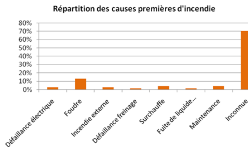
Figure 29 : Répartition des causes premières d'incendie
