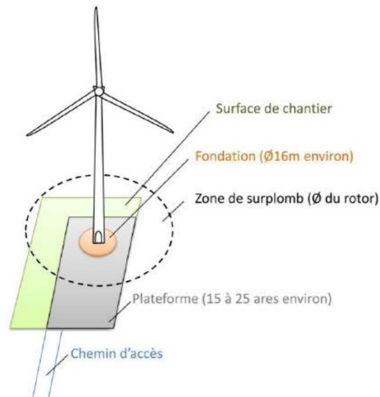
Figure 21 : Illustration des emprises au sol d'une éolienne
