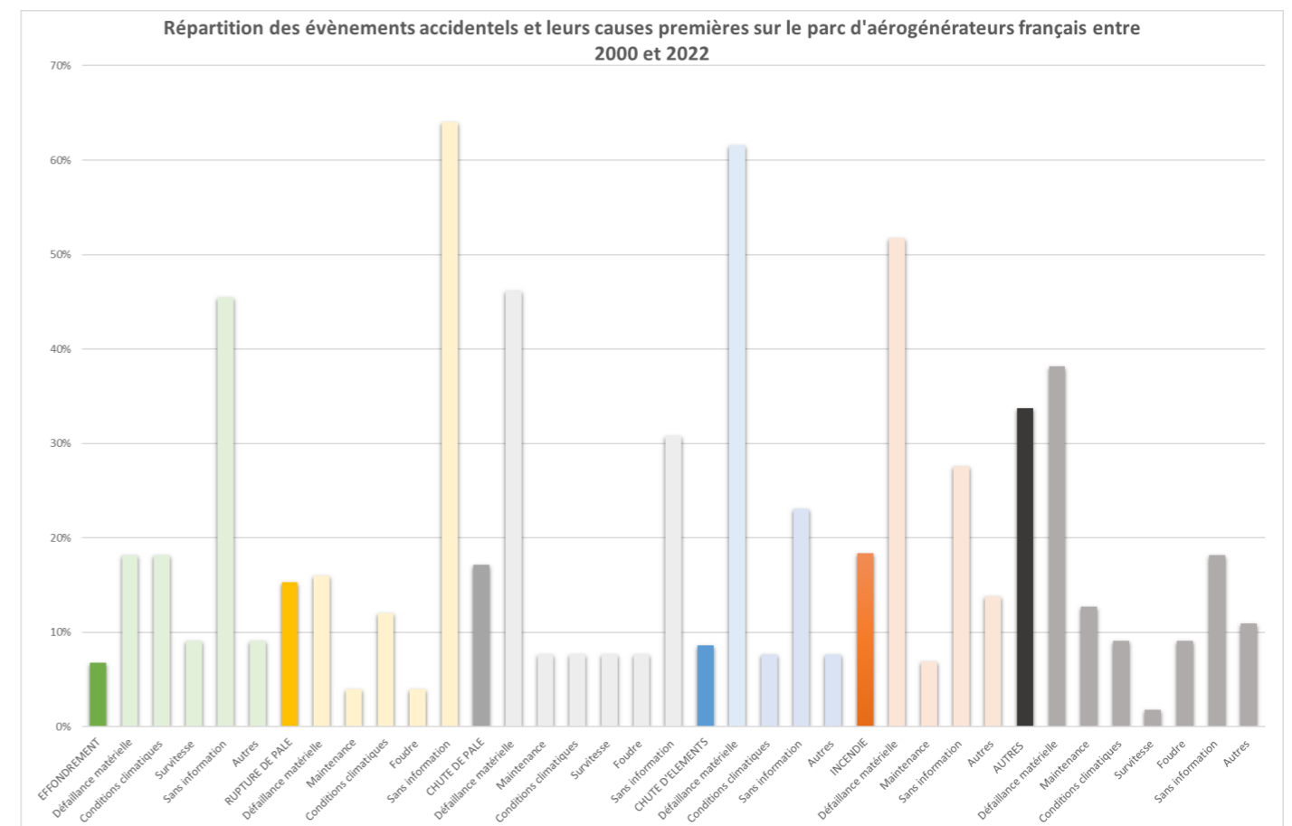
Figure 25 : Répartition des événements accidentels sur les parcs éoliens français entre 2000 et 2022
