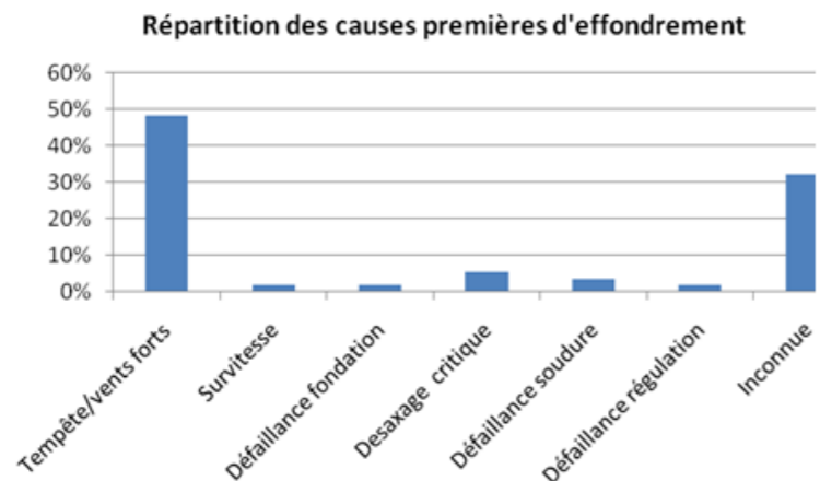
Figure 27 : Répartition des causes premières d'effondrement
