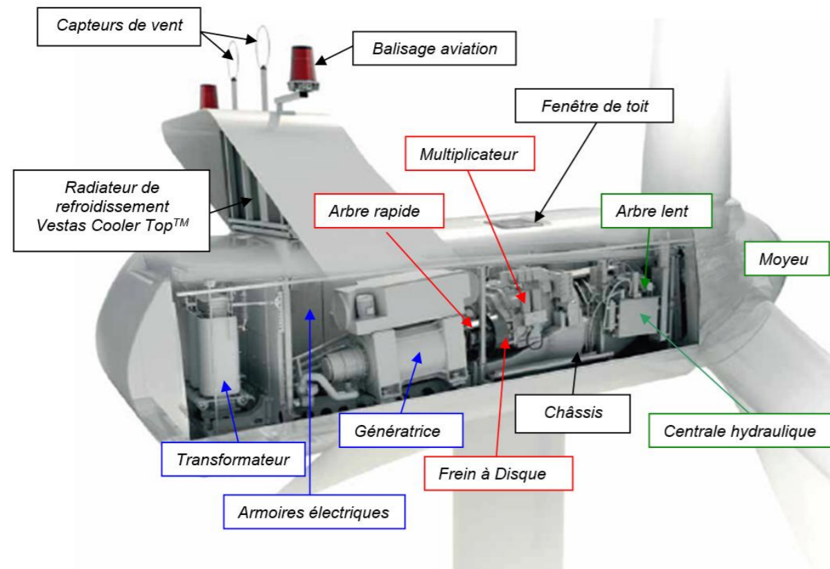
Figure 5 : Exemple de schéma illustrant les composants de la nacelle (Source : Vestas)
