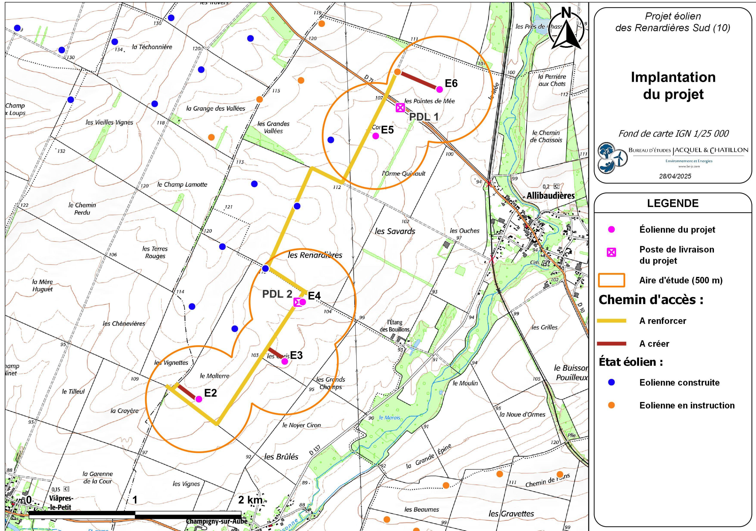
Carte 21 : Configuration de l'installation (Source : BE Jacquel et Chatillon)
