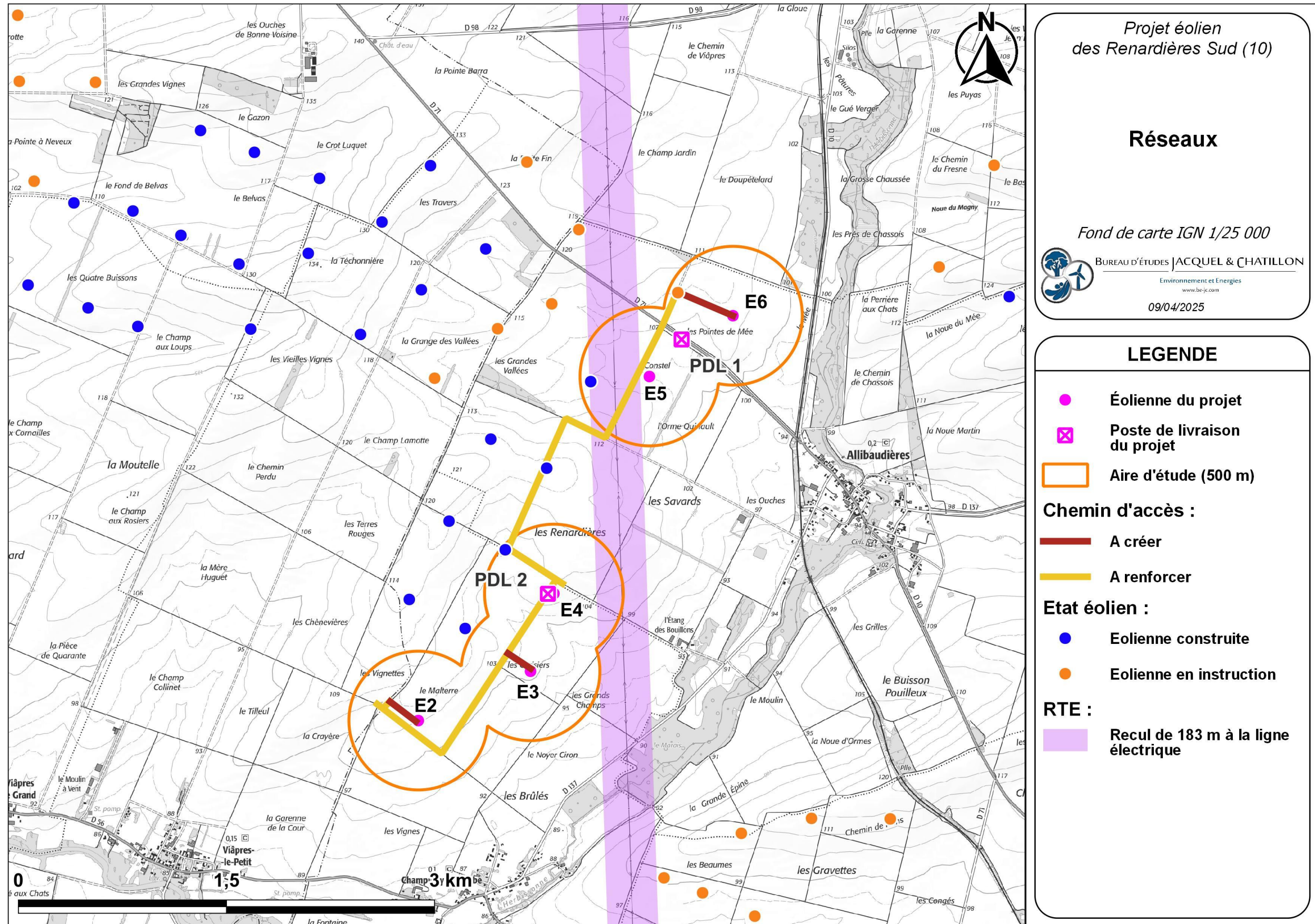
Carte 15 : Réseaux (Source : BE Jacquiel et Chatillon)
