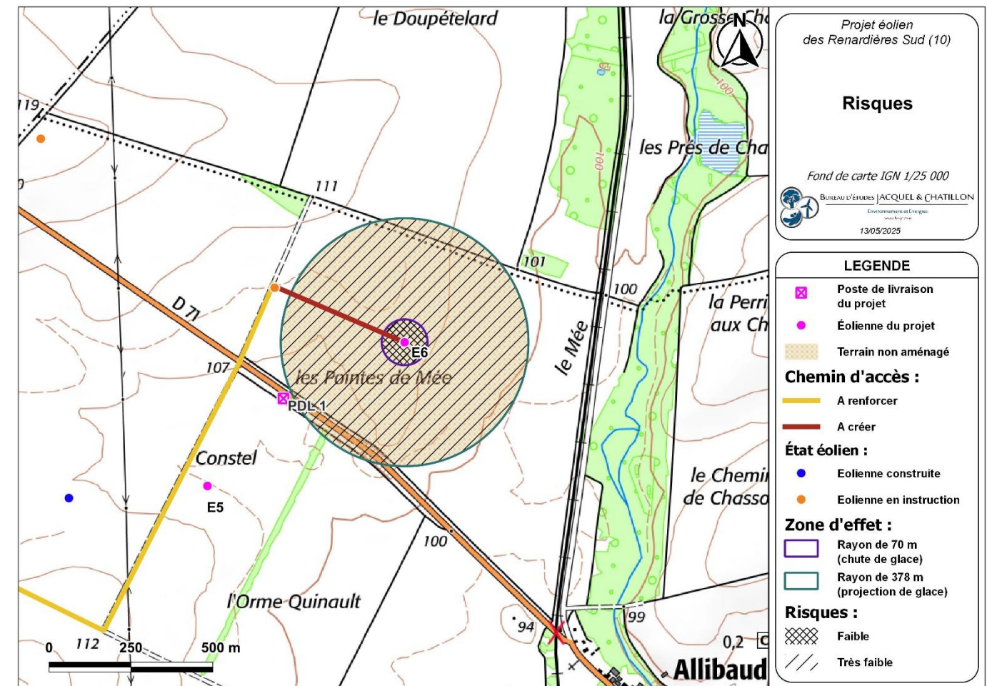
Carte 33 : Éolienne n°5 – Risques liés à la chute et à la projection de glace (Source : BE Jacquel et Chatillon)
