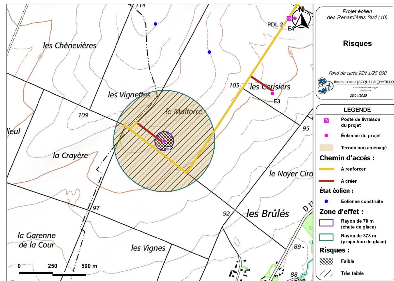
Carte 25 : Éolienne n°1 – Risques liés à la chute et à la projection de glace (Source : BE Jacquel et Chatillon)
