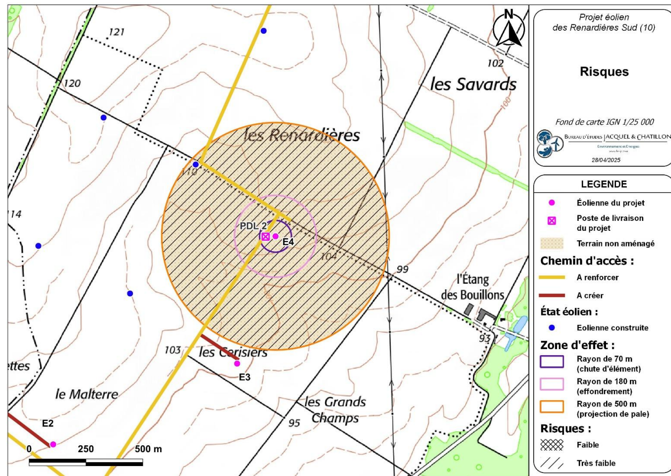
Carte 28 : Éolienne n°3 – Risques liés à l'effondrement de l'éolienne, à la chute d'élément de l'éolienne, et à la projection de pale ou de fragment de pale (Source : BE Jacquel et Chatillon)
