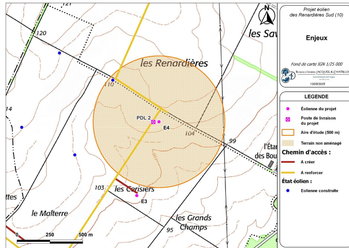
Carte 18 : Éolienne n°3 – Zones à enjeux (Source : BE Jacquel et Chatillon)
