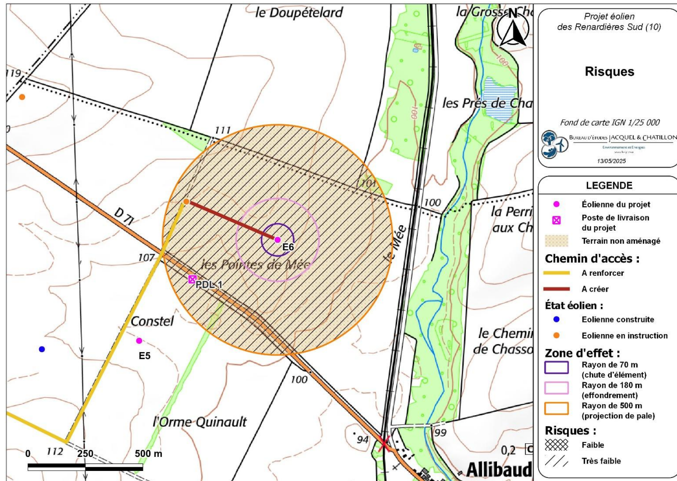
Carte 32 : Éolienne n°5 – Risques liés à l'effondrement de l'éolienne, à la chute d'élément de l'éolienne, et à la projection de pale ou de fragment de pale (Source : BE Jacquel et Chatillon)
