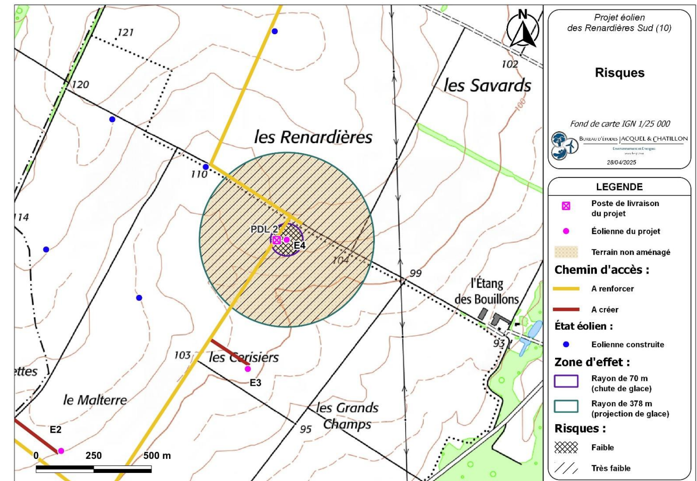
Carte 29 : Éolienne n°3 – Risques liés à la chute et à la projection de glace (Source : BE Jacquel et Chatillon)
