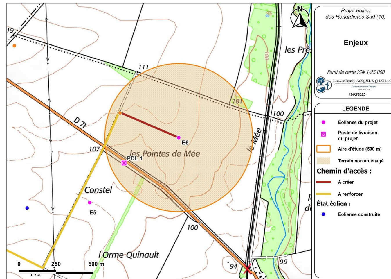
Carte 20 : Éolienne n°5 – Zones à enjeux (Source : BE Jacquel et Chatillon)
