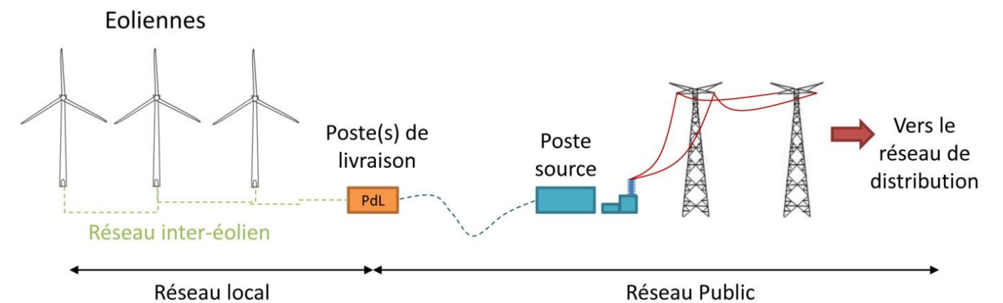
Figure 4 : Raccordement électrique des installations (Source : INERIS)
