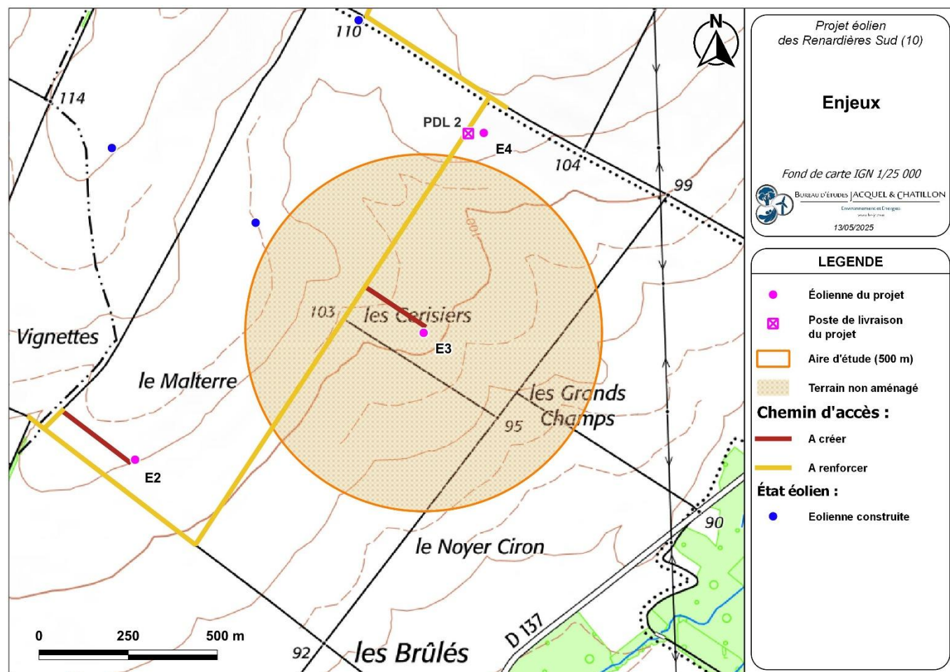
Carte 17 : Éolienne n°2 – Zones à enjeux (Source : BE Jacquel et Chatillon)
