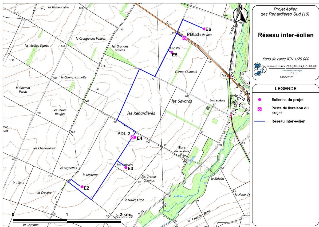
Carte 22: Réseau inter-éolien du projet (Source : Be Jacquiel et Chatillon, d'après données Innergex)
