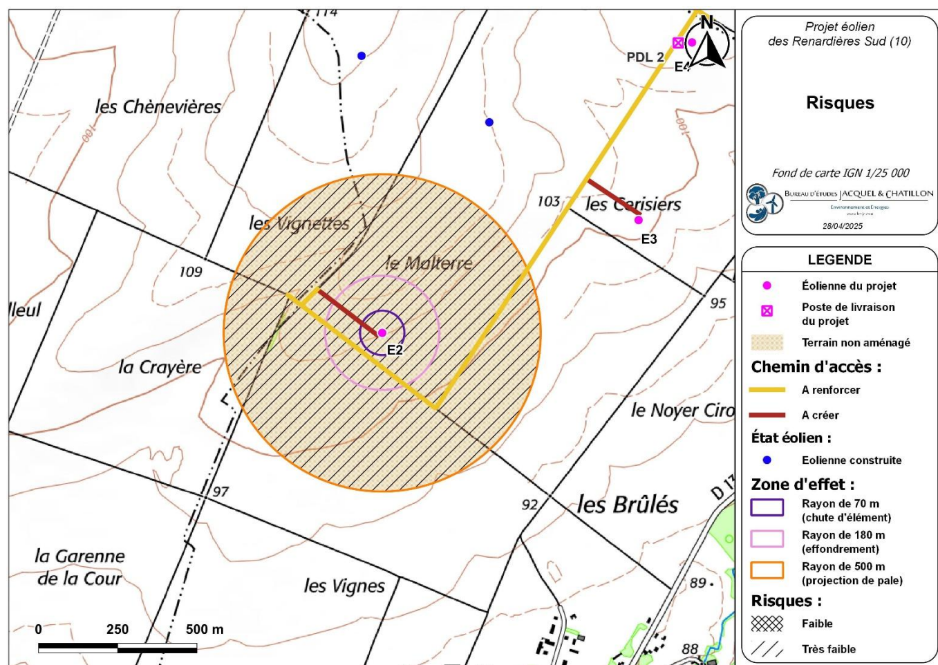
Carte 24 : Éolienne n°1 – Risques liés à l'effondrement de l'éolienne, à la chute d'élément de l'éolienne, et à la projection de pale ou de fragment de pale (Source : BE Jacquel et Chatillon)
