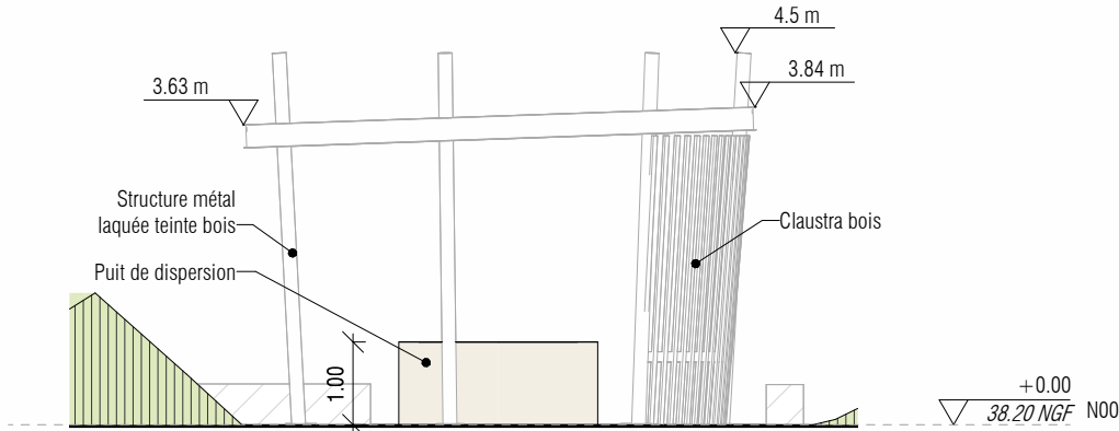
6 - Élévation Kiosque EST
