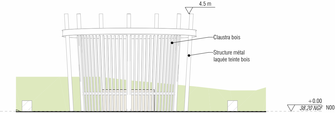
3 - Élévation Kiosque NORD
