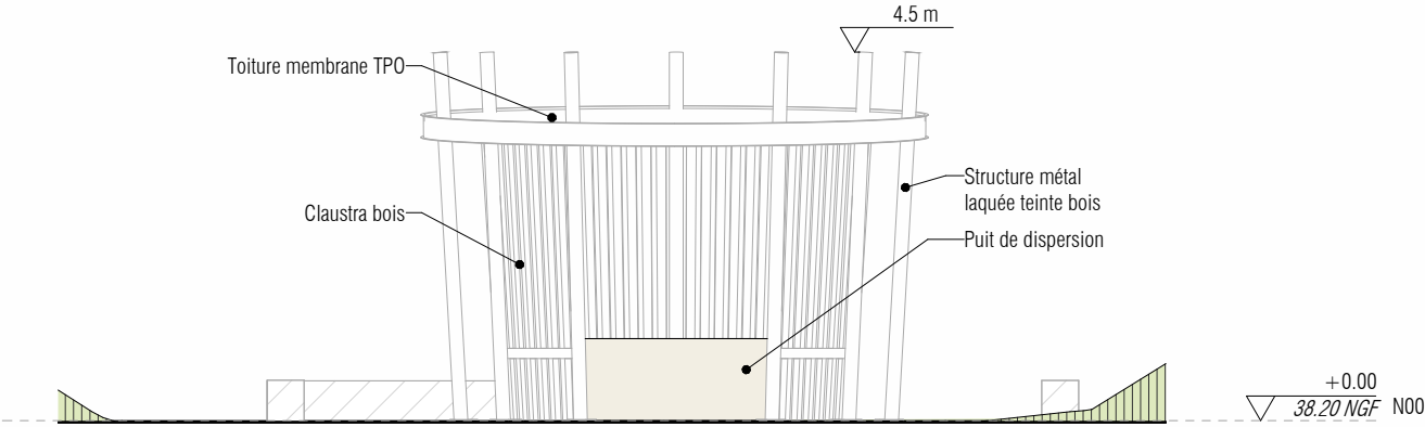
4 - Élévation Kiosque SUD
