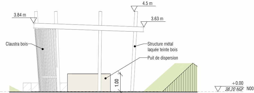
5 - Élévation Kiosque OUEST
