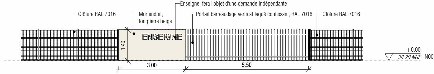
2 - Élévation Zoom sur entrée de parking
