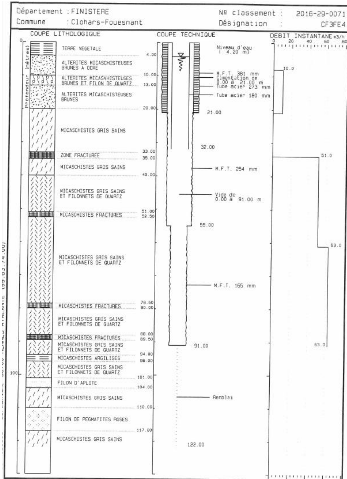
Figure 4 : Coupe technique de l'ouvrage CF3-FE4
