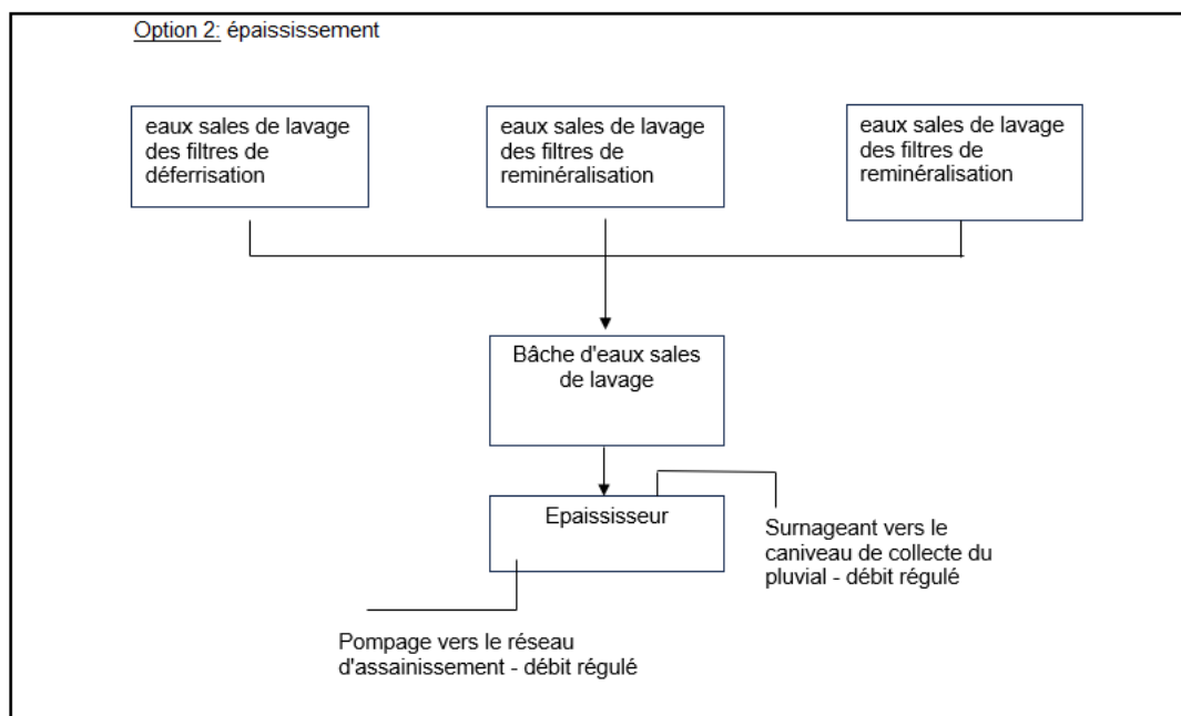
Figure 7 : Filière de rejet avec épaisseur
