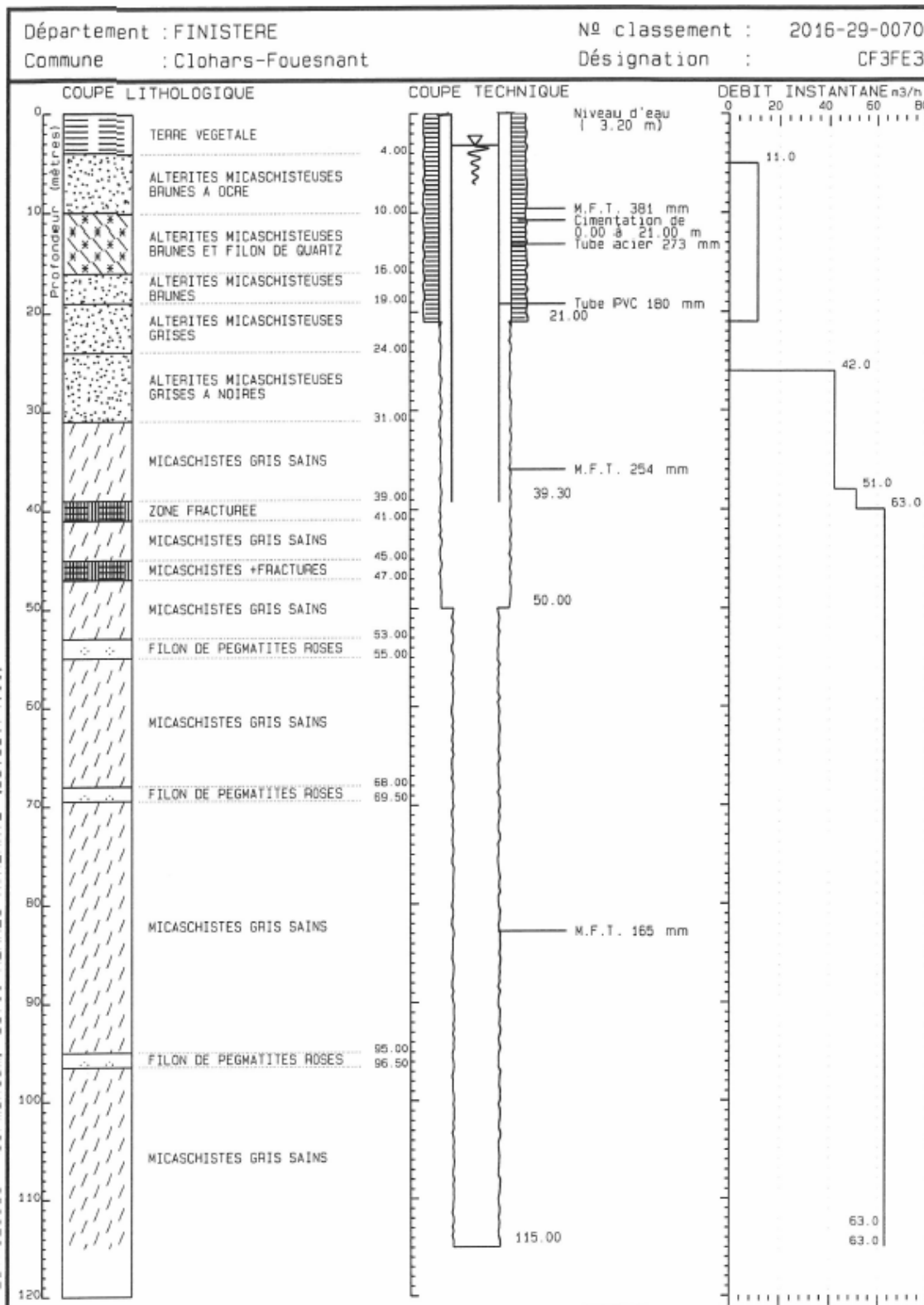
Figure 2 : Coupe technique de l'ouvrage CF3-FE3
