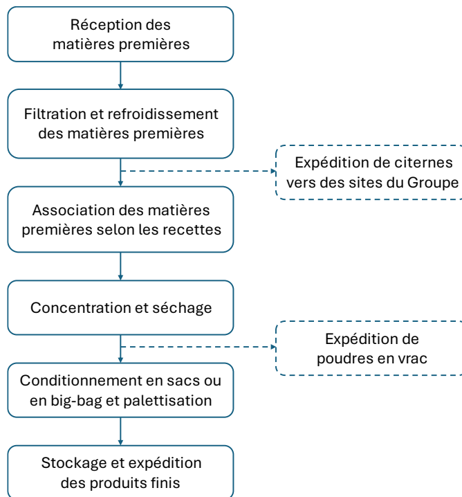
Figure 3 : Synoptique simplifié de l'activité du site
