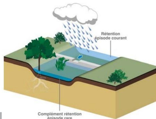
Figure - Noue à stockage successif : les eaux d'événements pluviaux courants sont stockées dans un premier tronçon en amont (pluie annuelle par exemple), tandis que le supplément d'eau dû à des événements plus rares est stocké dans un tronçon successif par un dispositif de surverse (pour les pluies décennales ou centennales par exemple). Source Architecture & Climat.
