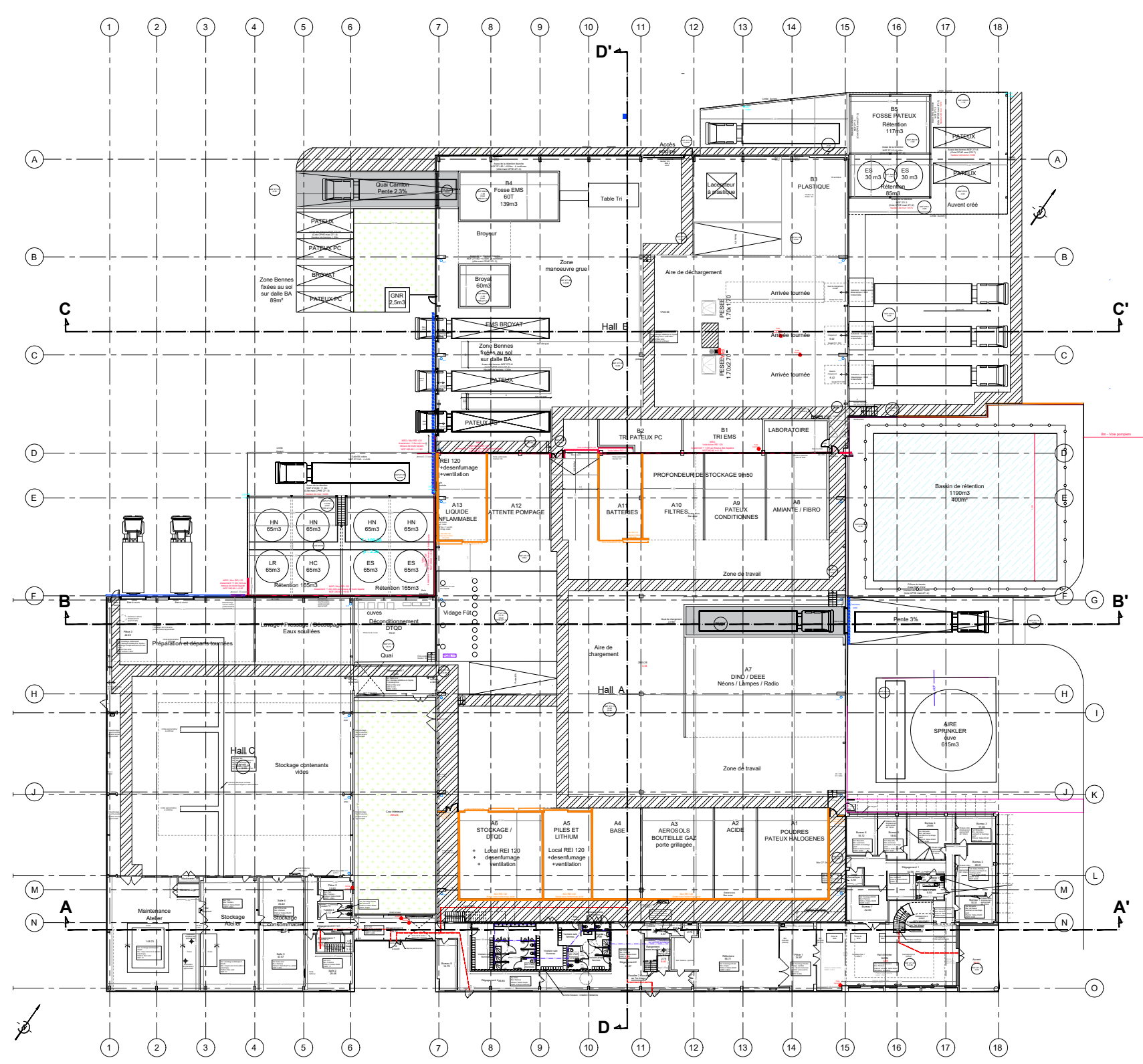
Plan de repérage coupes
