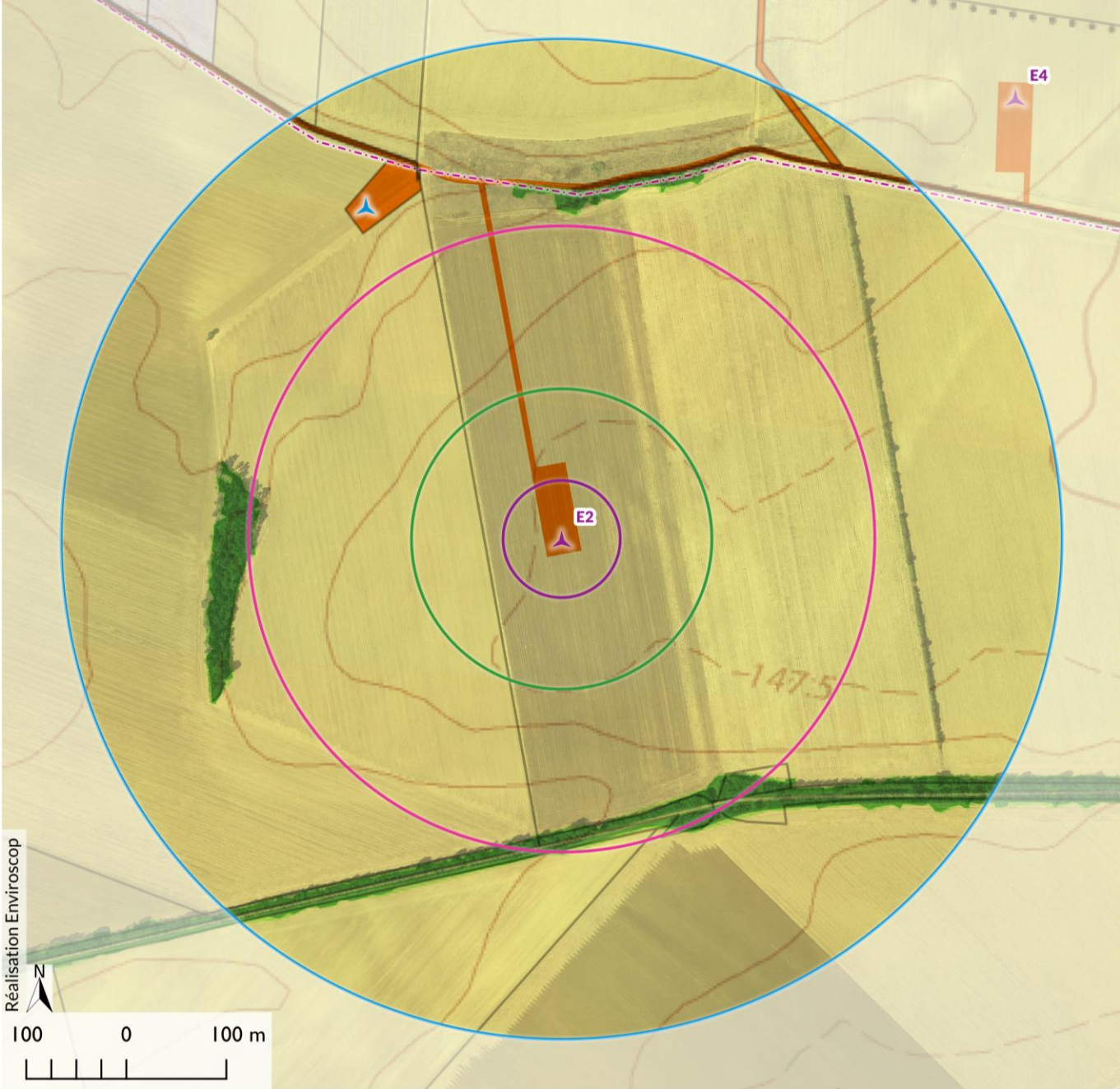
Carte 16 : Synthèse des risques de l'éolienne E2
