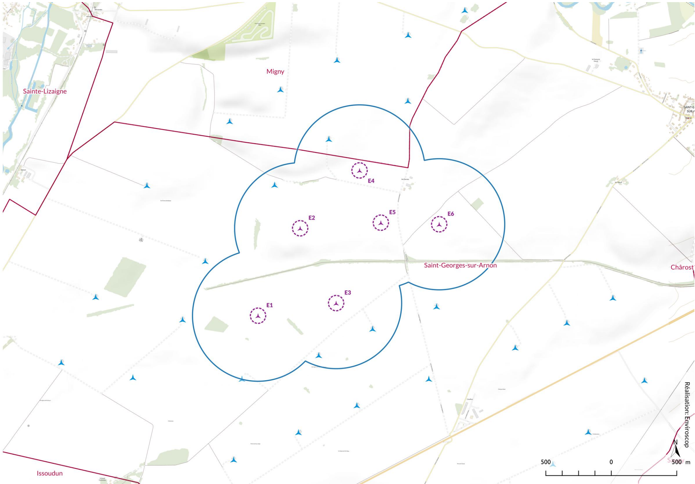
Carte 1 : Situation du Parc éolien les Coeurs de Boeuf et de l'aire d'étude de dangers Réalisation Enviroscop. Sources : Plan IGNv2, ADMIN Express, RWE
