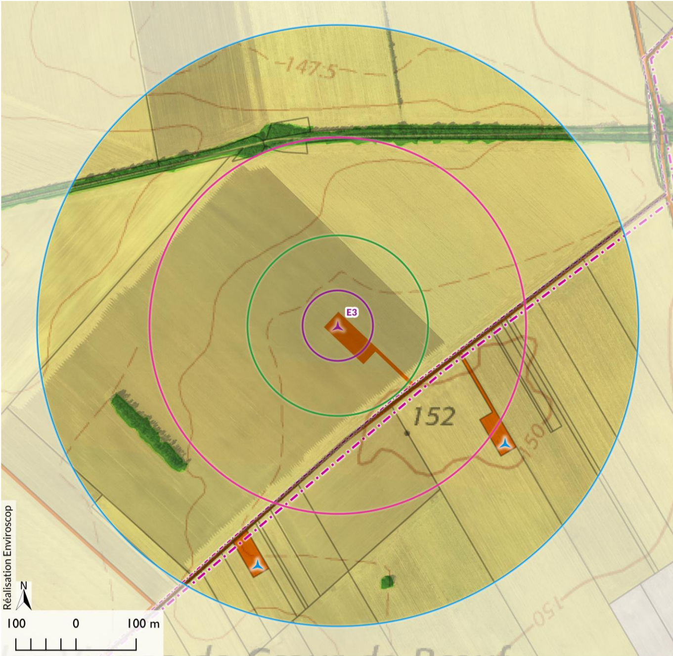
Carte 17 : Synthèse des risques de l'éolienne E3
