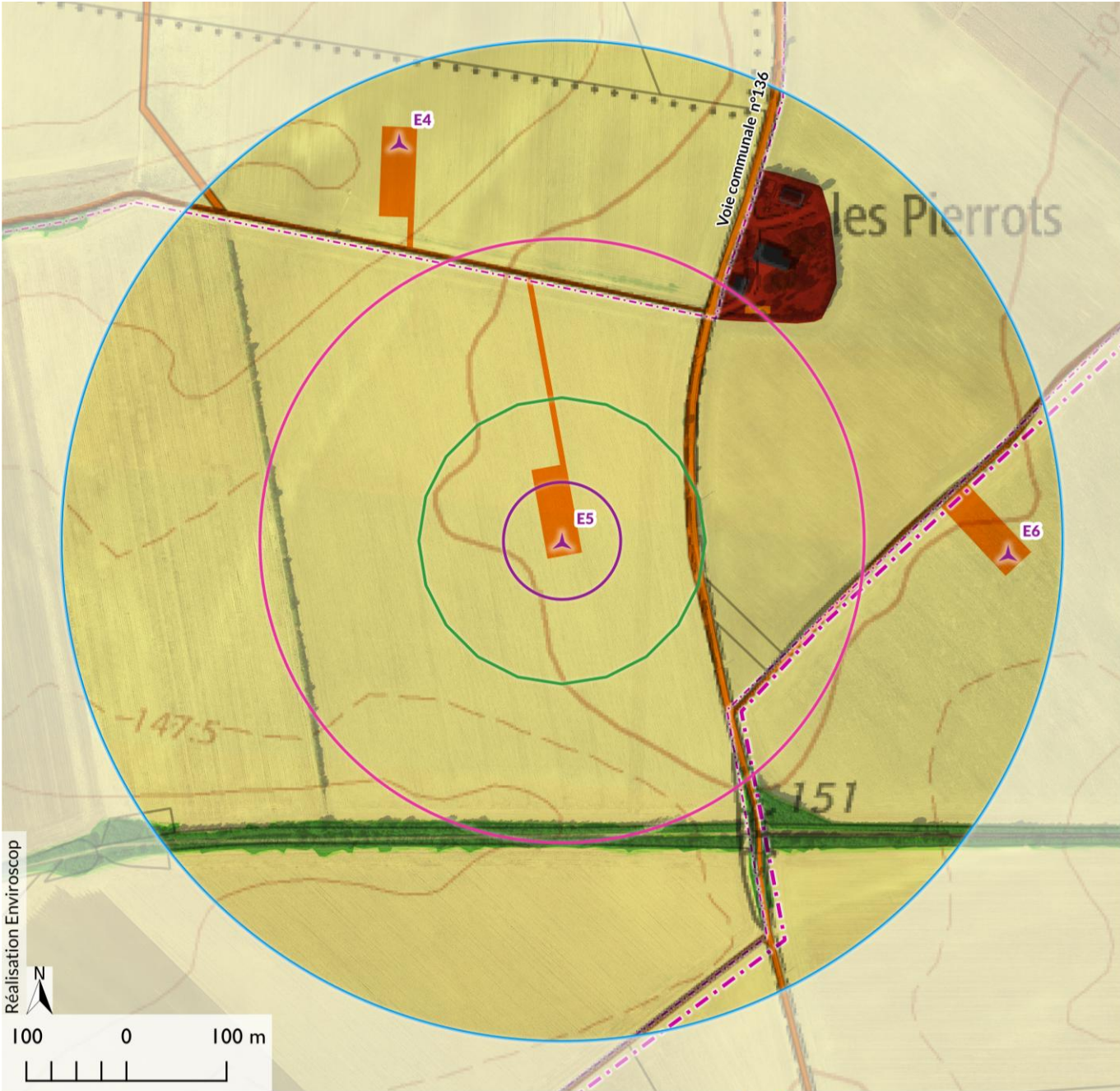
Carte 8 : Synthèse des risques de l'éolienne E5
