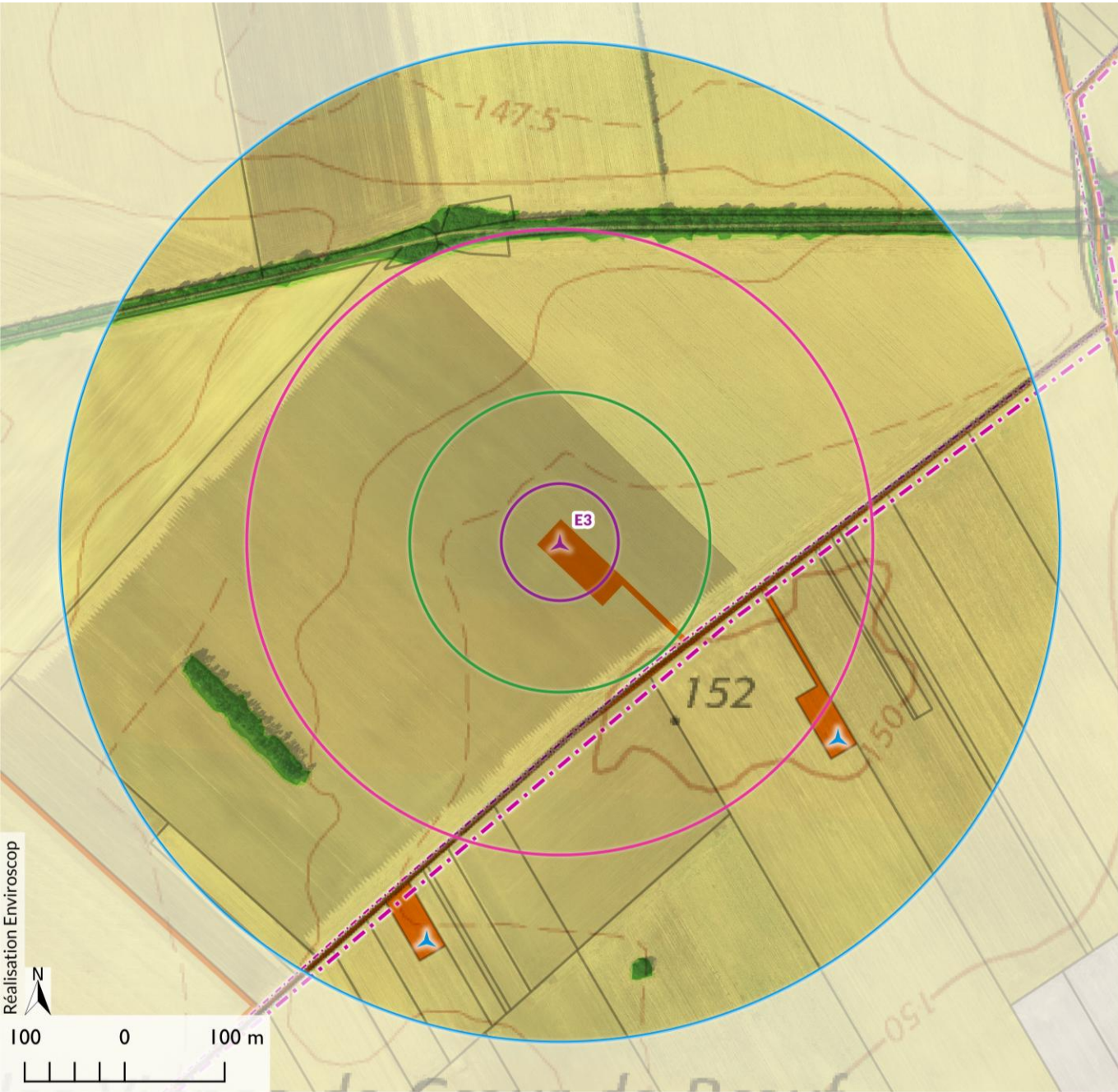
Carte 6 : Synthèse des risques de l'éolienne E3
