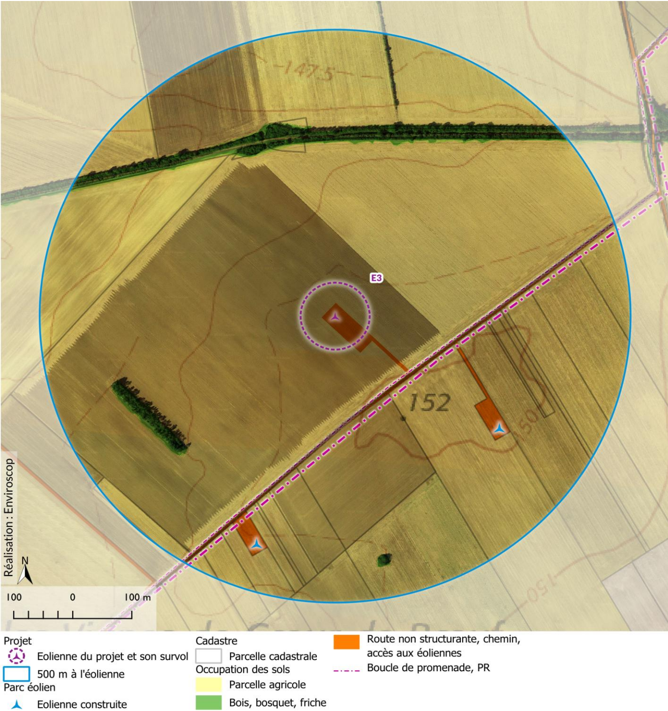
Carte 10 : Synthèse de l'environnement dans l'aire d'étude de dangers (500 m) de E3
