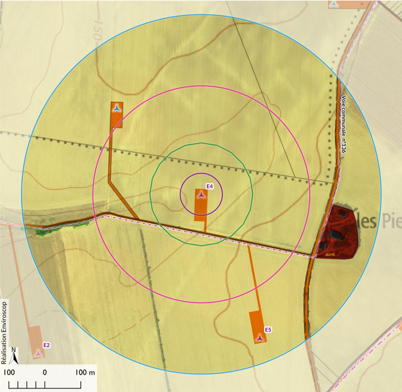
Carte 18 : Synthèse des risques de l'éolienne E4
