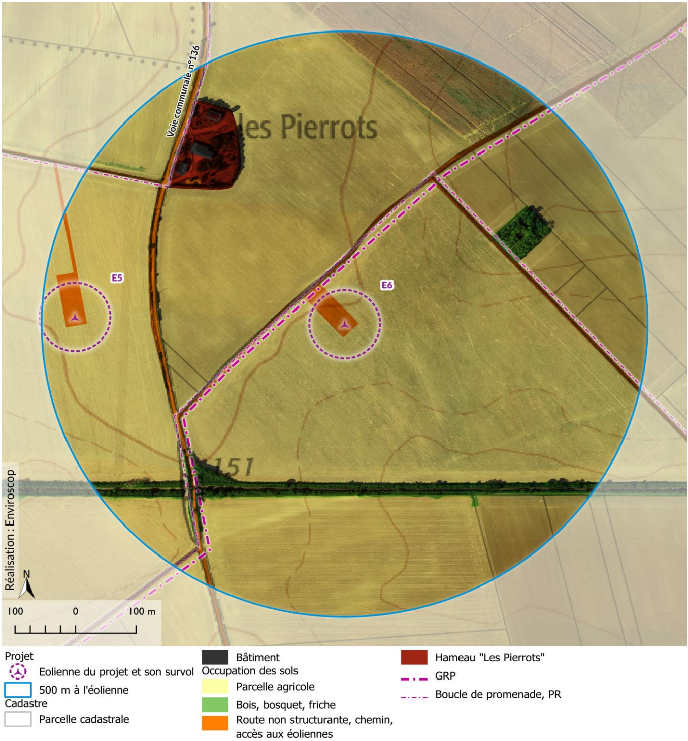
Carte 13 : Synthèse de l'environnement dans l'aire d'étude de dangers (500 m) de E6
