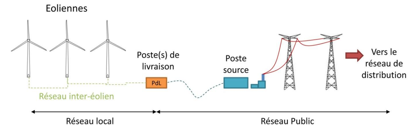
Figure 5 : Principe du raccordement électrique des installations
