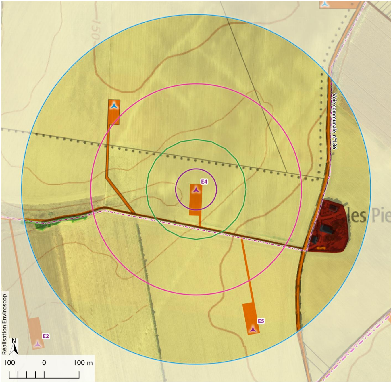
Carte 7 : Synthèse des risques de l'éolienne E4
