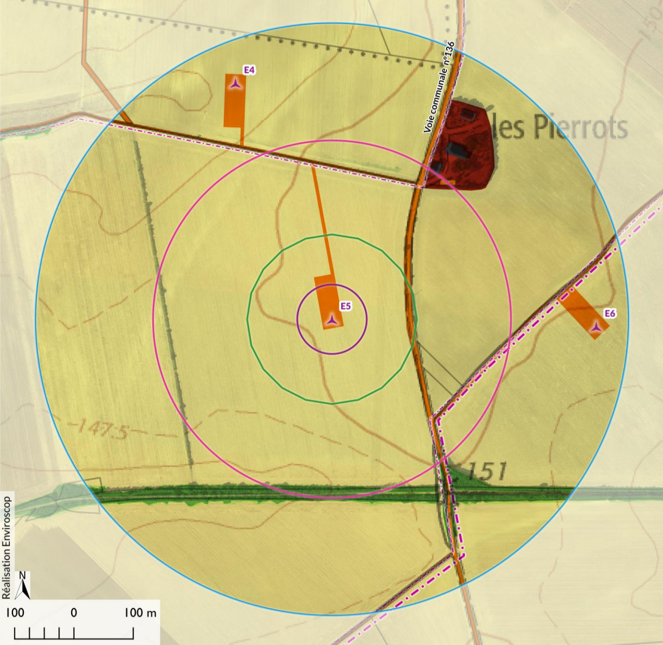
Carte 19 : Synthèse des risques de l'éolienne E5
