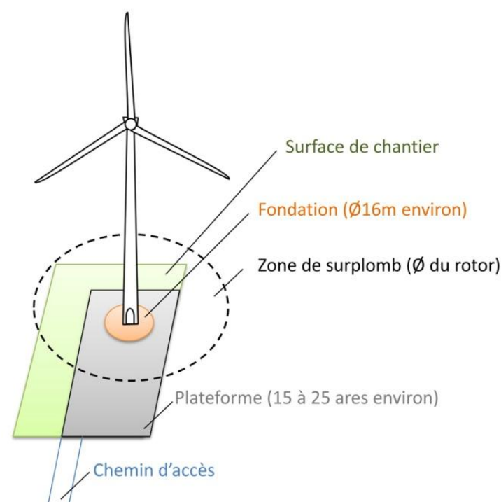
Figure 4 : Schéma de principe des emprises au sol d'une éolienne
