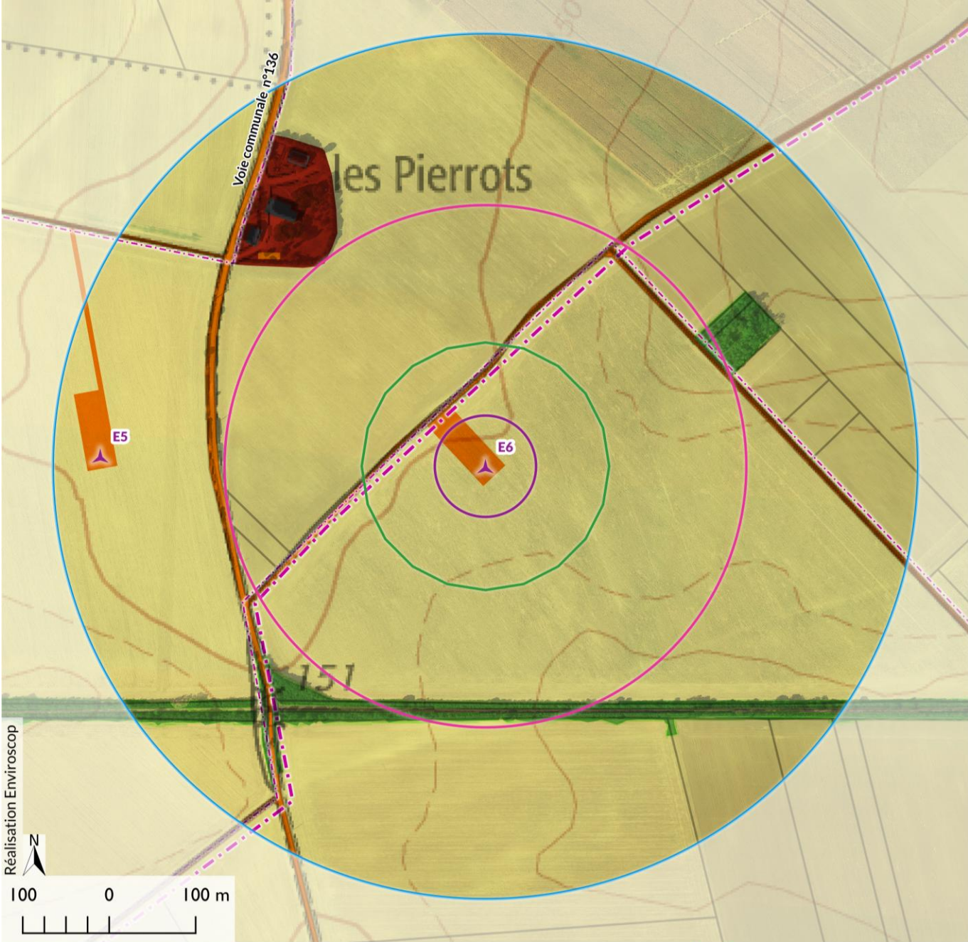
Carte 20 : Synthèse des risques de l'éolienne E6
