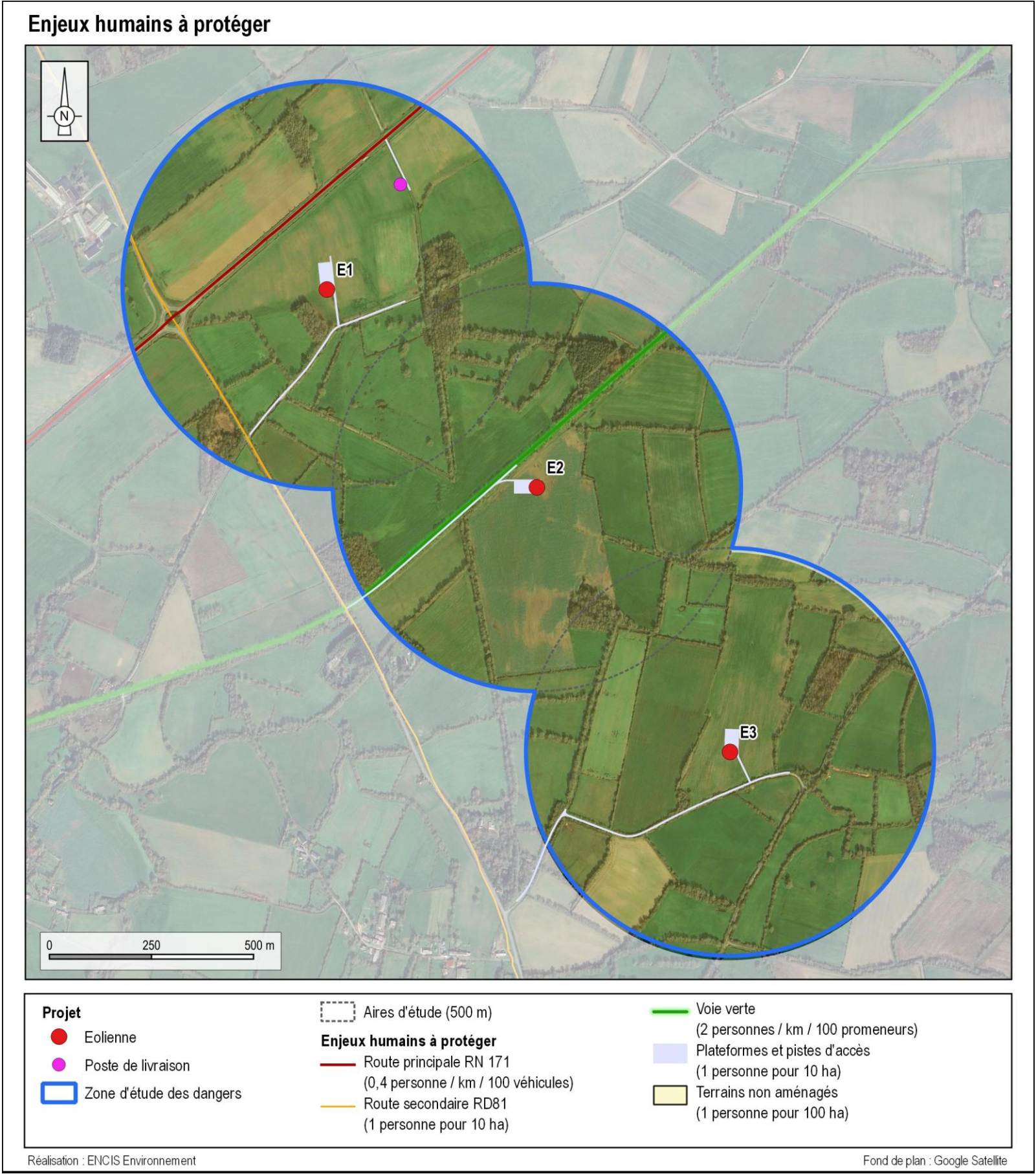
Carte 10 : Les intérêts à protéger (enjeux) au sein des aires d'étude des dangers du parc des Éoliennes de l'Hôtel de France
