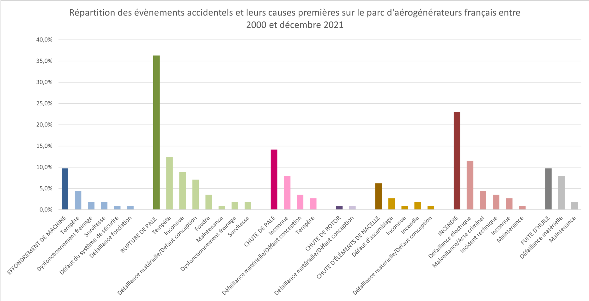
Figure 6 : Répartition des accidents et de leurs causes premières sur le parc éolien français entre 2000 et décembre 2021 (Source : ENCIS Environnement, d'après le Guide technique, mai 2012)
