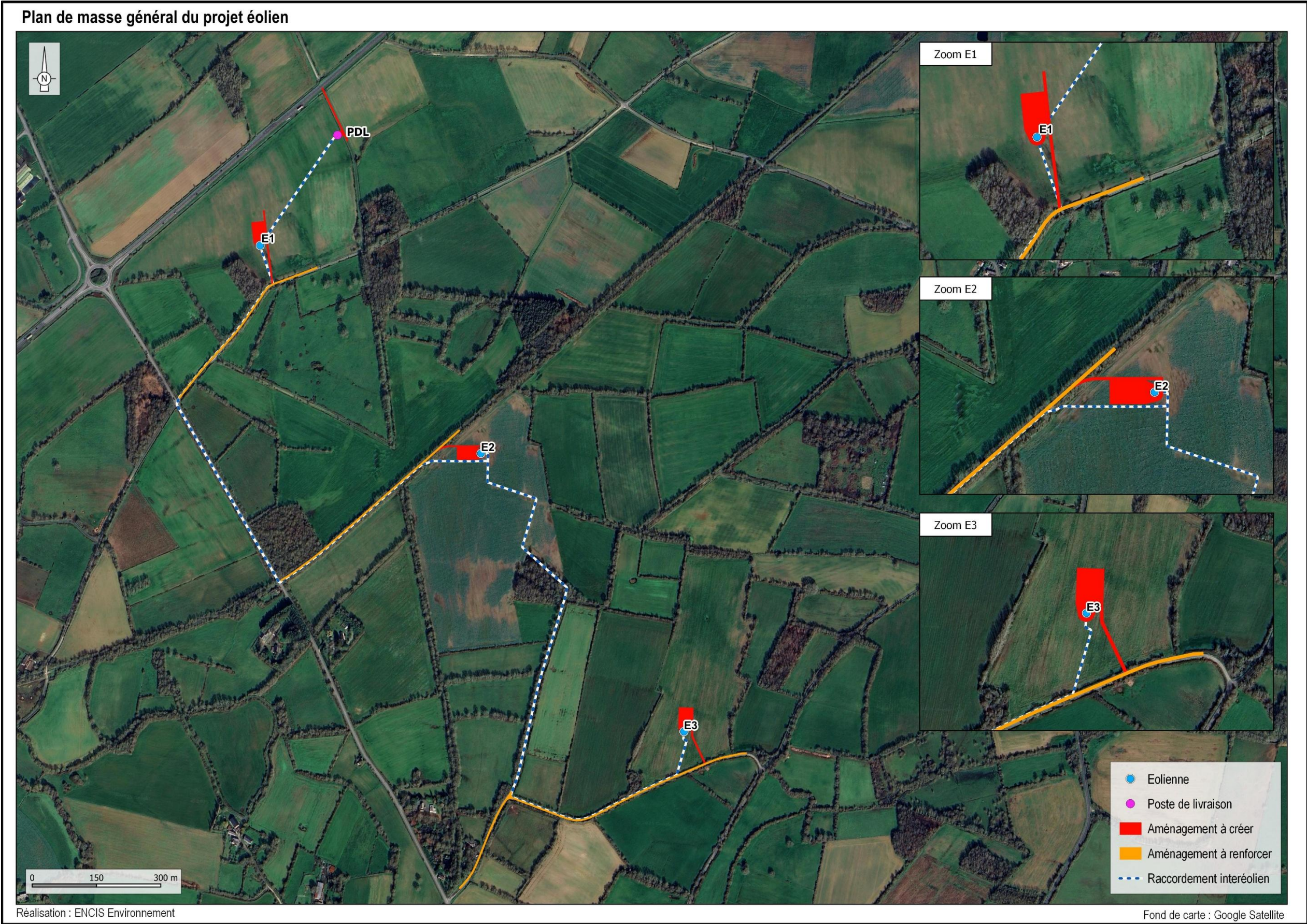
Carte 11 : Plan du projet de parc éolien de l'Hôtel de France
