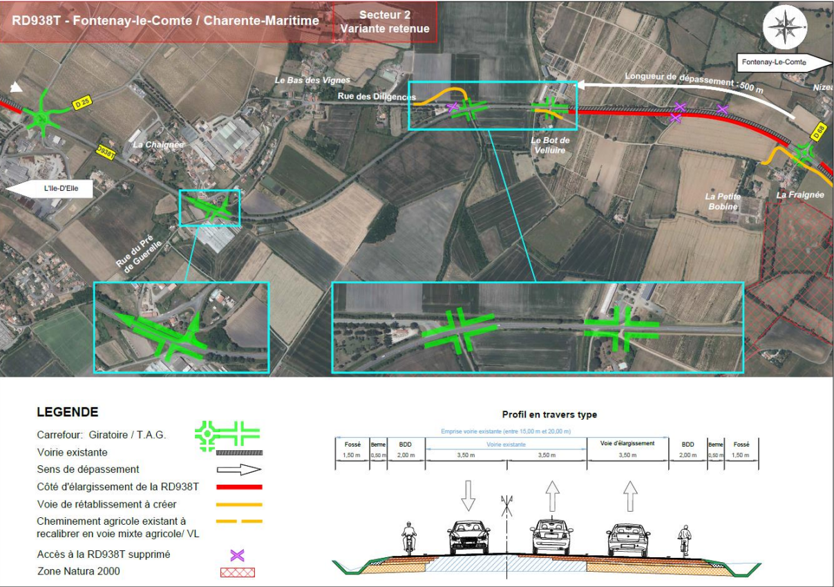
Figure 38 : Plan de la variante retenue sur le secteur 2
