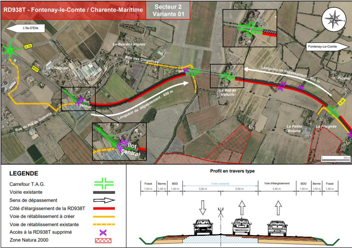
Figure 35 : Présentation de la variante 1 secteur 2 (Source : Concertation 2024, IRIS Conseil)
