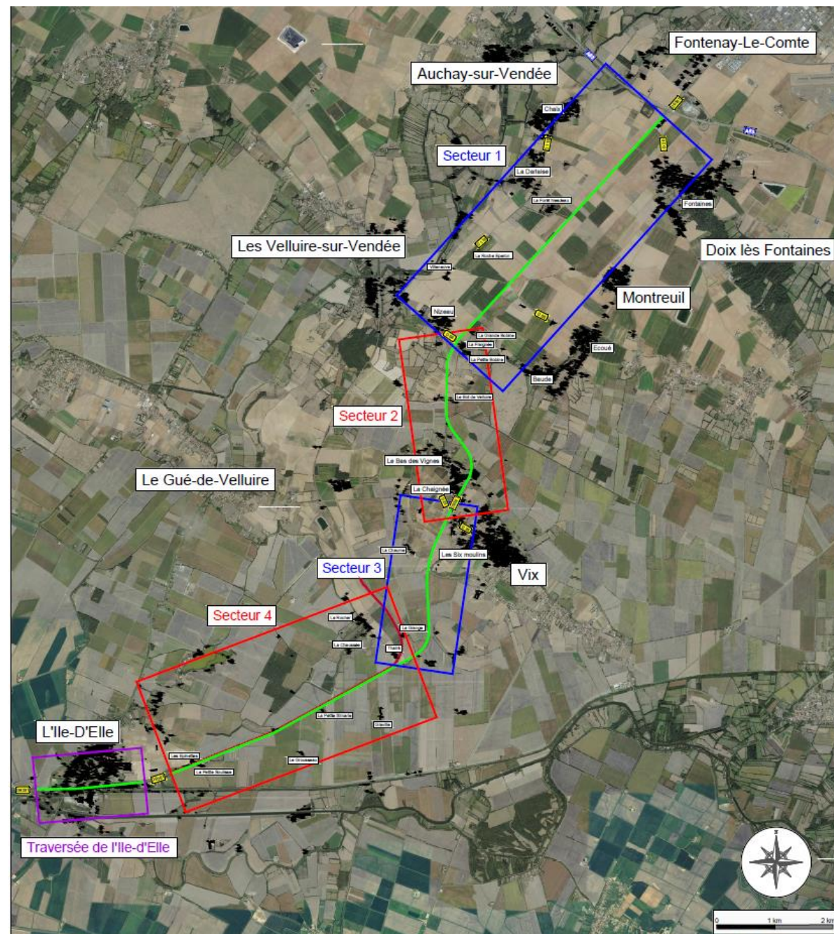
Figure 30 : Secteurs d'aménagement sur la RD938T (Source : IRIS Conseil)
