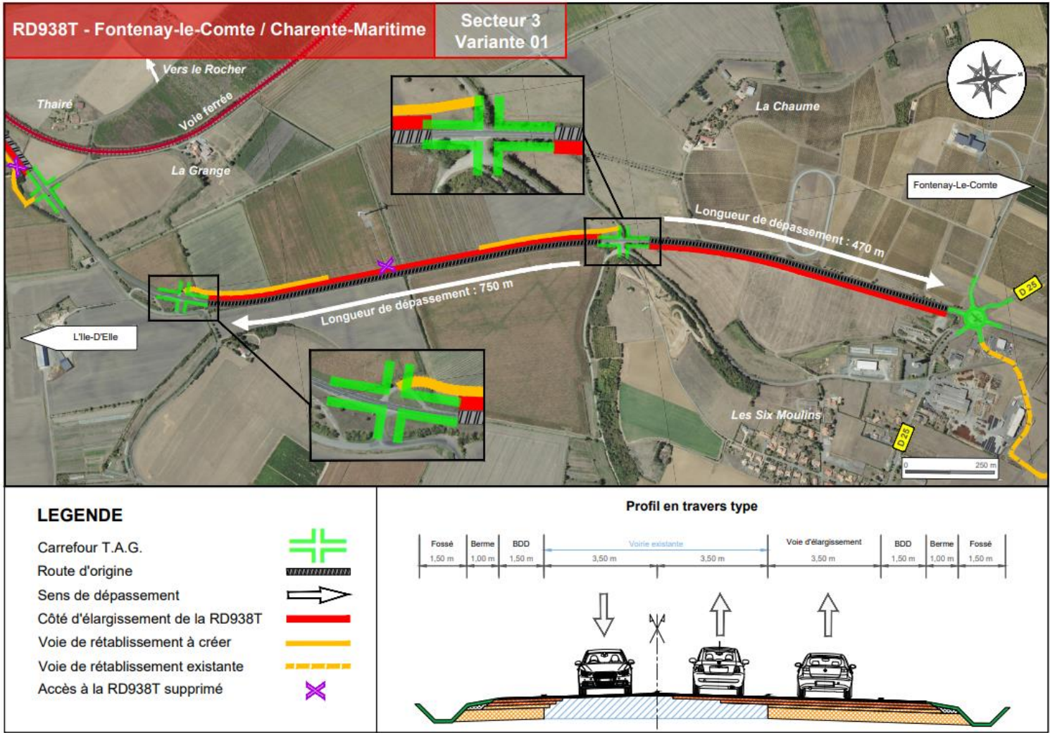
Figure 39 : Présentation de la variante 1 secteur 3 (Source : Concertation 2024, IRIS Conseil)
