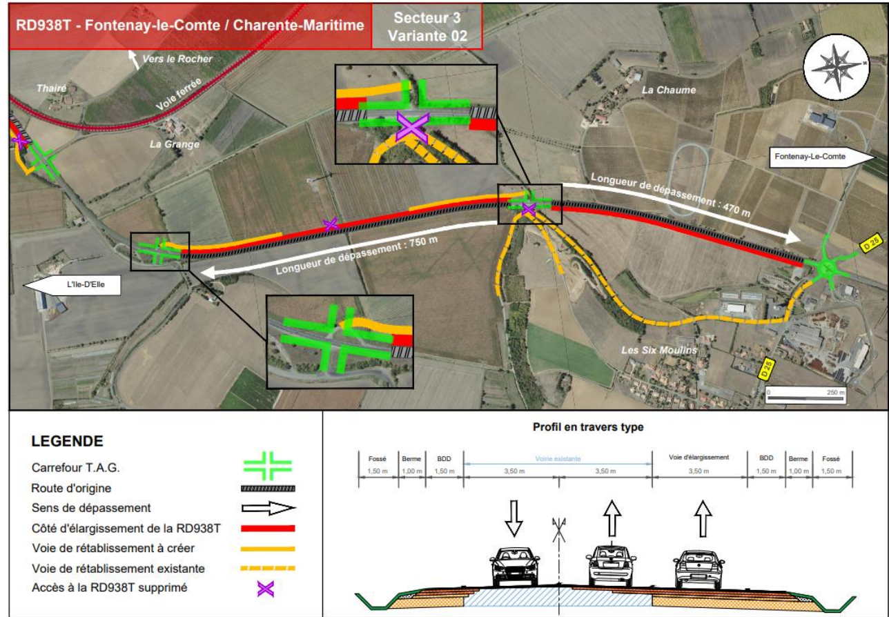
Figure 40 : Présentation de la variante 2 secteur 3 (Source : Concertation 2024, IRIS Conseil)
