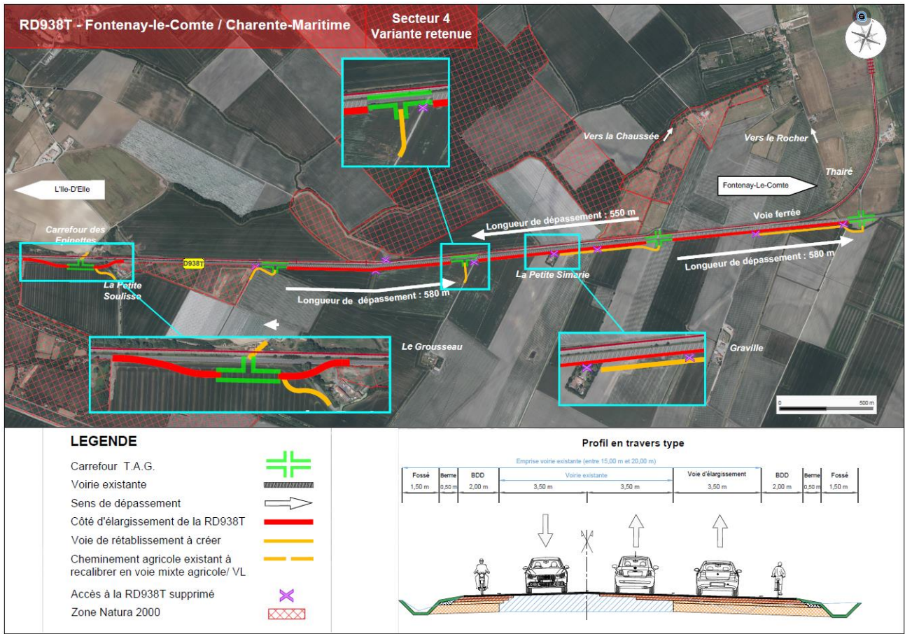
Figure 46 : Plan de la variante retenue sur le secteur 4
