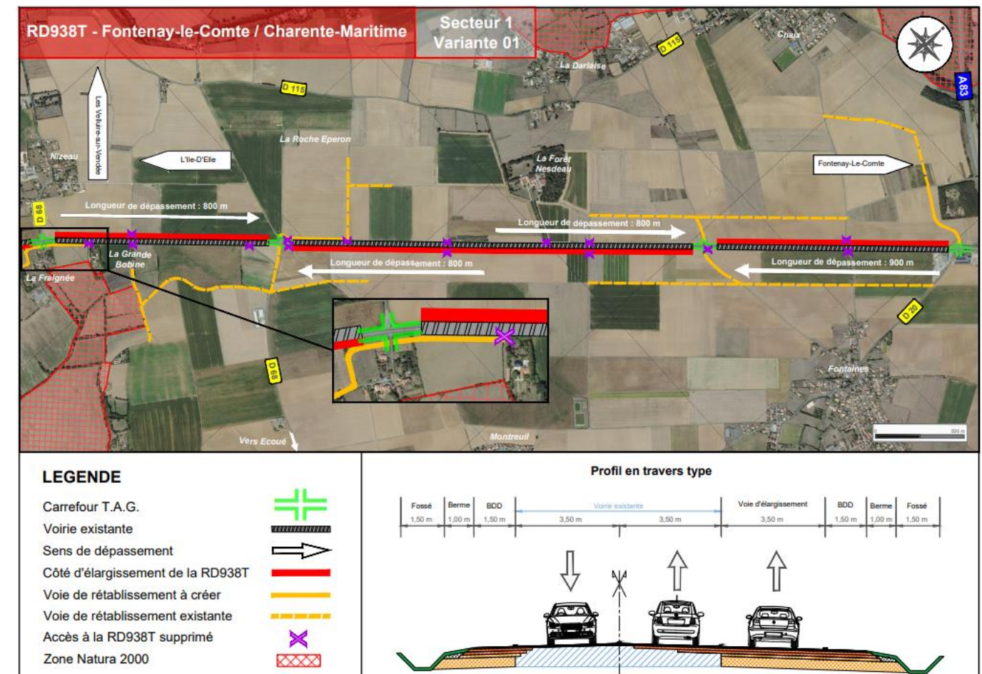
Figure 31 : Présentation de la variante 1 secteur 1 (Source : Concertation 2024, IRIS Conseil)
