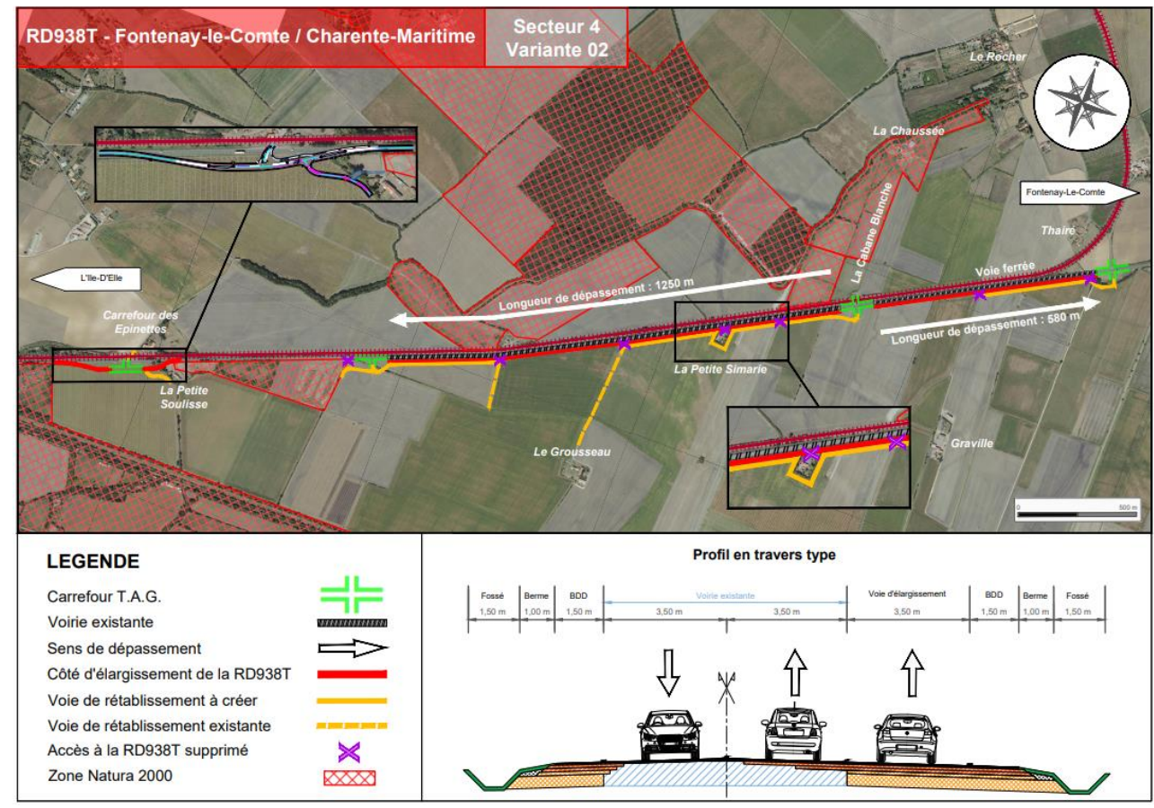
Figure 44 : Présentation de la variante 2 secteur 4 (Source : Concertation 2024, IRIS Conseil)
