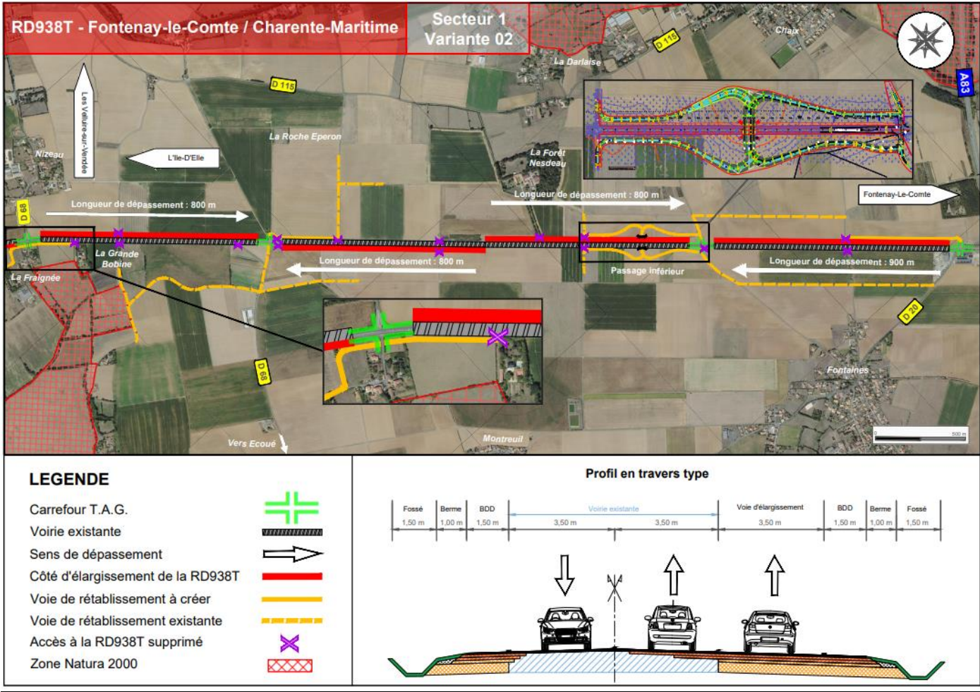
Figure 32 : Présentation de la variante 2 secteur 1 (Source : Concertation 2024, IRIS Conseil)
