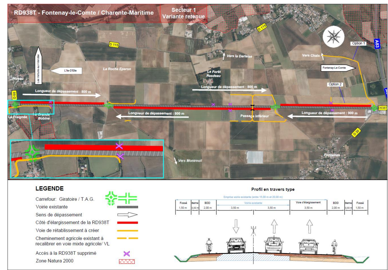
Figure 34 : Plan de la variante retenue sur le secteur 1
