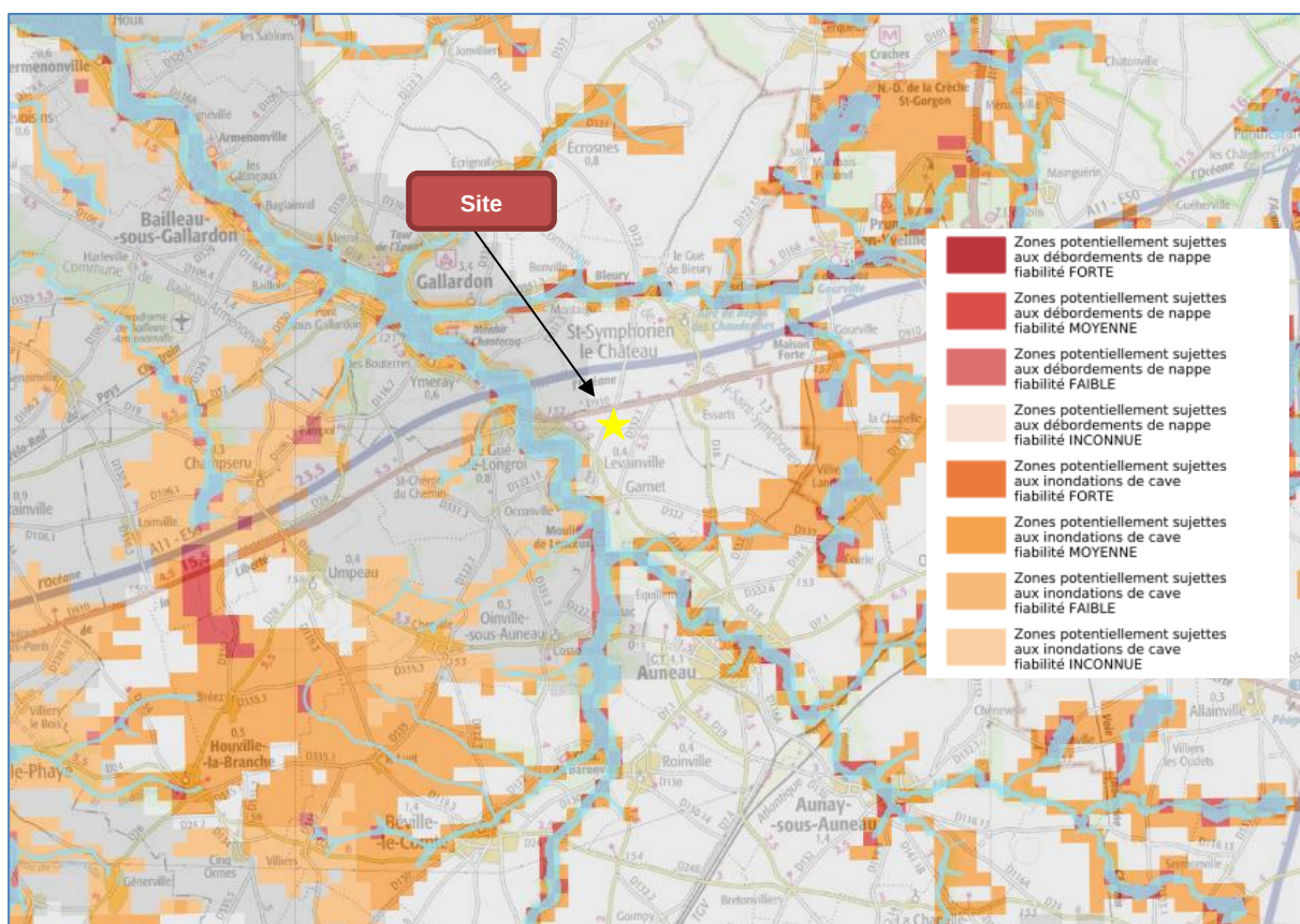
Figure 37 : Carte de sensibilité au phénomène de remontée de nappe
