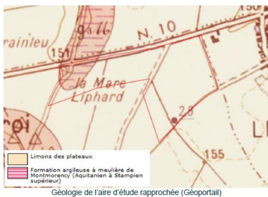
Géologie de l'aire d'étude rapprochée (Géoportail)
