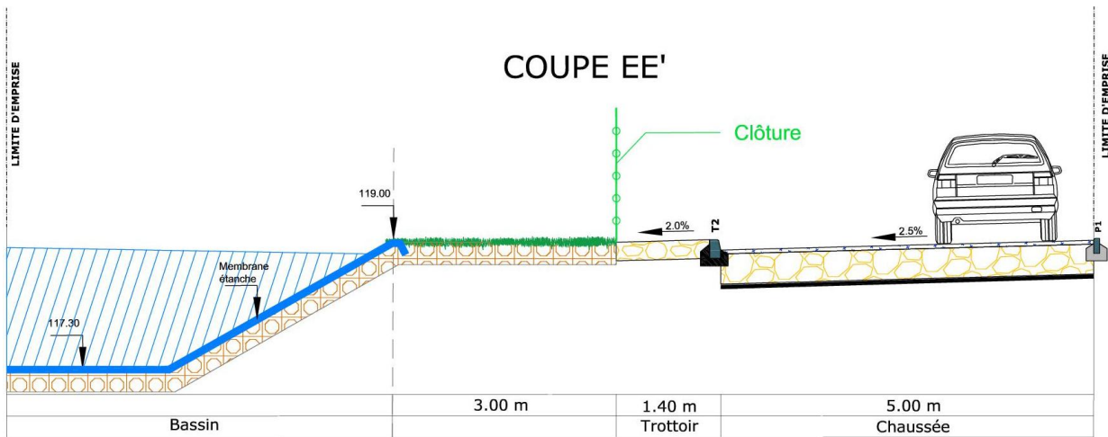
Coupe de principe reprise avec membrane étanche.
