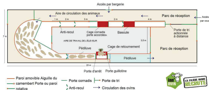
Parc de contention spécialisé brebis
