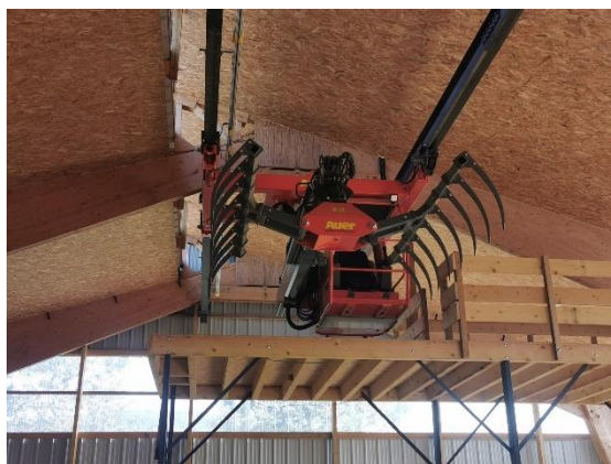
Figure 35 : Photo d'une griffe à fourrage qui permet la manutention du foin vrac à l'intérieur du bâtiment (Source : AS DEV.)
