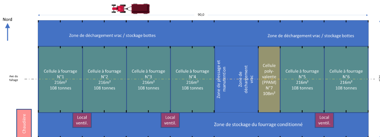
Figure 32 : Croquis général d'organisation du bâtiment de séchage et stockage du fourrage (vue de dessus) (Source : AS DEV.)
