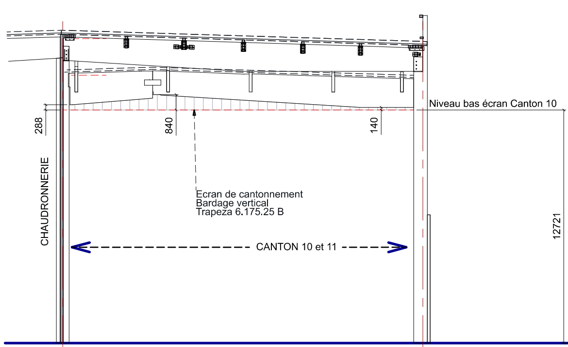
COUPE AXE 12
