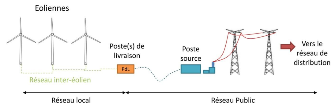
Figure 5 : Principe du raccordement électrique des installations
