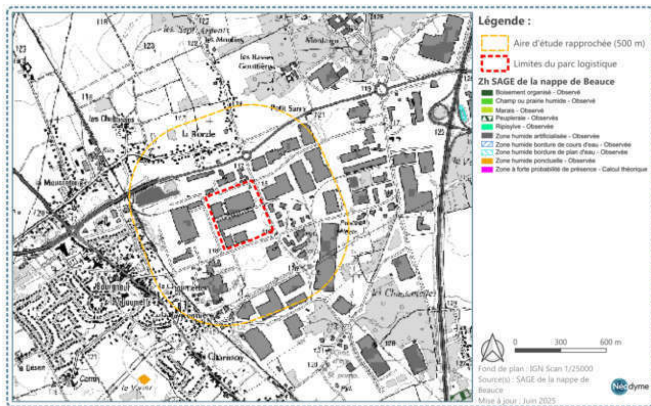
Figure 24 : Zones humides du SAGE de la nappe de Beauce et de ses milieux aquatiques associés
