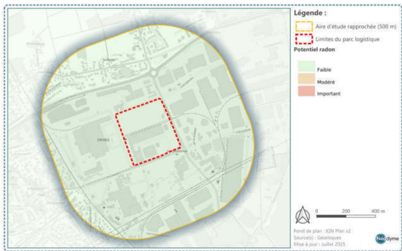
Figure 79 : Potentiel radon à l'échelle de l'aire d'étude rapprochée
