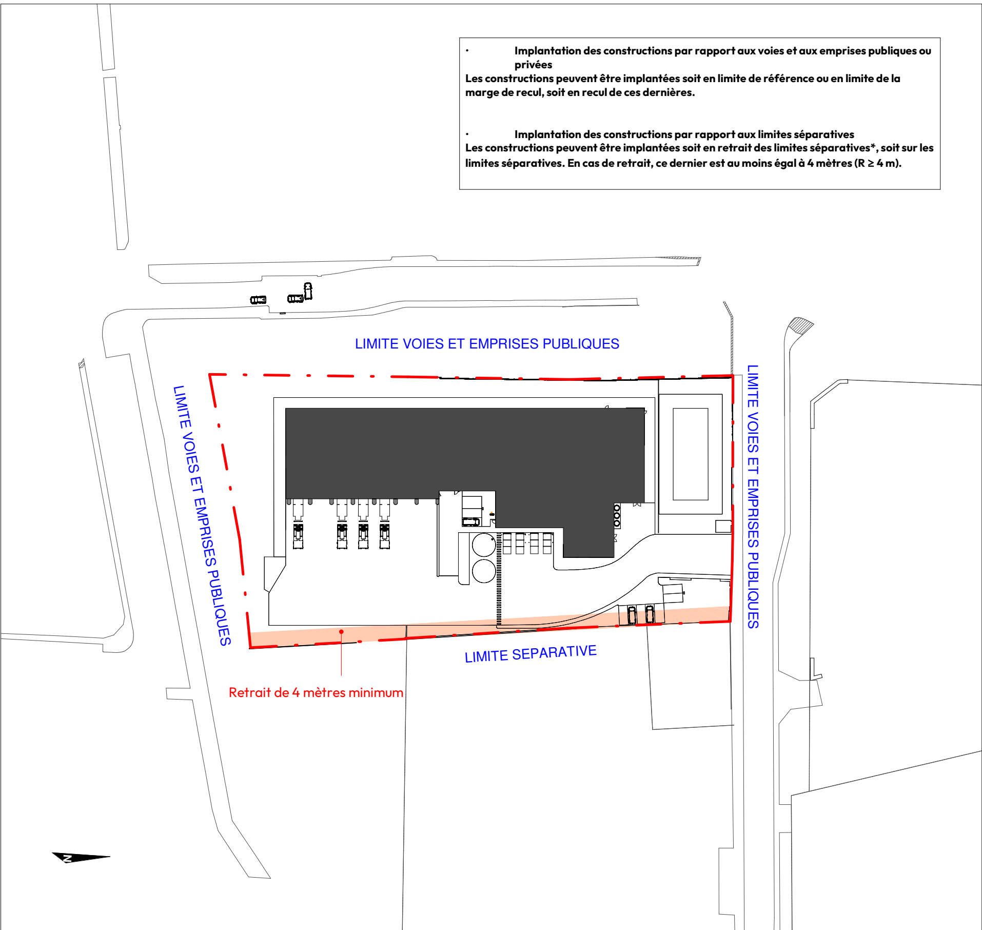
Plan de masse - PLU Ech. 1 : 1000
