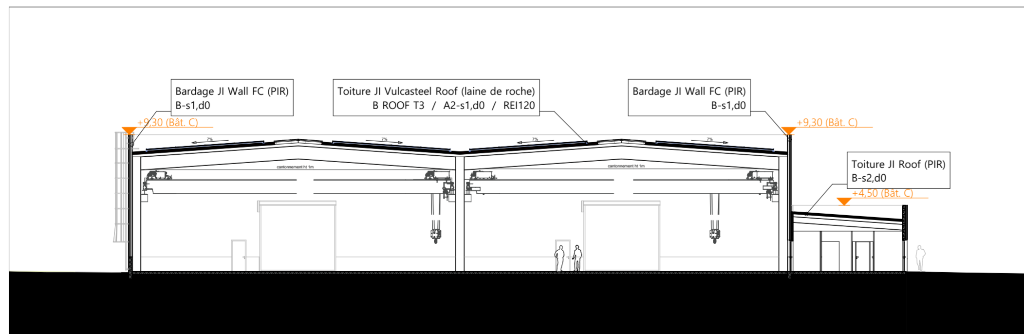
PROJET Coupe C1 1:250
