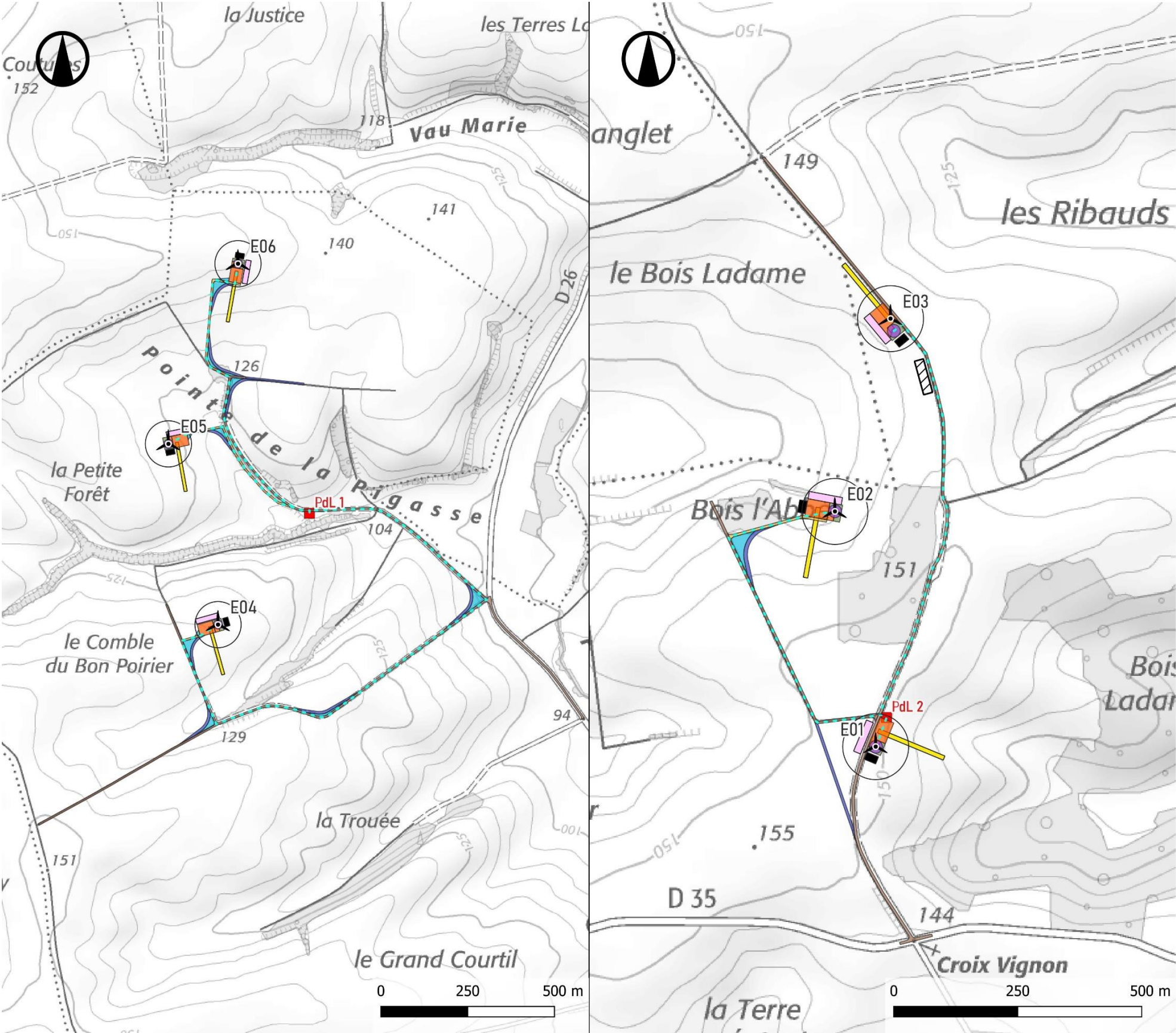
Carte 13 : Présentation de l'installation
