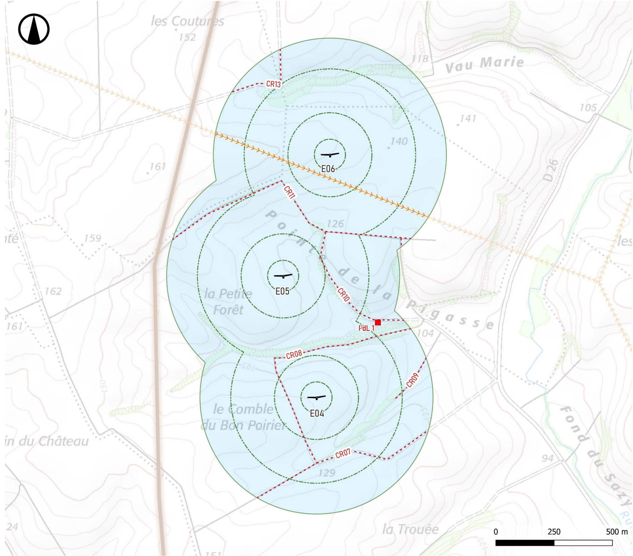
Carte 11 : Enjeux humains et matériels - partie nord
