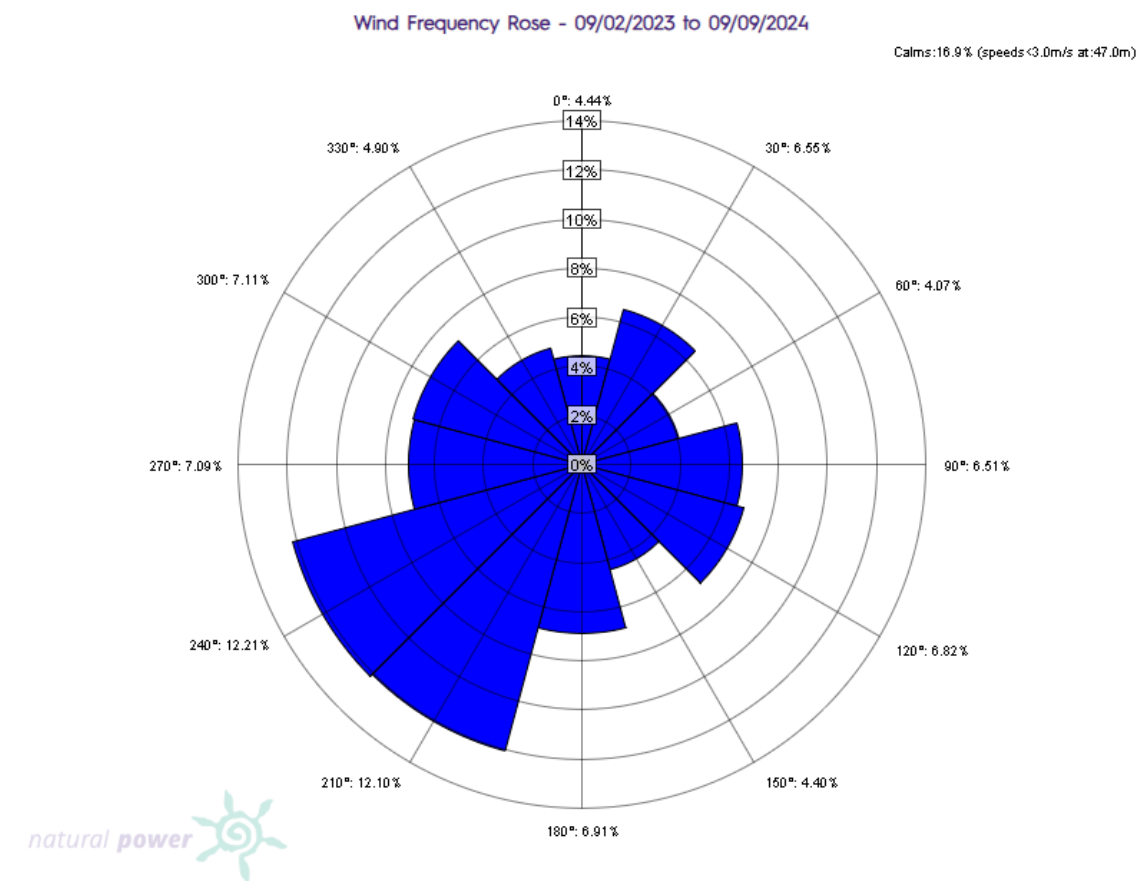
Figure 1 : Rose des vents (source : TTR Energy et ELEMENTS, 2024) ► Le périmètre d’étude de dangers est soumis à un climat océanique dégradé. ► La vitesse des vents et la densité d’énergie observées au niveau du périmètre d’étude de dangers définissent aujourd’hui ce dernier comme assez bien venté.
