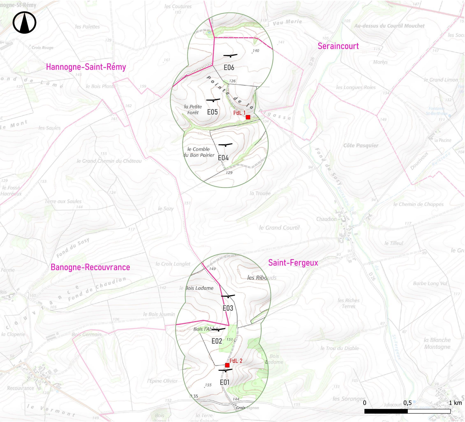
Carte 2 : Périmètre de l'étude de dangers
