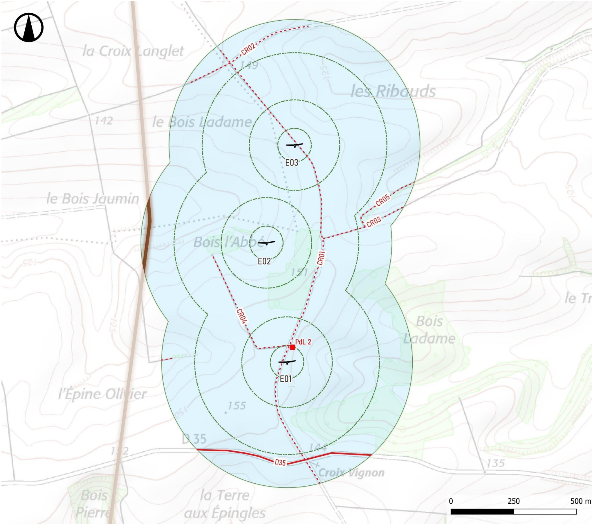
Carte 12 : Enjeux humains et matériels - partie sud
