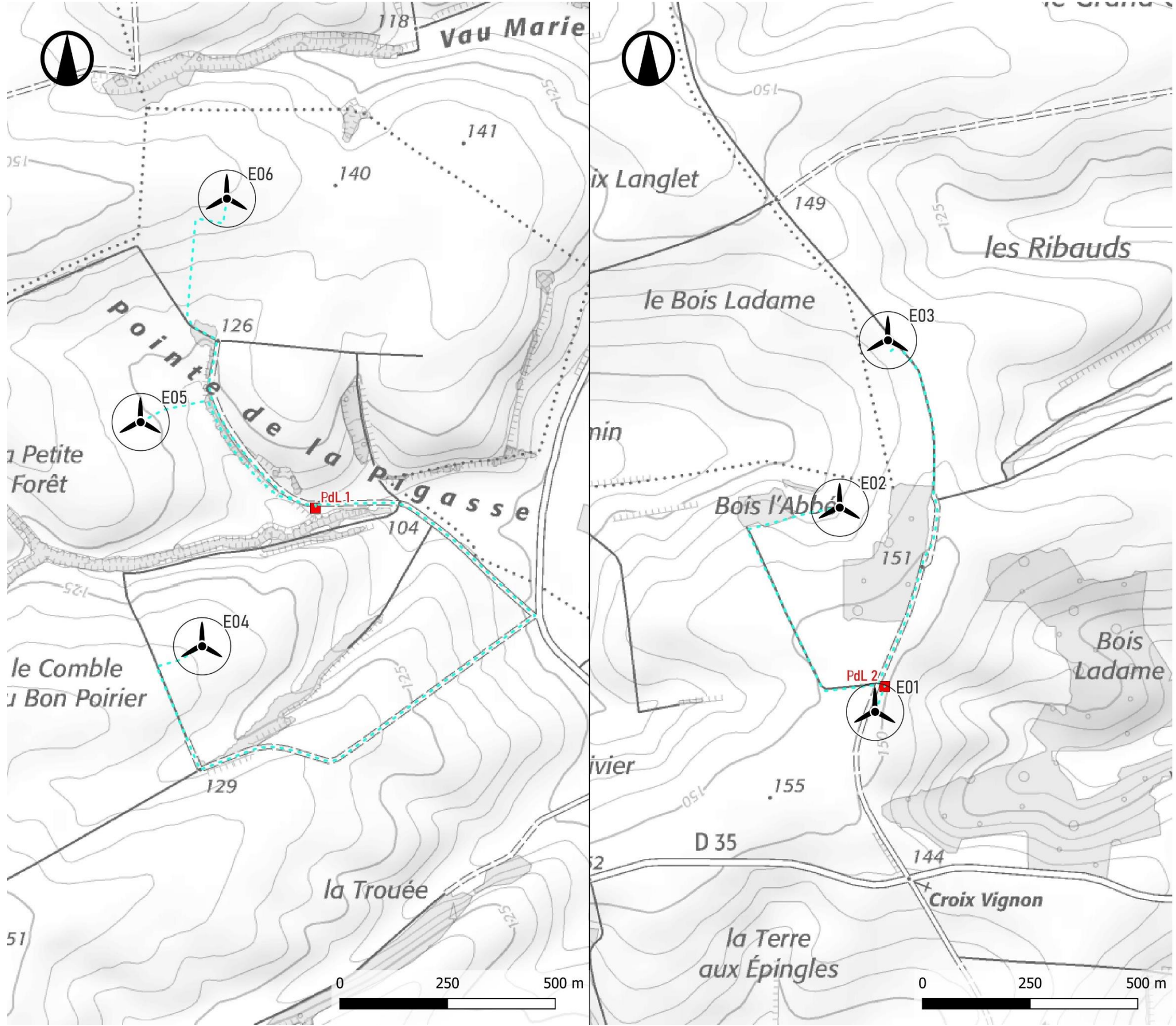
Carte 14 : Raccordement inter-éolien
