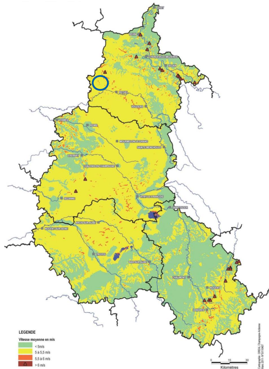
Carte 5 : Vitesse des vents dans l’ancienne région Champagne-Ardenne – Cercle bleu : Périmètre d’étude de dangers (source : Schéma Régional Eolien, 2012)
