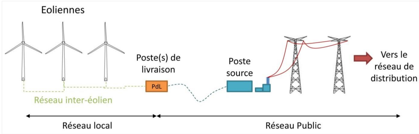
Figure 9 : Raccordement électrique des installations avec l'option HTA
