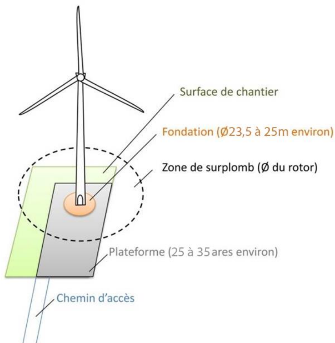
Figure 6 : Schéma illustratif de l'emprise au sol d'une éolienne (Source : Vestas)
