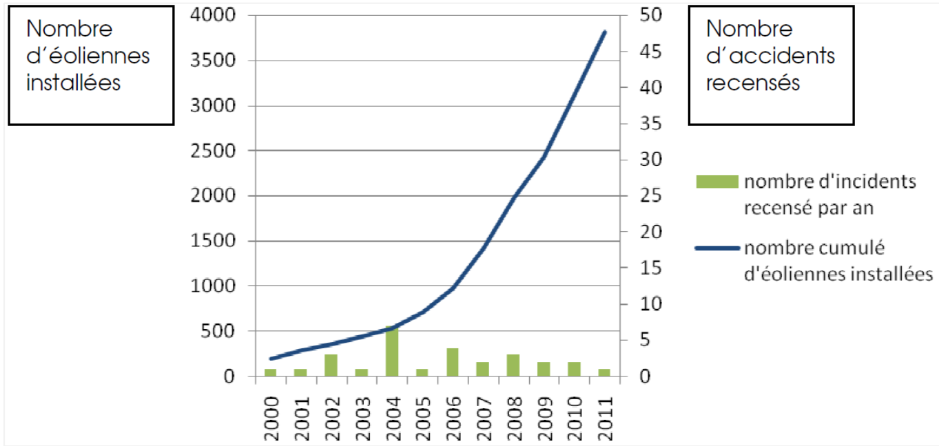
Figure 2 : Nombre d'incidents en rapport avec la puissance éolienne installée en France
