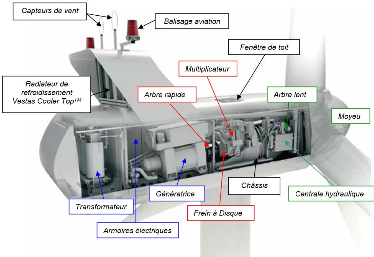
Figure 7 : Exemple de schéma illustrant les composants de la nacelle (Source : Vestas)
