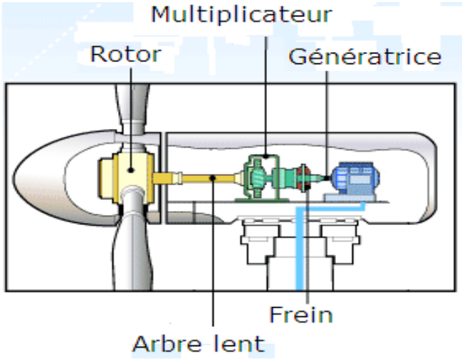
Figure 8 : Schéma simplifié de la chaîne cinématique (Source : Vestas)
