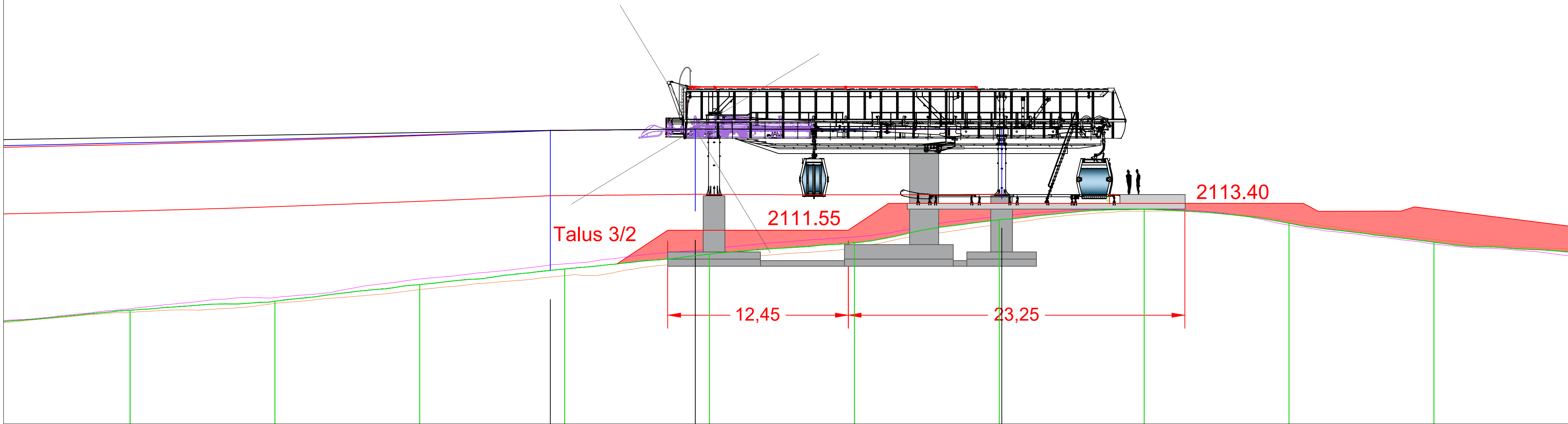
Coupe sur gare amont Echelle : 1/200
