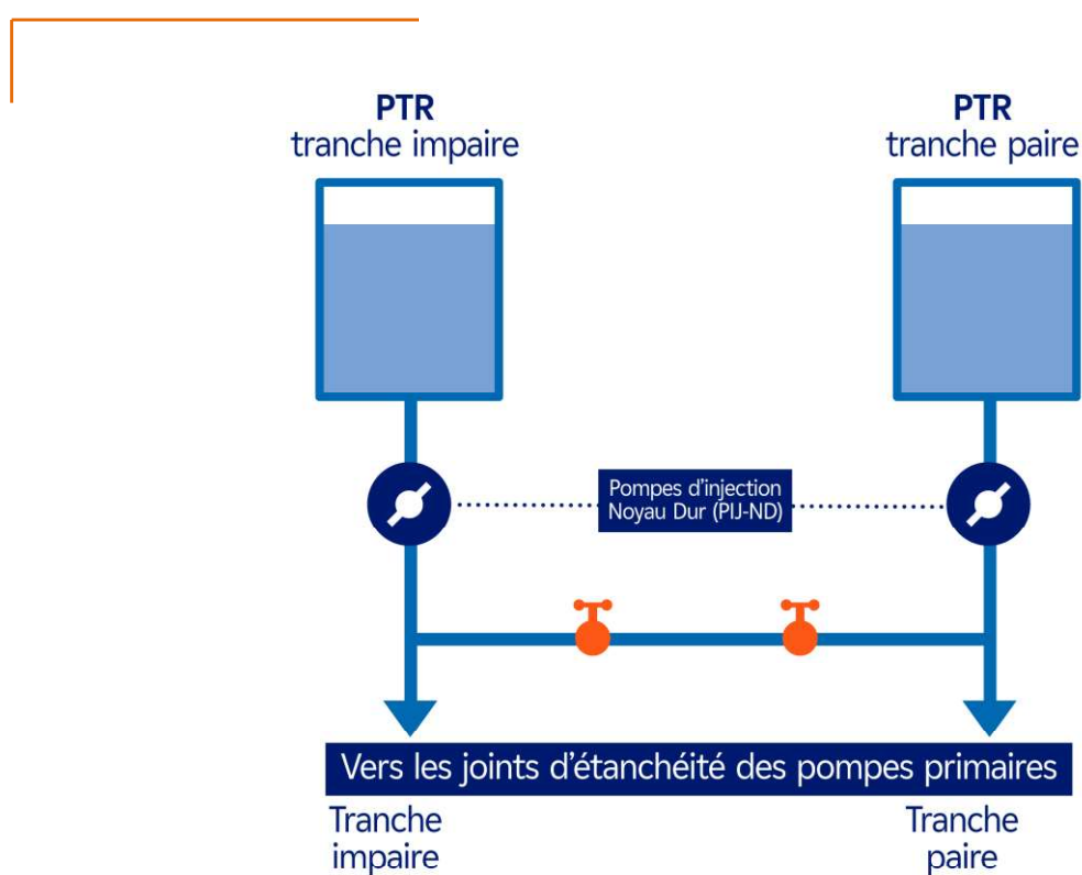
Figure 18. Configuration avec pompes d'injection aux joints « Noyau Dur » (PIJ-ND)
