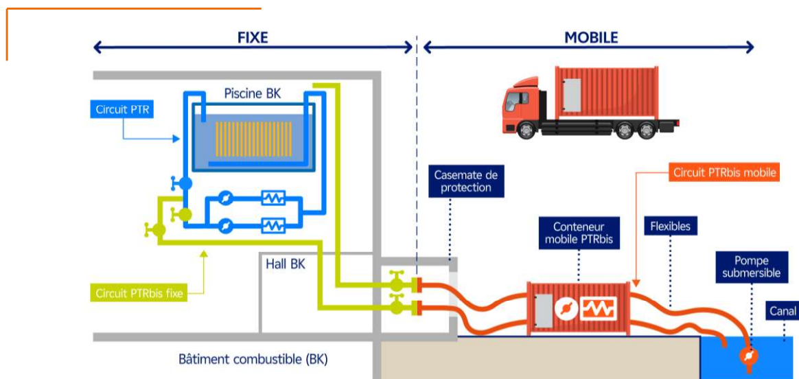
Figure 19. Appoint Noyau Dur par le haut de la piscine d'entreposage du combustible (représenté par la tuyauterie verte sur le schéma à droite de la piscine d'entreposage du combustible)
