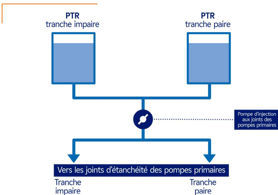
Figure 17. Configuration avant l'installation de la pompe d'injection aux joints « Noyau Dur » (PIJ-ND)
