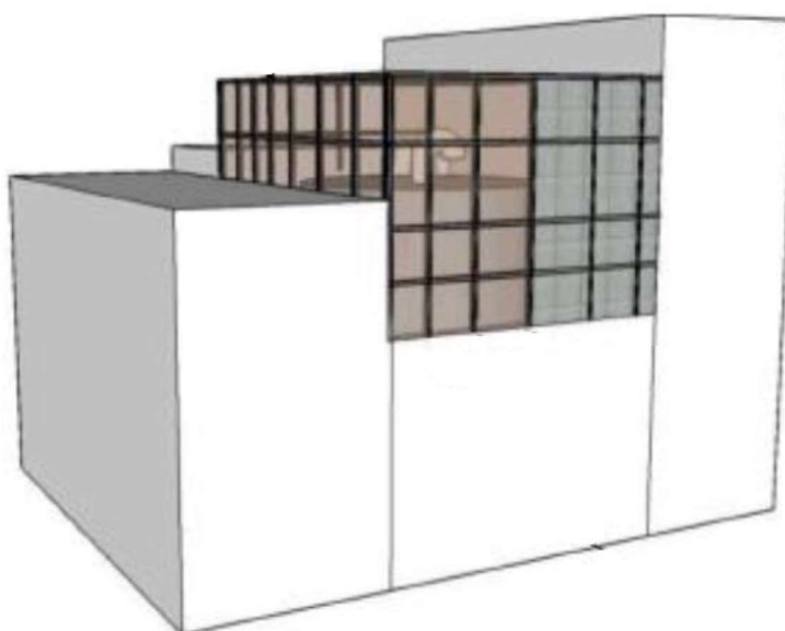
Figure 20. Protection contre la tornade « Noyau Dur » : photo de l'installation actuelle – exemple du réacteur n° 1 de la centrale de Chinon – et illustration de la disposition proposée, de type « grilles renforcées », autour de la bâche PTR cylindrique.
