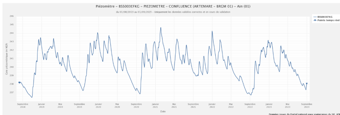
Figure 16 : Niveau de la nappe par le piézomètre Confluence de Valromey sur Séran
