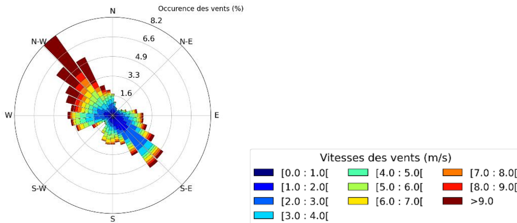
Figure 5 : Rose des vents 2022 – 2024 – Station Météo France de Marignane
