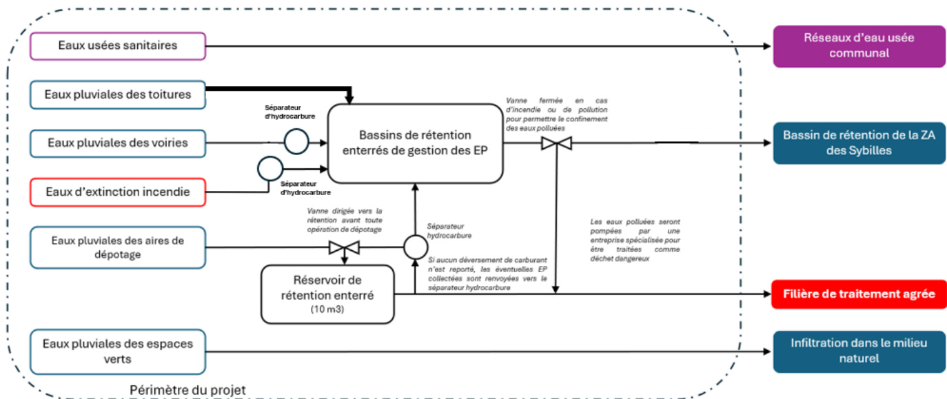
Figure 3 : Schéma de gestion des eaux
