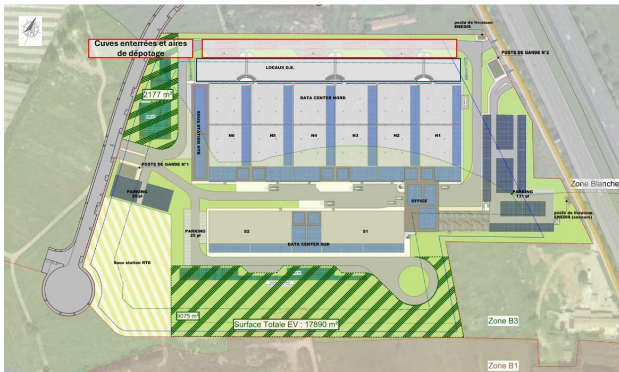
Figure 2 : Localisation des groupes électrogènes et des cuves de HVO enterrées
