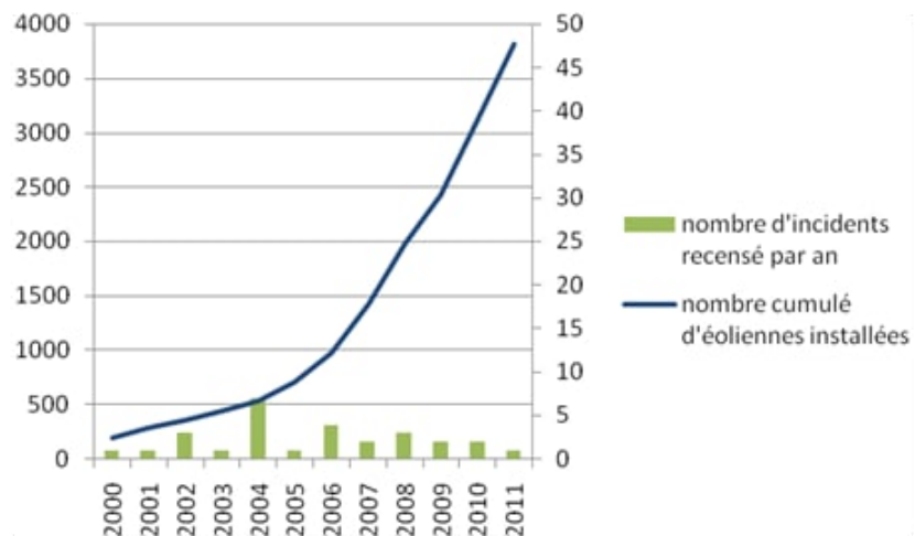
Figure 27 : Evolution du nombre d'incidents annuels en France et du nombre d'éoliennes installées
