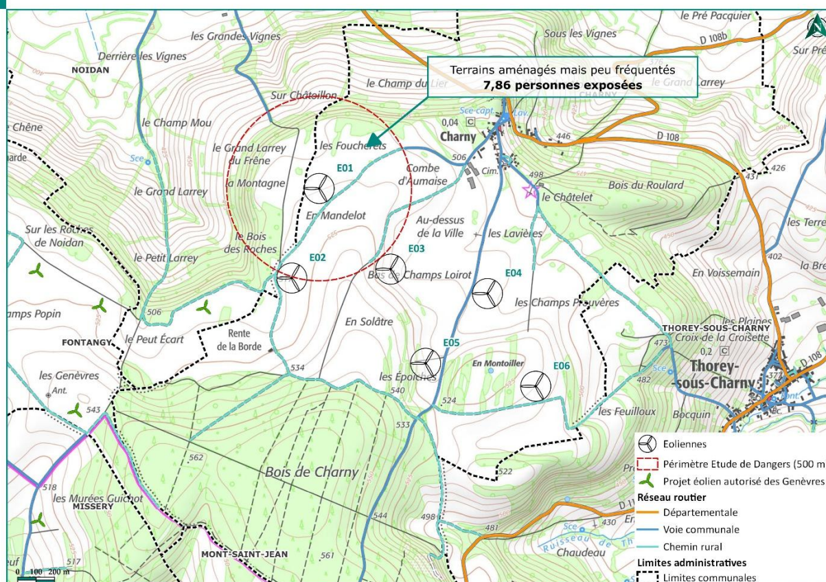
Carte 16 : Synthèse des cibles et du nombre de personnes exposées pour l'éoliennes E01
