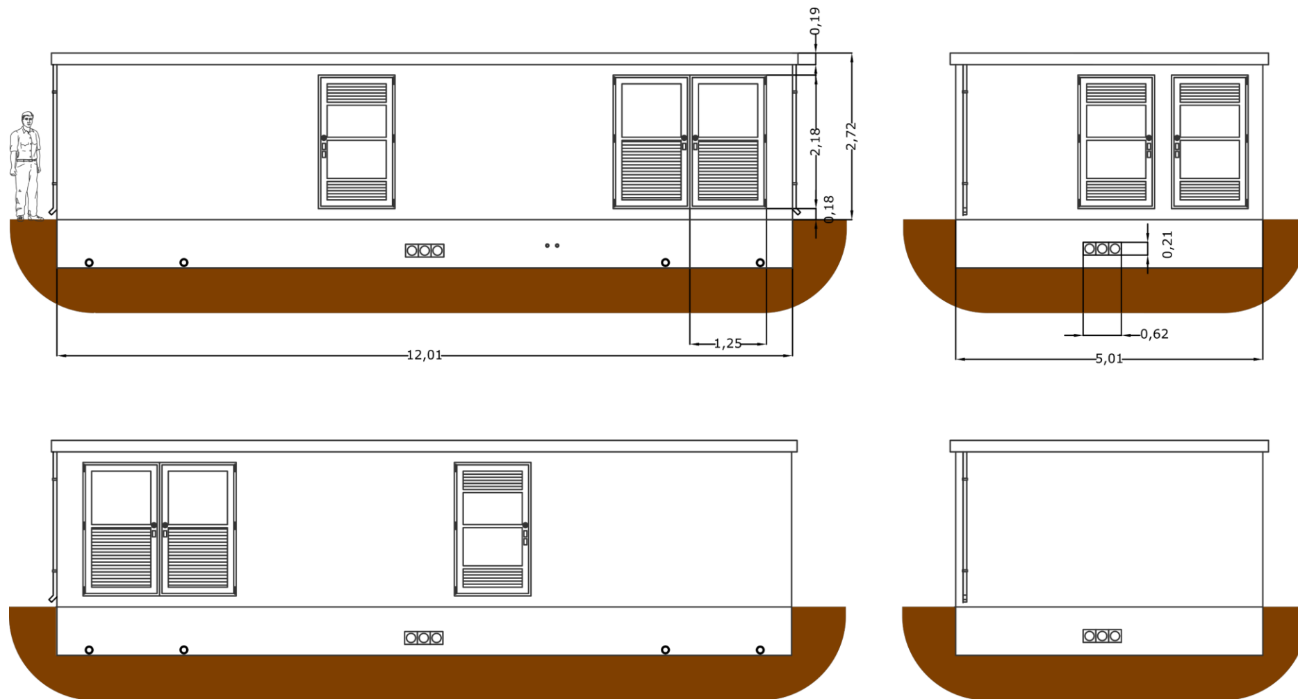
Figure 15 : Schéma d'un poste de livraison
