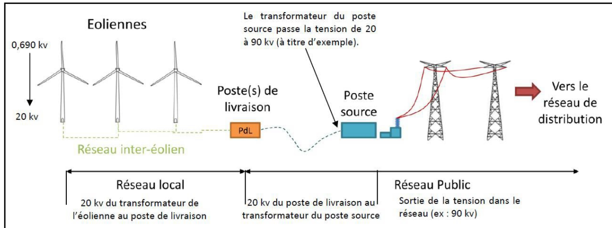
Figure 13 : Schéma de raccordement électrique d'un parc éolien
