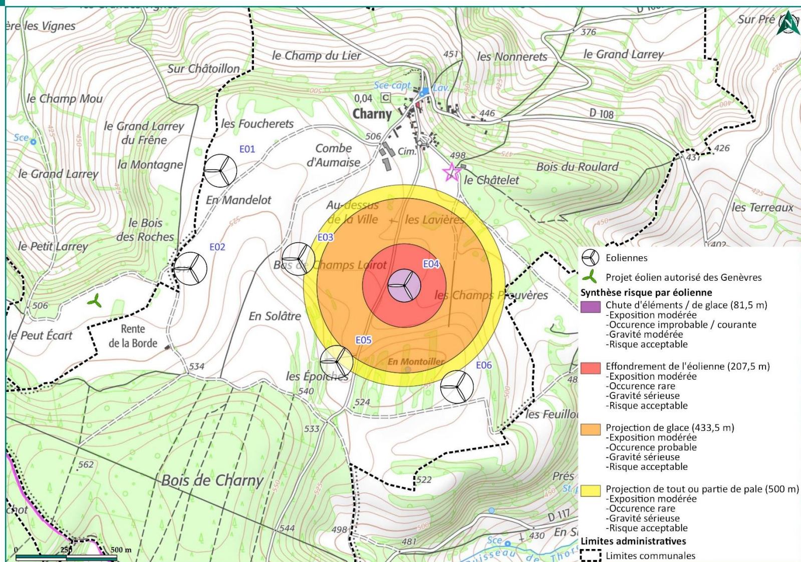
Carte 30 : Synthèse des risques pour l'éolienne E04
