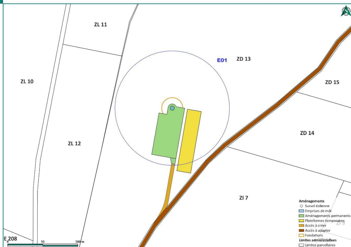
Figure 7 : Aires de montage et d'entretien de l'éolienne E01
