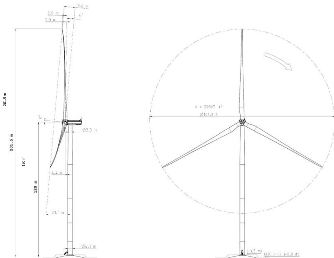
Figure 5 : Dessin d'élévation de l'éolienne Nordex N163- 5,9 MW avec une hauteur de moyeu de 120 m
