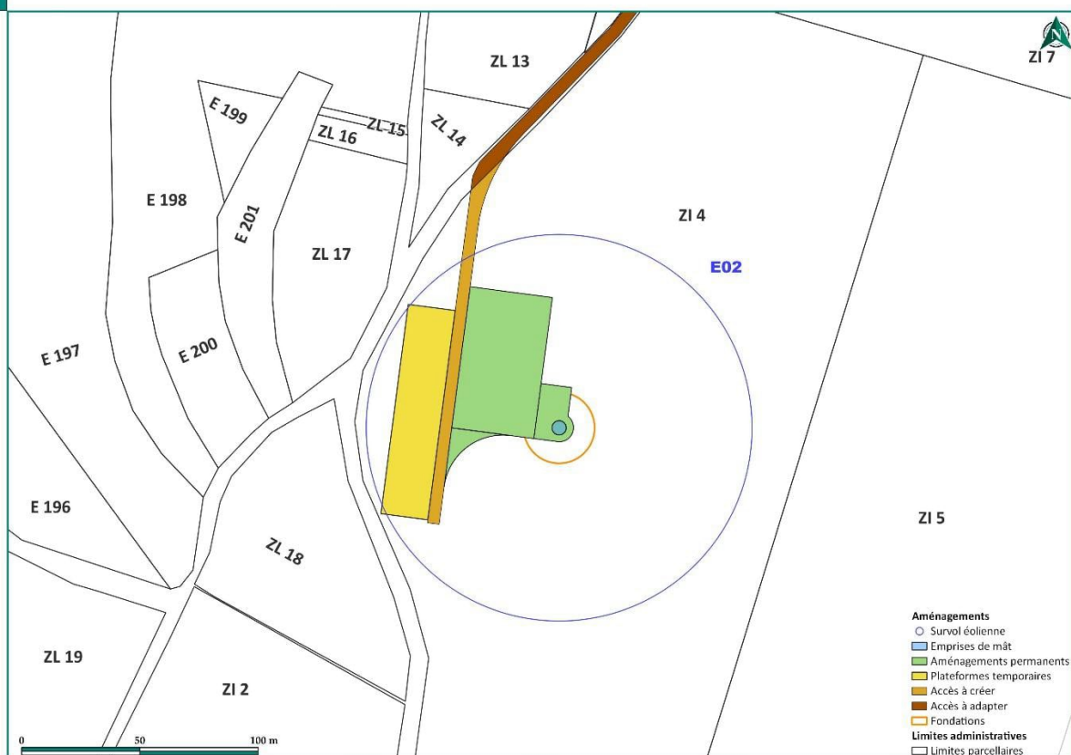
Figure 8 : Aires de montage et d'entretien de l'éolienne E02
