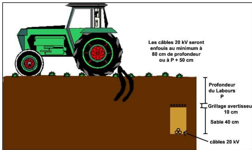
Figure 14 : Exemple de tranchées sous champs labouré
