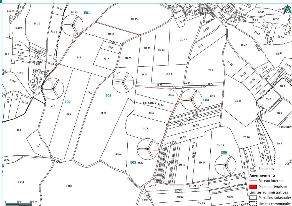
Carte 24 : Localisation du poste de livraison et réseau interne du parc éolien
