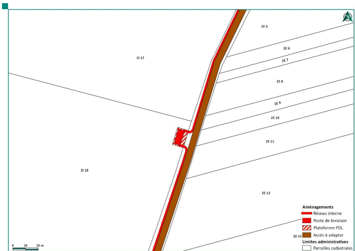
Carte 25 : Plan d'installation du poste de livraison
