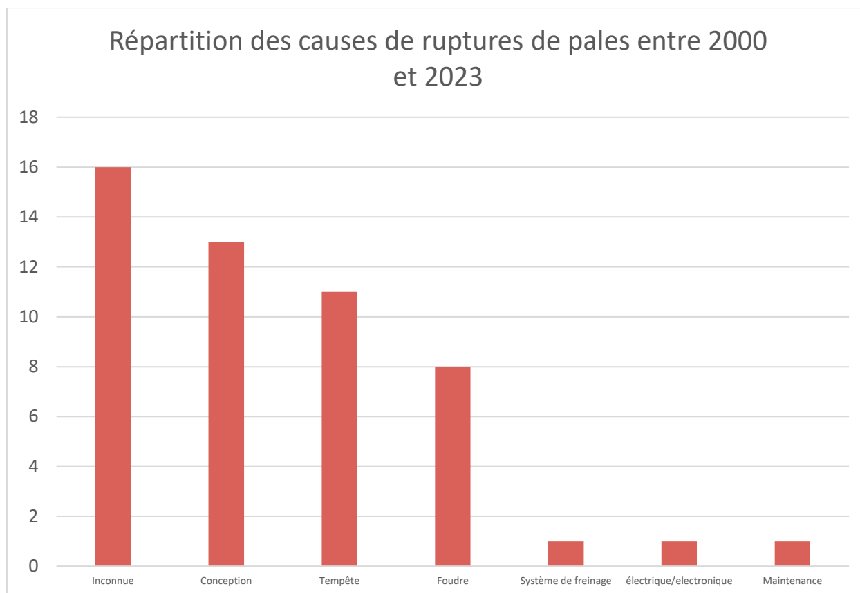
Figure 22 : Répartition des causes de ruptures de pales en France
