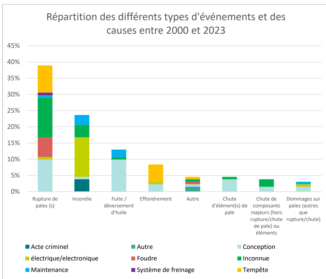
Figure 19 : Répartition des événements accidentels en France
