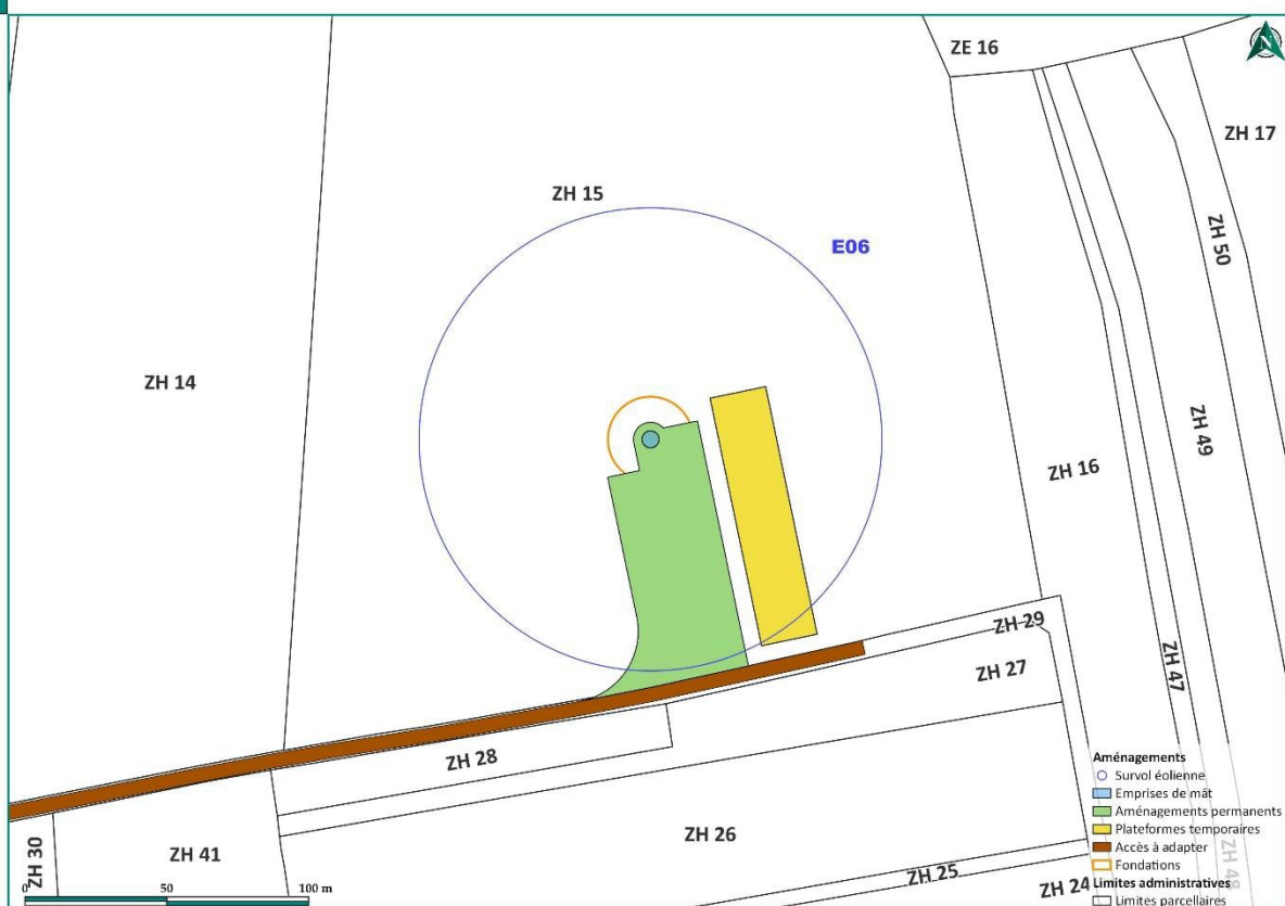
Figure 12 : Aires de montage et d'entretien de l'éolienne E06
