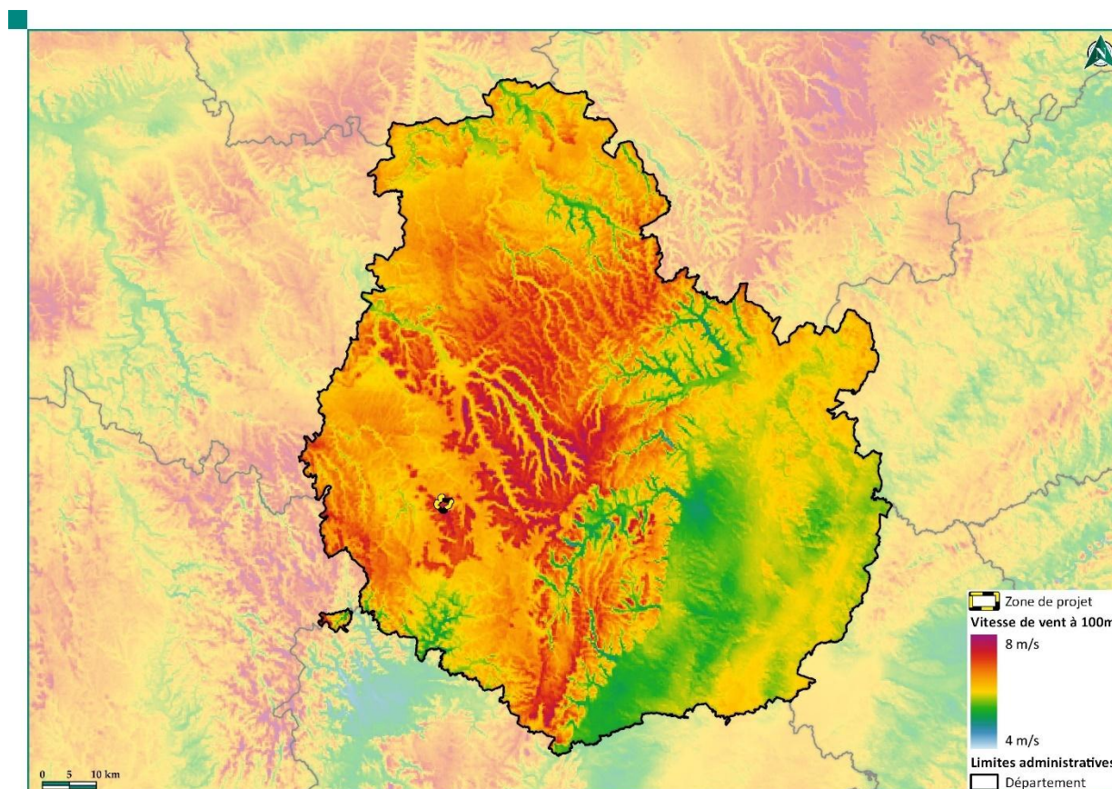
Carte 5 : Vitesse de vent moyen à 100 m dans la Côte-d'Or
