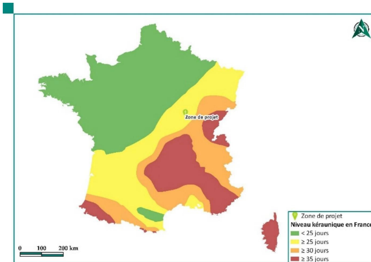
Carte 6 : Carte de France du niveau kéraunique
