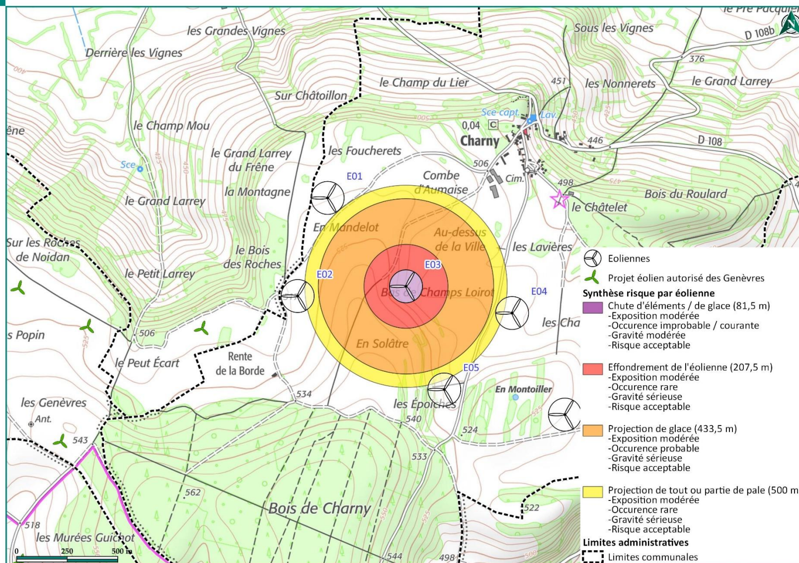
Carte 29 : Synthèse des risques pour l'éolienne E03
