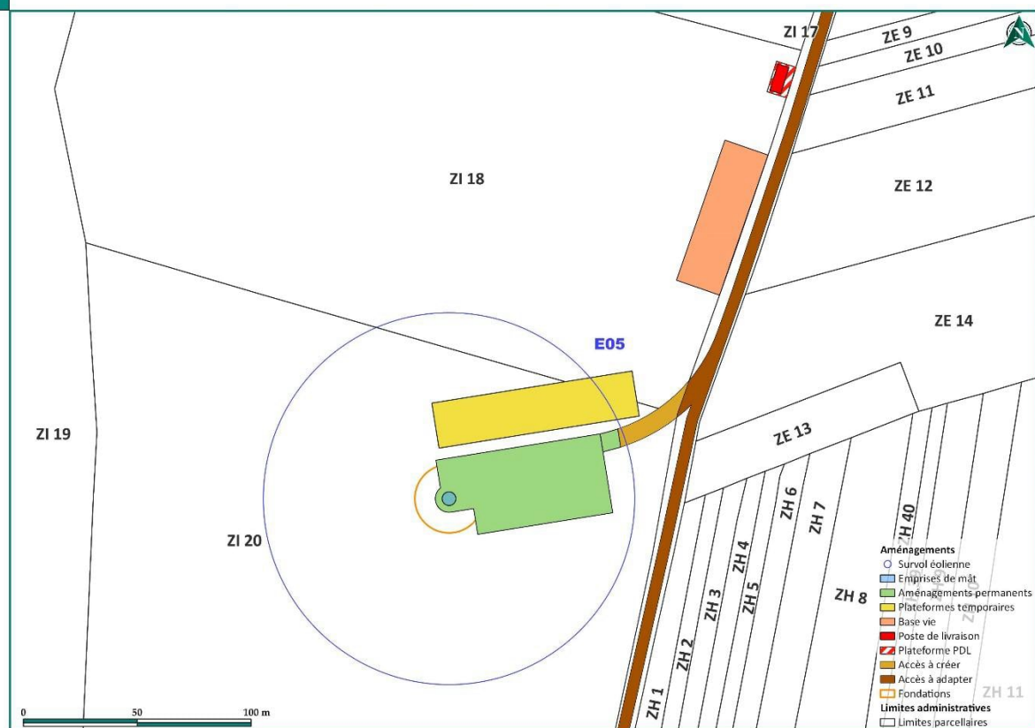
Figure 11 : Aires de montage et d'entretien de l'éolienne E05
