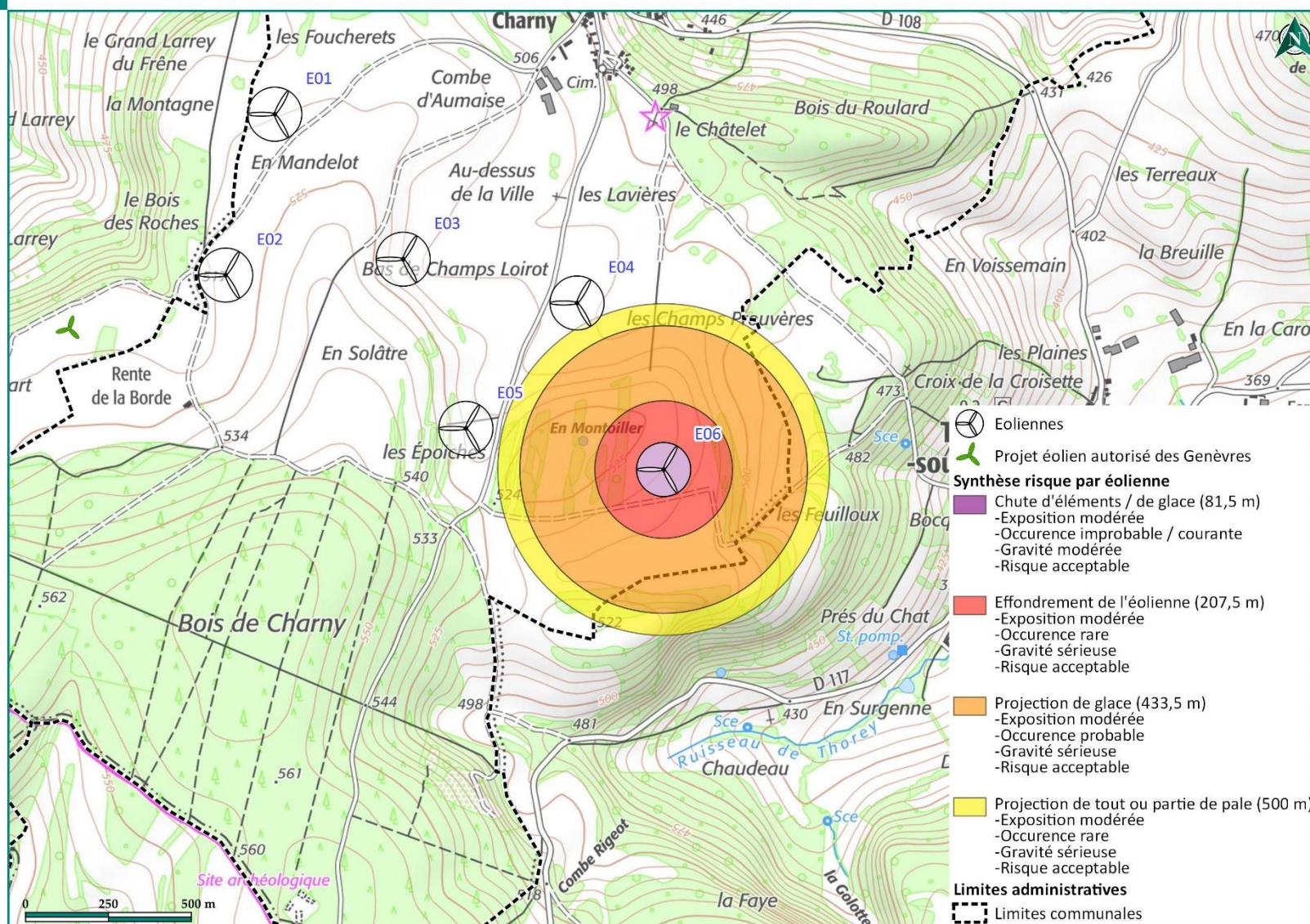
Carte 32 : Synthèse des risques pour l'éolienne E06
