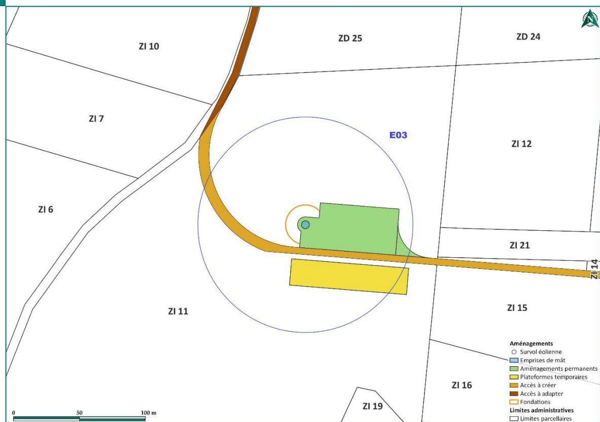
Figure 9 : Aires de montage et d'entretien de l'éolienne E03
