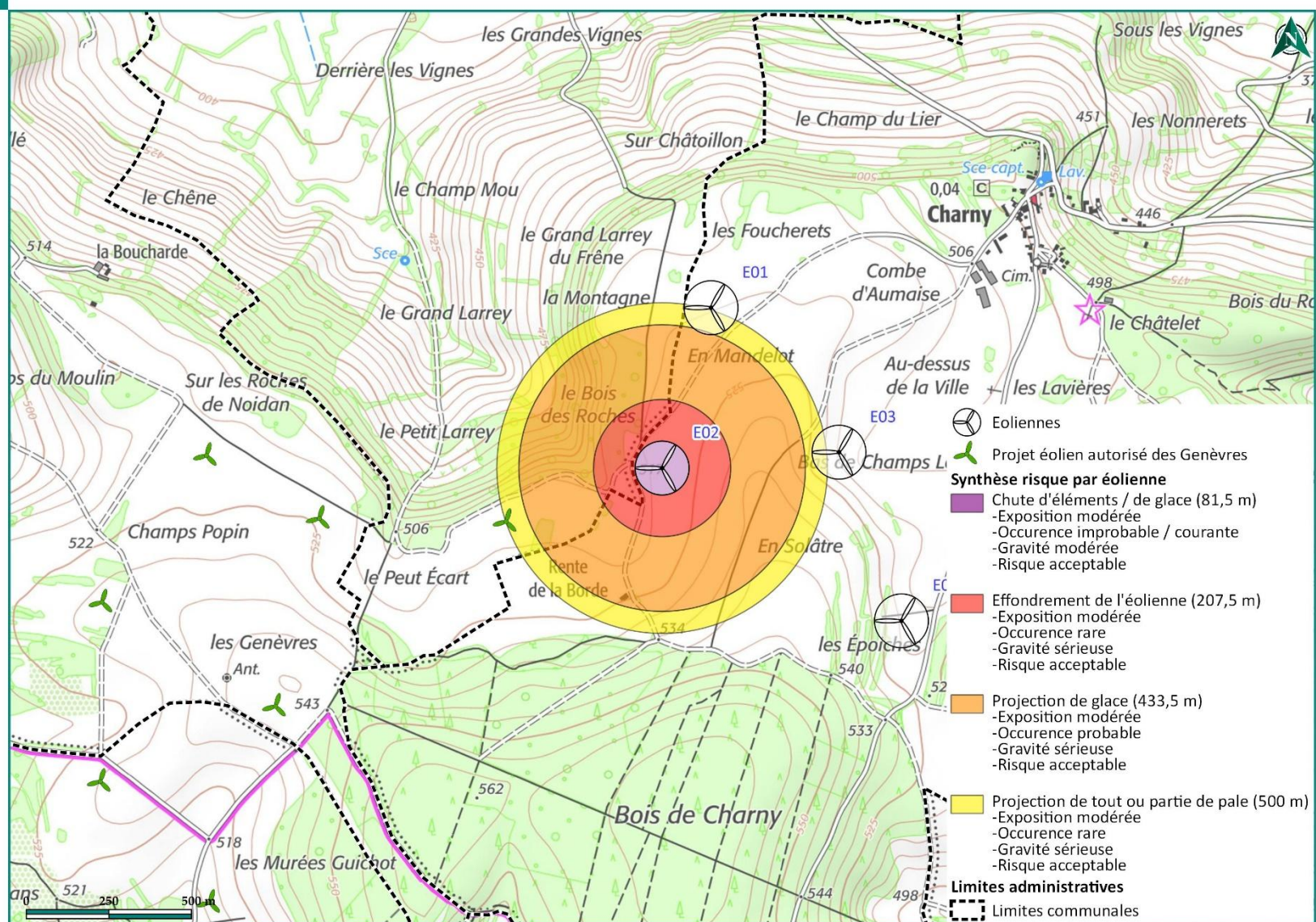
Carte 28 : Synthèse des risques pour l'éolienne E02
