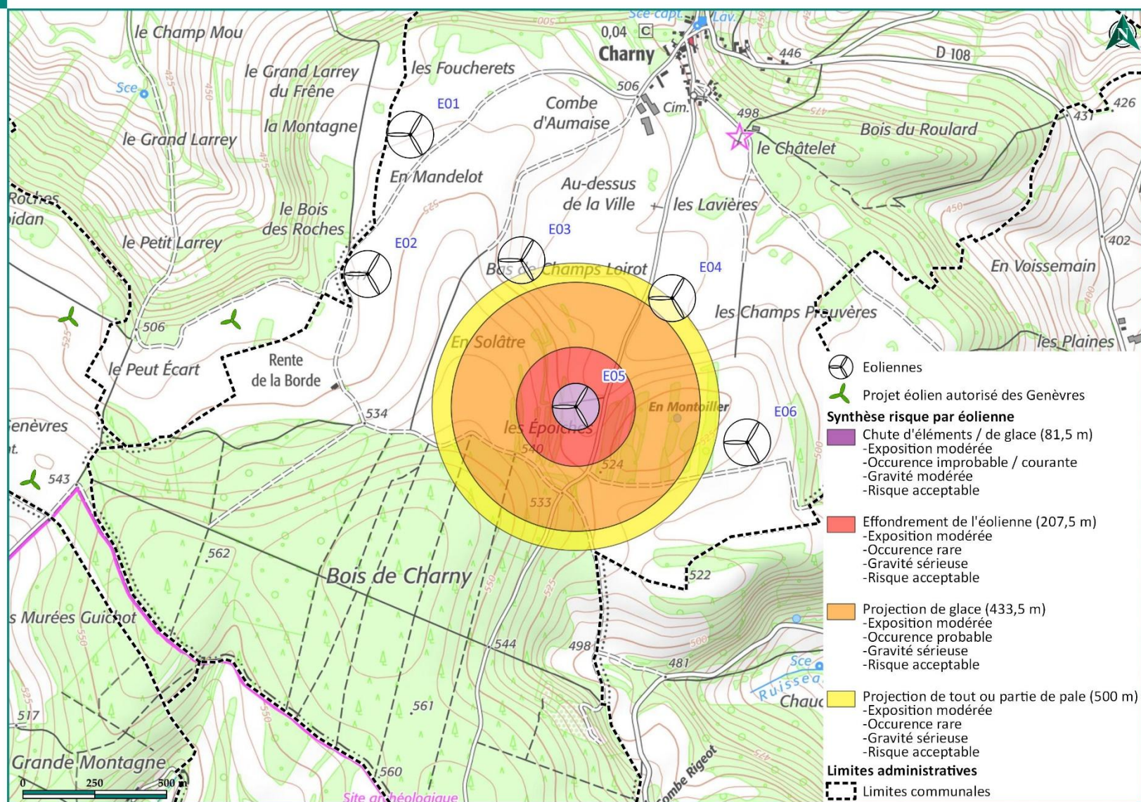
Carte 31 : Synthèse des risques pour l'éolienne E05
