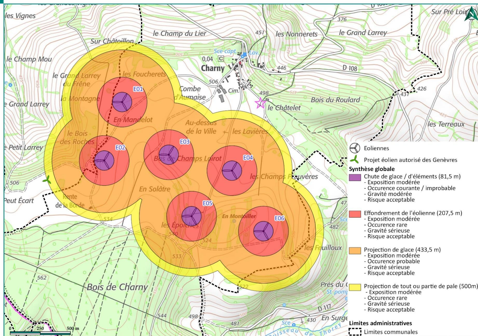
Carte 26 : Synthèse des risques
