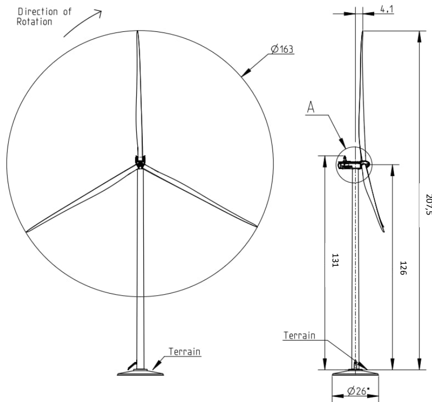
Figure 4 : Dessin d'élévation de l'éolienne Vestas V163- 4,5 MW avec une hauteur de moyeu de 126 m
