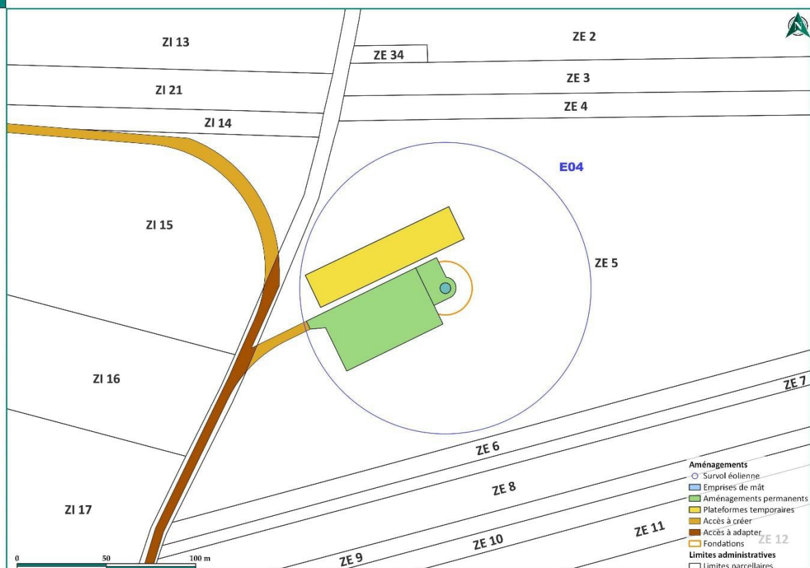
Figure 10 : Aires de montage et d'entretien de l'éolienne E04
