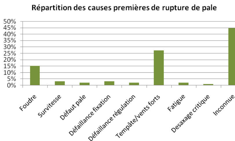
Figure 25 : Répartition des causes premières de rupture de pale
