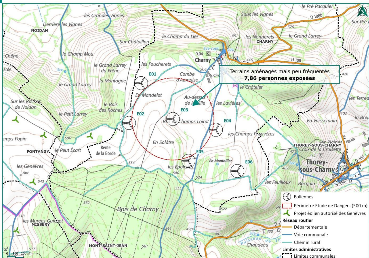
Carte 18 : Synthèse des cibles et du nombre de personnes exposées pour l'éoliennes E03
