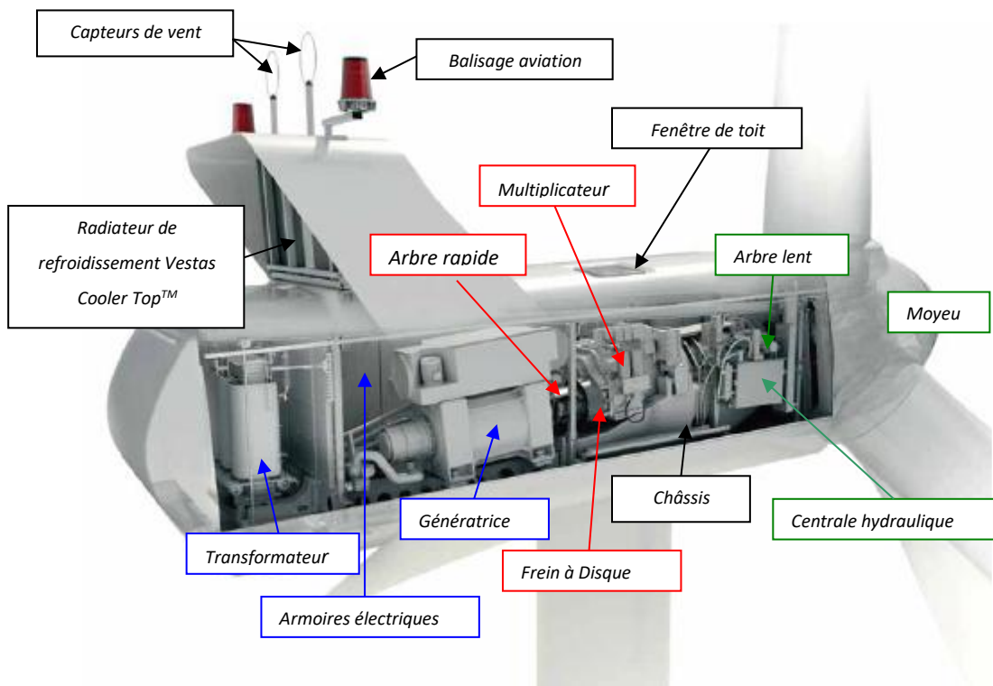
Figure 3 : Exemple de schéma technique (nacelle Vestas V136 - 4,2 MW)
