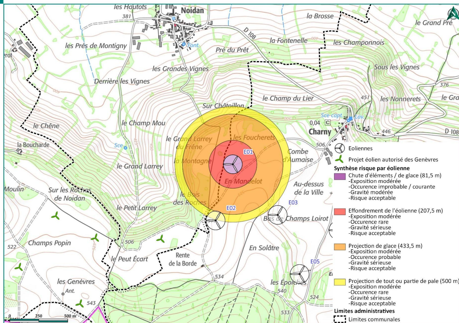
Carte 27 : Synthèse des risques pour l'éolienne E01
