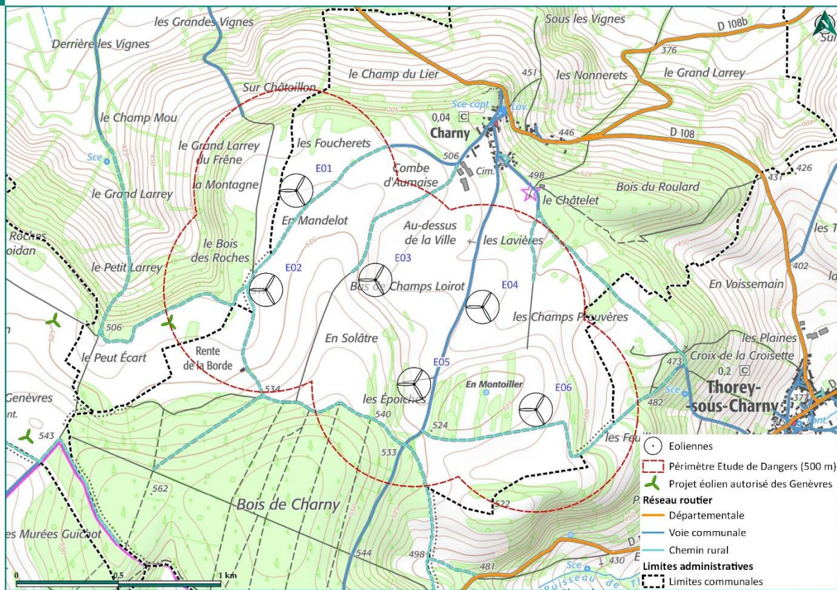
Carte 11 : Voies de communication dans le périmètre d'étude
