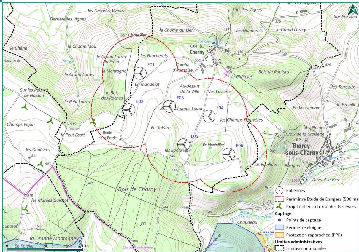
Carte 14 : Captage et périmètre de protection de Côte d'Or (Source : ARS)
