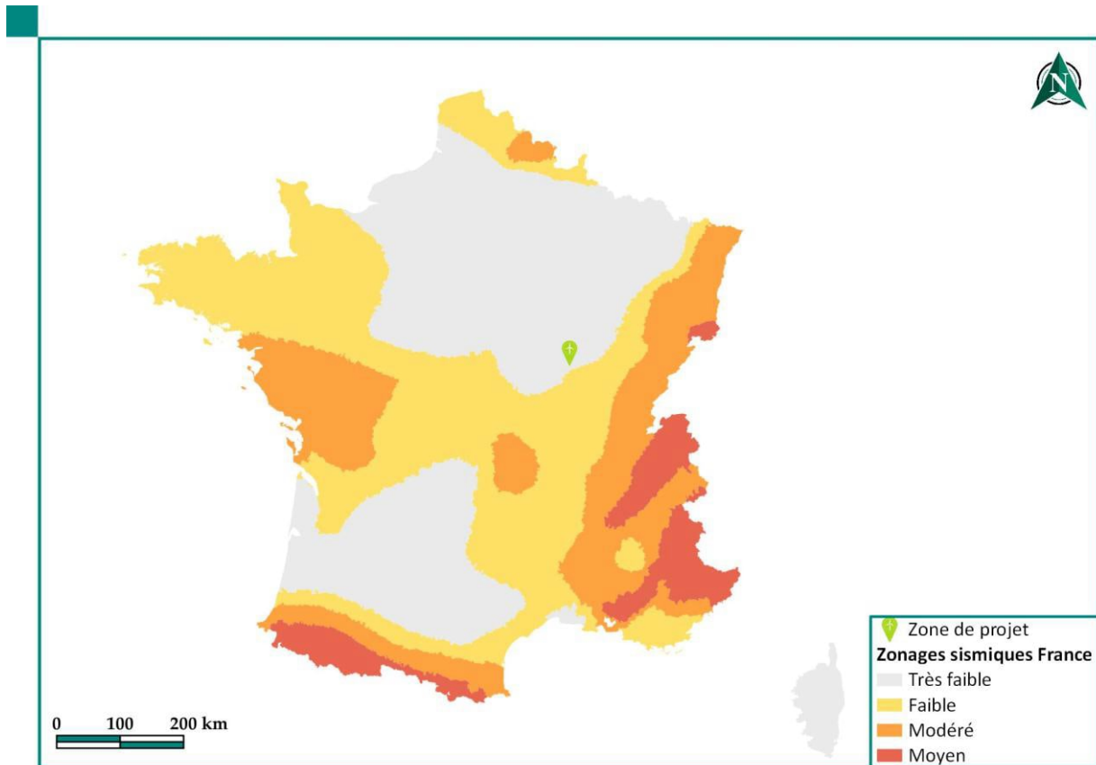
Carte 7 : Zonage sismique de France (Source : Géorisques)
