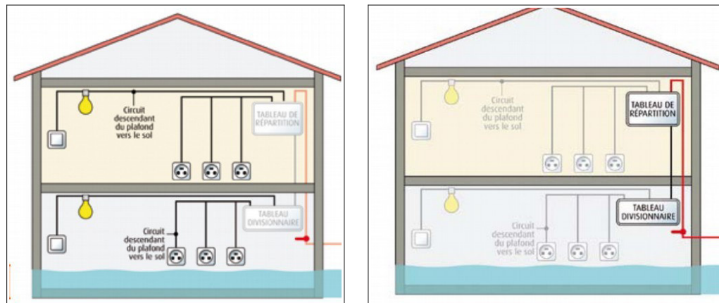
Principe de séparation des installations électriques
