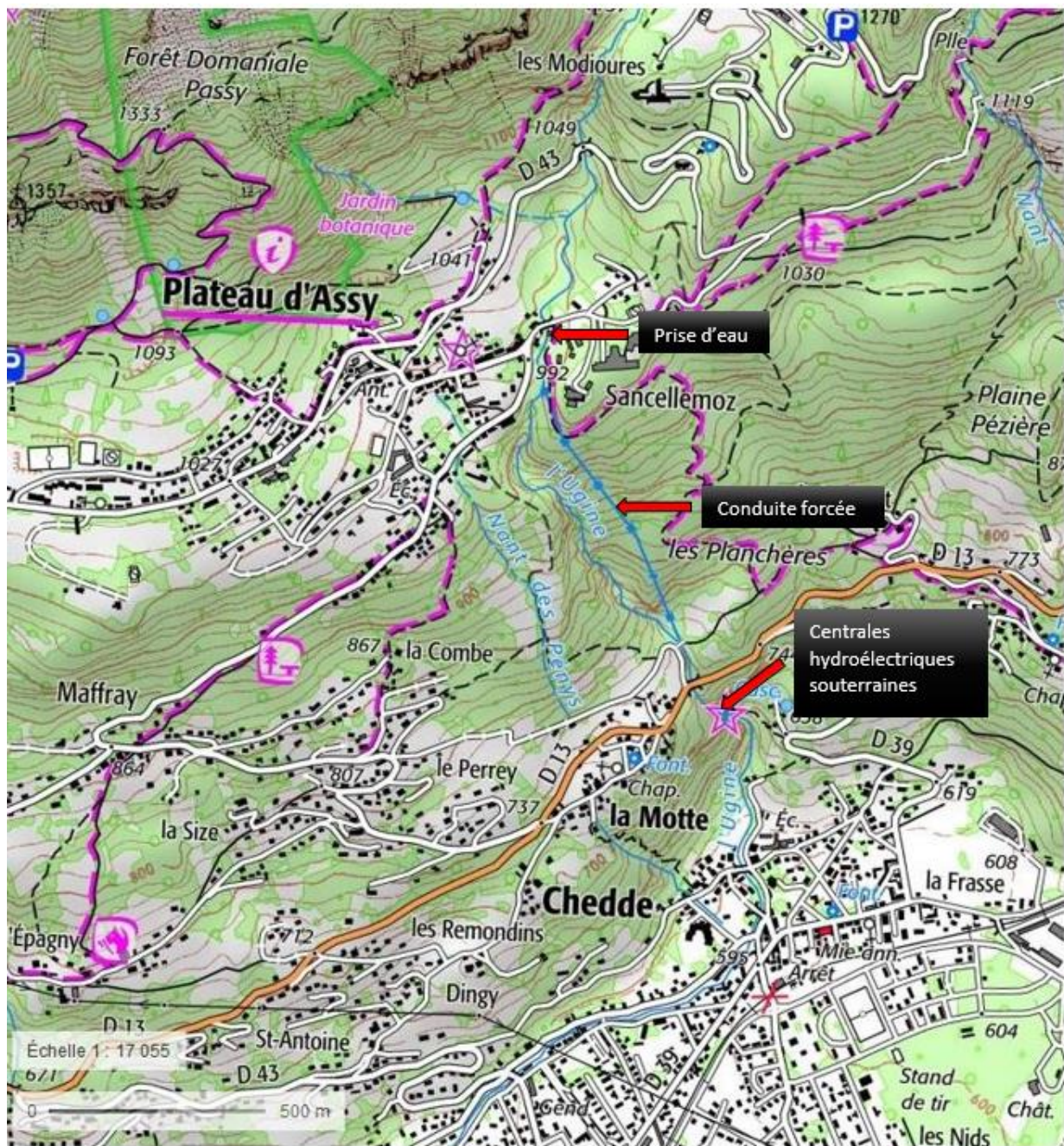
Carte 2 : L'aménagement hydroélectrique et les ouvrages associés.
