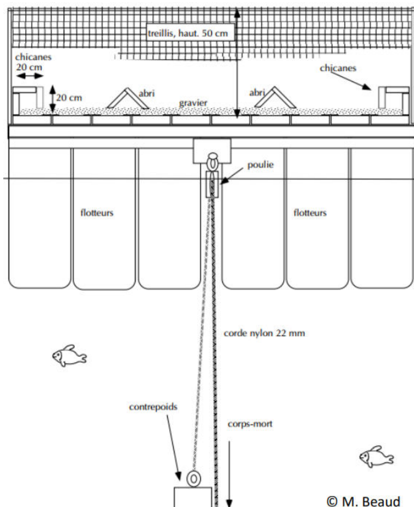
Schéma du radeau du lac de la Gruyère (Suisse)
