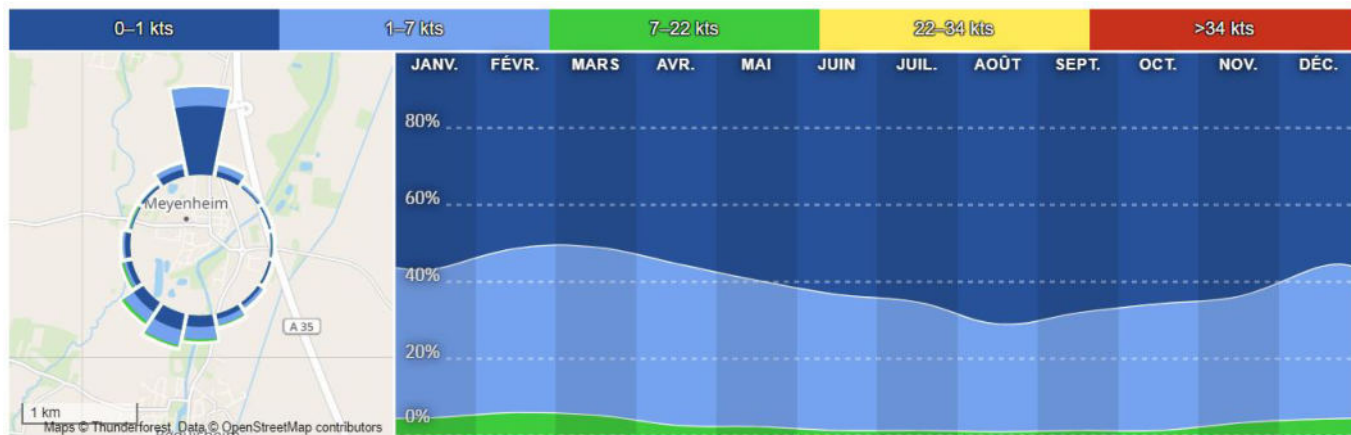
Figure 38 : Distribution annuelle de la direction du vent en % au niveau de la station météo de Meyenheim (Source : windfinder.com)
