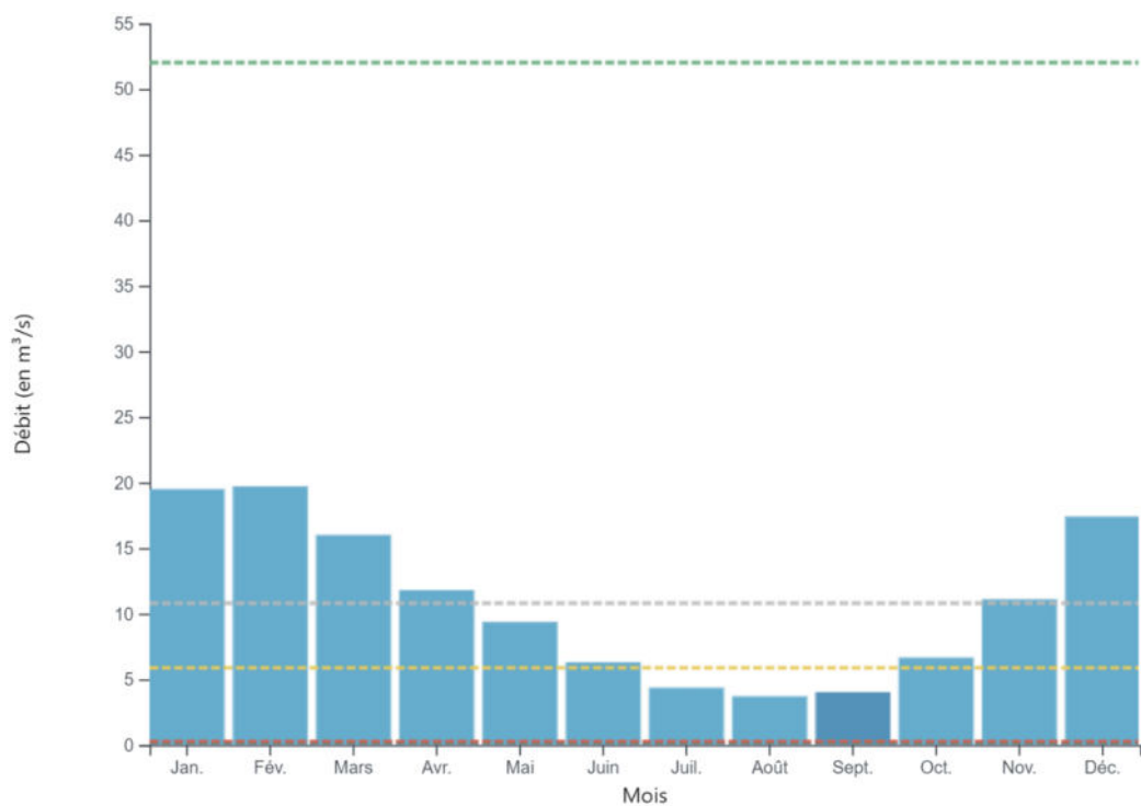
Figure 15 : Débits moyens mensuels (1957-2024) du cours d'eau l'Ill à Ensisheim
