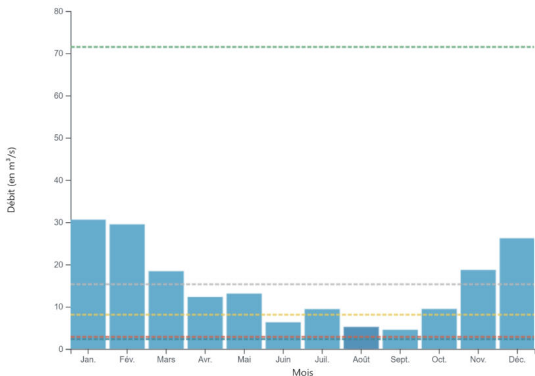
Figure 16 : Débits moyens mensuels (2019-2024) du cours d'eau l'Ill à Meyenheim
