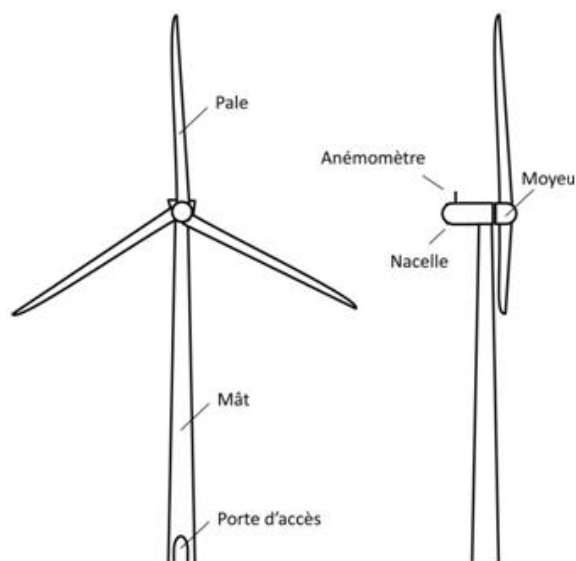
Figure 21 : Schéma simplifié d'un aérogénérateur
