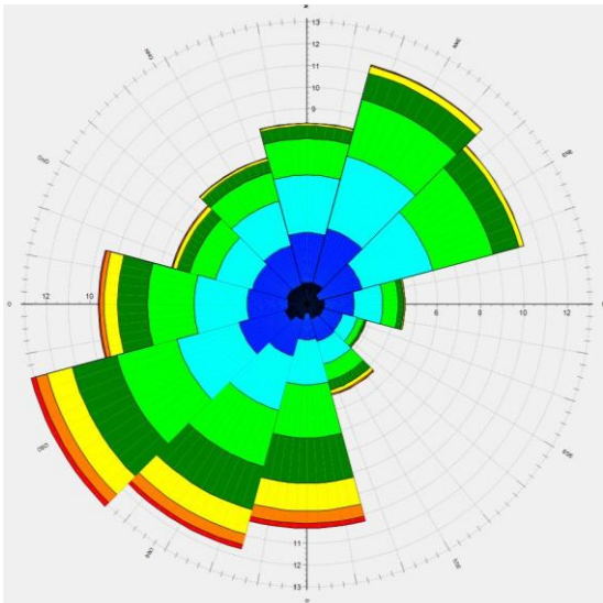
Figure 2 : Rose des vents sur le long terme (2009-2024) (Source : EOLISE)
