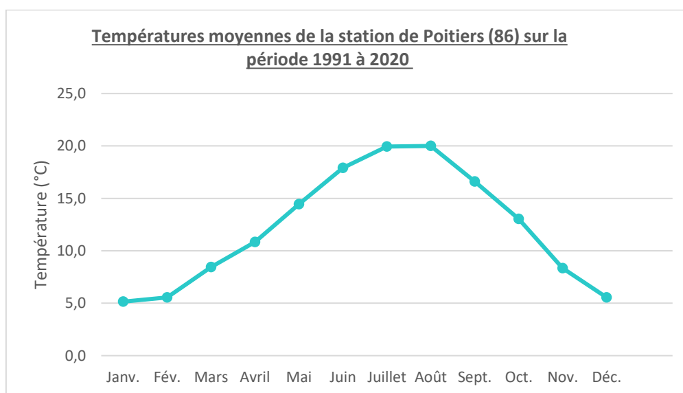
Figure 3 : Températures moyennes à Poitiers, 1991-2020. (Source : d'après Météo France)
