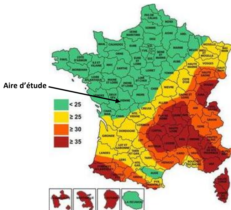
Figure 15 : Niveau céraunique en France (nombre de jours d'orage par an)
