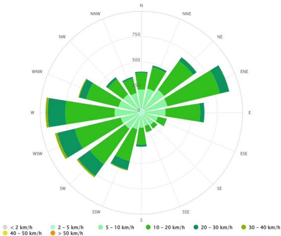
Figure 7 : Rose de vent des 30 dernières années à Poitiers (86). (Source : Meteoblue)
