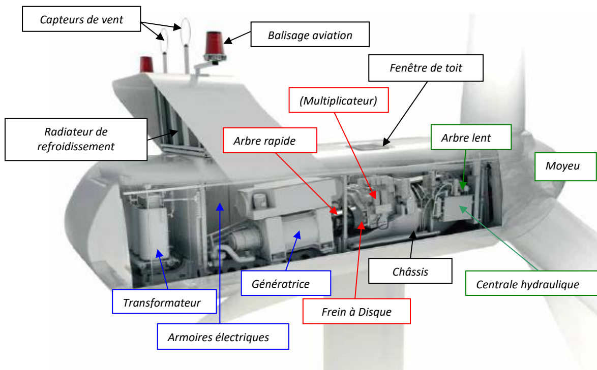
Figure 22 : Composants d'une nacelle (Source : Vestas)
