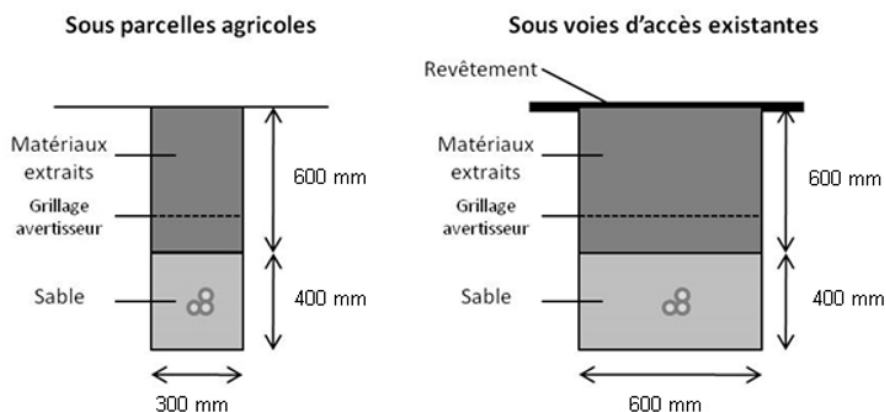
Figure 26 : Coupes générales des tranchées destinées à l'enfouissement des lignes électriques
