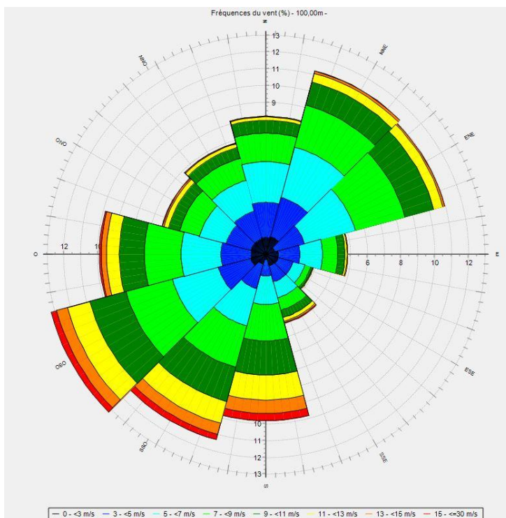
Figure 10 : Rose des vents sur le long terme (2004-2019) (Source : EOLISE)
