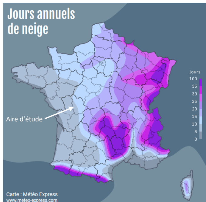
Figure 13 : Jours annuels de neige en France
