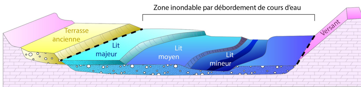
Figure 3 : Organisation de la plaine alluviale fonctionnelle
