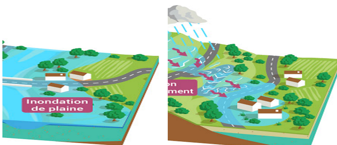
Figure 4: Types d'inondation
