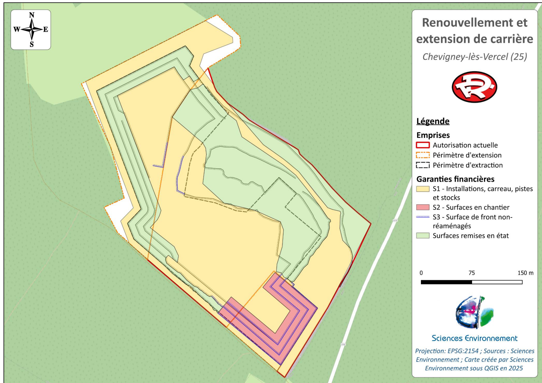
Figure 5 : Plan des garanties financières – Phase 5
