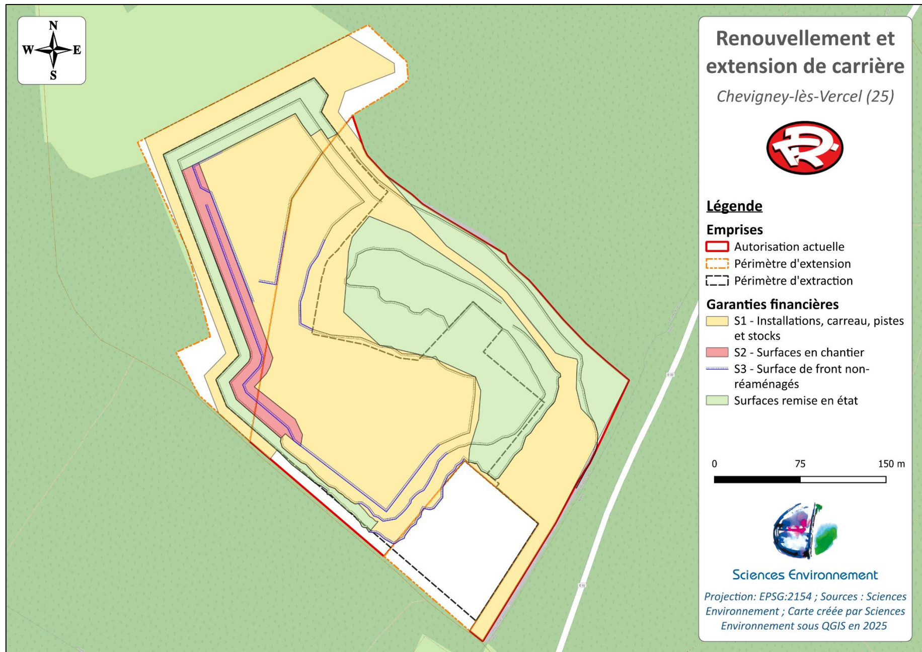
Figure 4 : Plan des garanties financières – Phase 4
