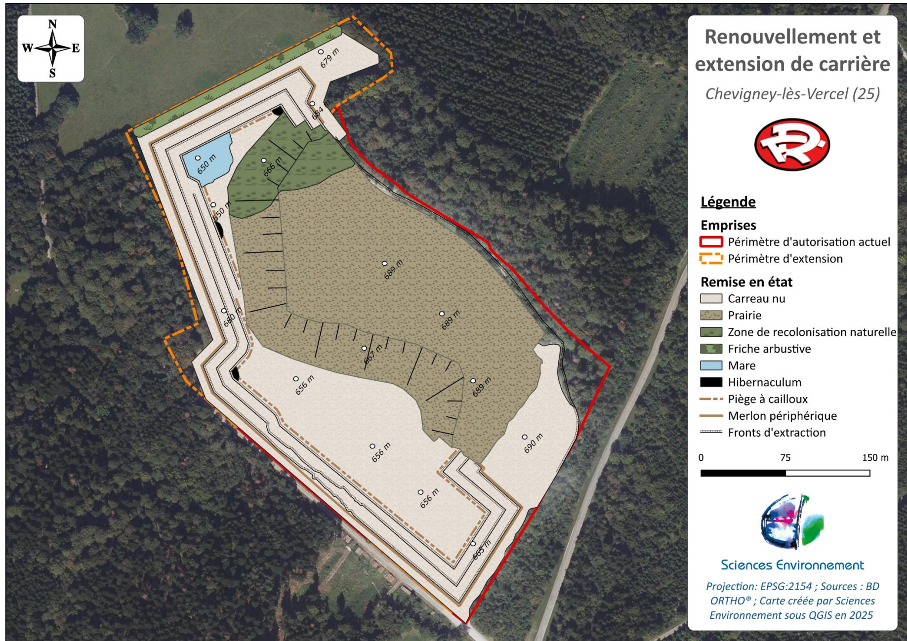
Figure 1 : Principes de remise en état de la carrière de Chevigny-lès-Vercel
