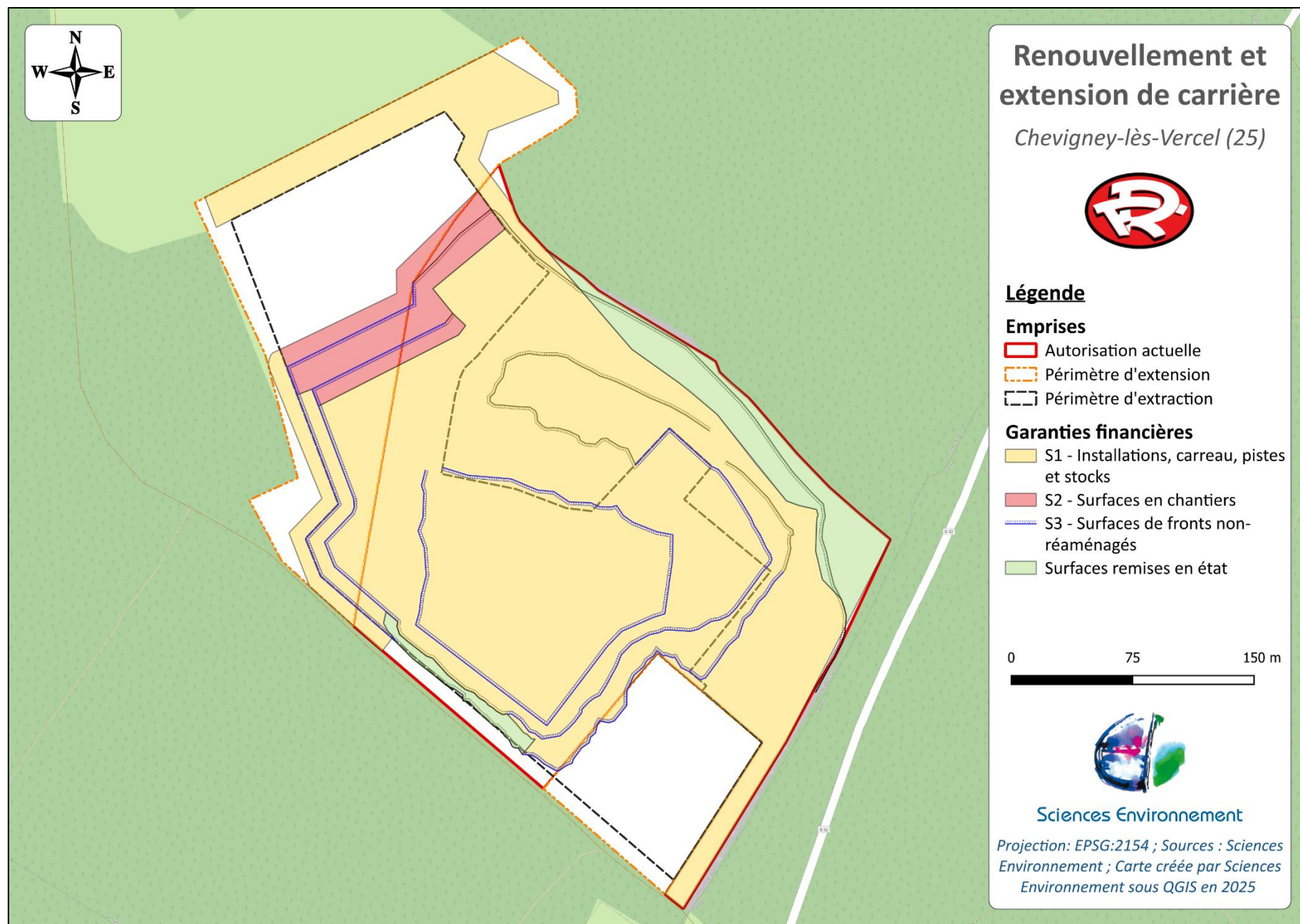
Figure 1 : Plan des garanties financières – Phase 1
